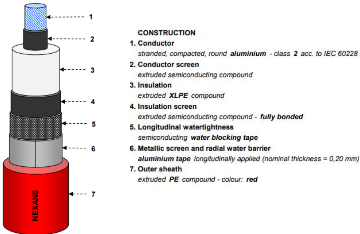
Figura 3 Configurazione tipica dei cavi unipolari previsti
