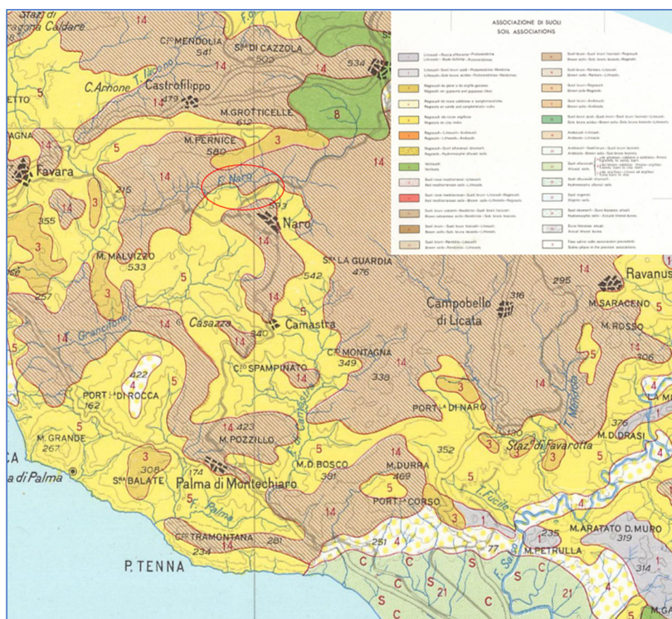
Fig.07 _ Stralcio della carta dei suoli della Sicilia
