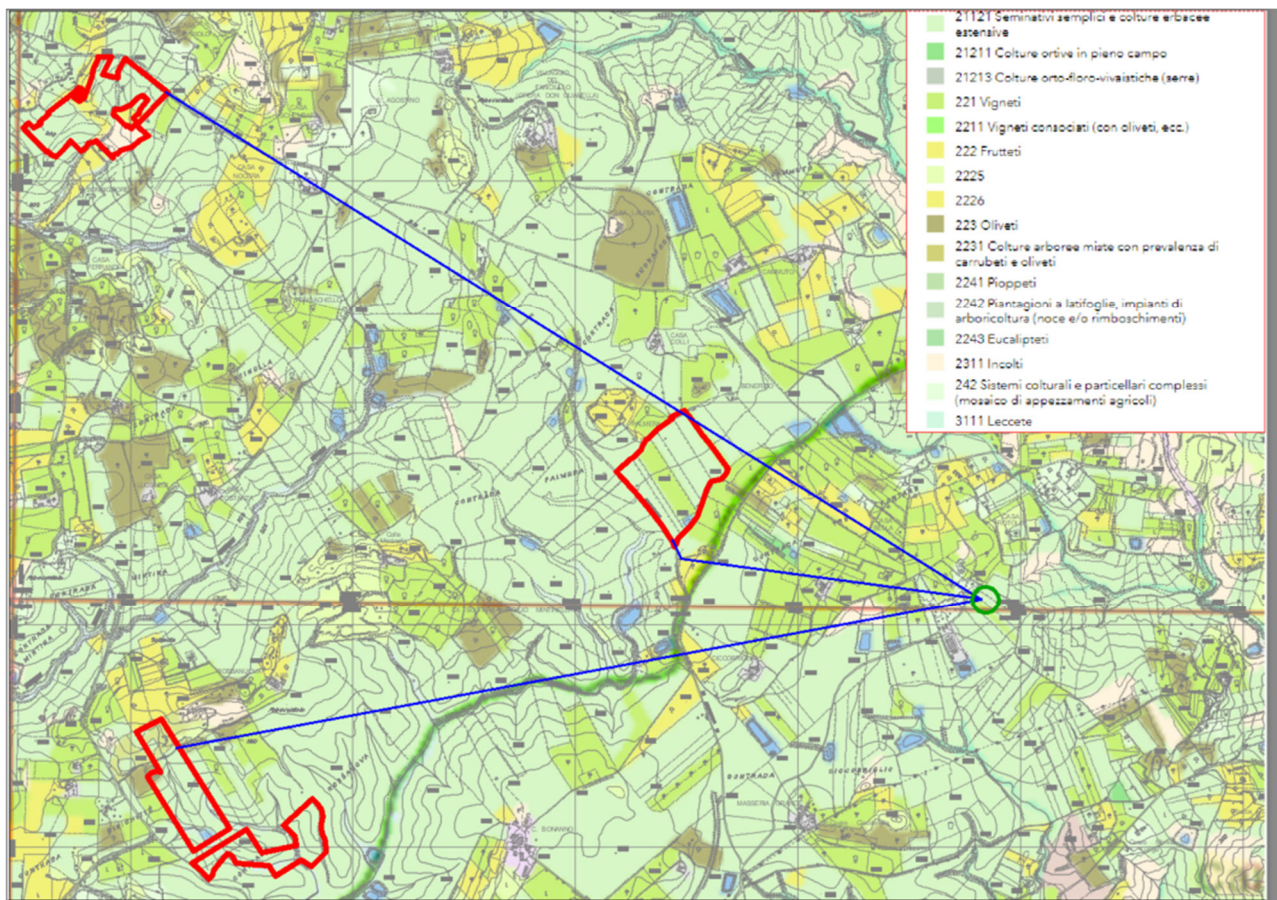
Fig.08 _ Carta dell'Uso del suolo
