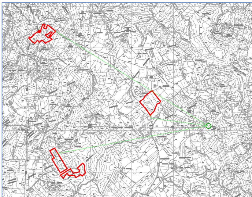
Fig. 03 _ Stralcio della CTR con ingombro dell'impianto ed il tracciato dell'elettrodotto
