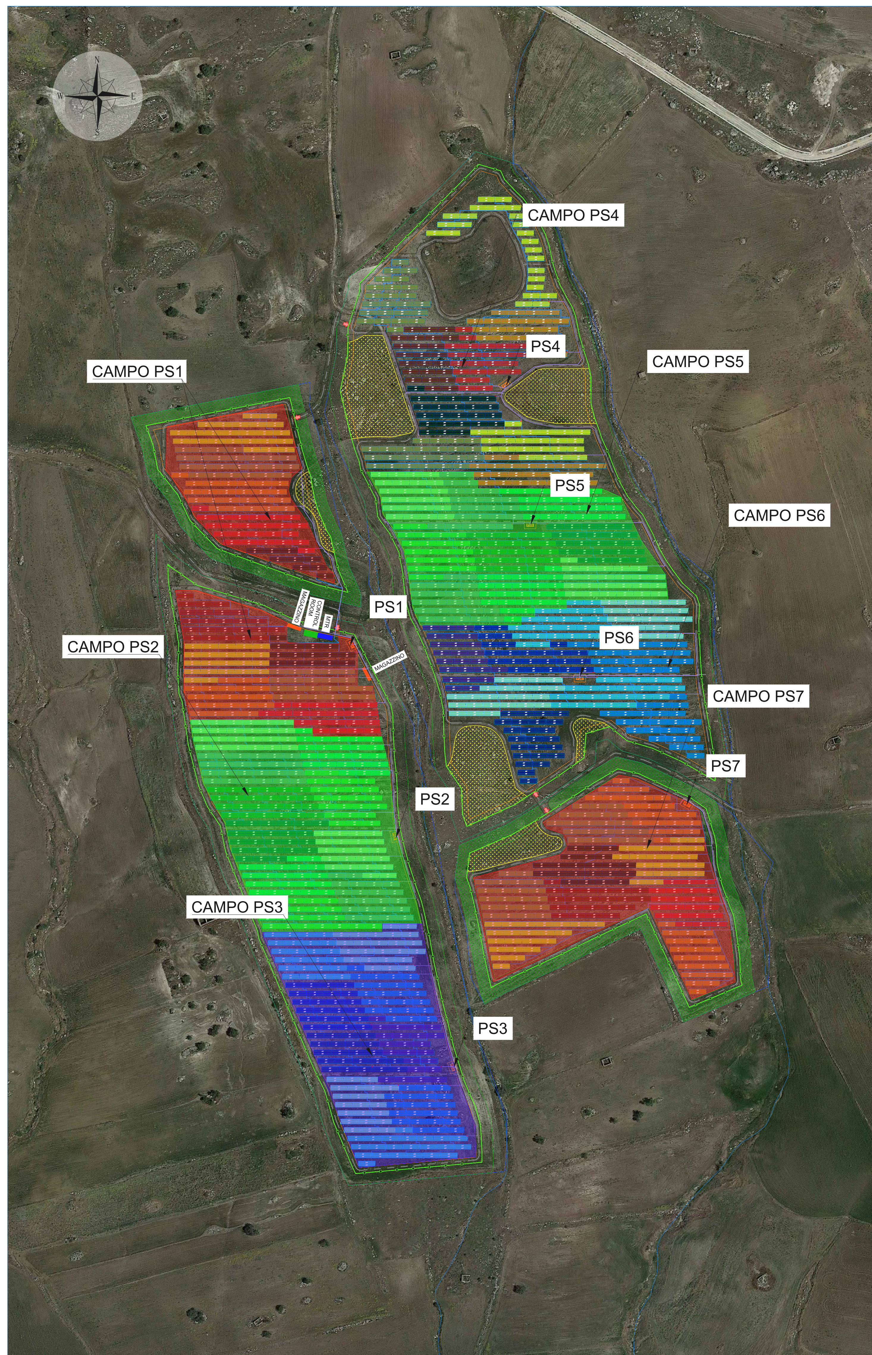
Planimetria di inquadramento: suddivisione in campi su ortofoto Scala 1:2.000
