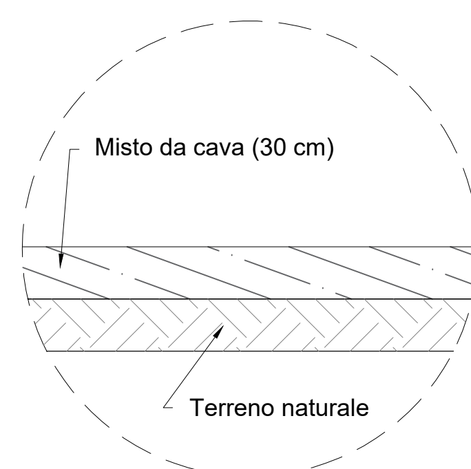
SEZIONE TIPO 4 - Aree Deposito Materiali; - Area uffici.
