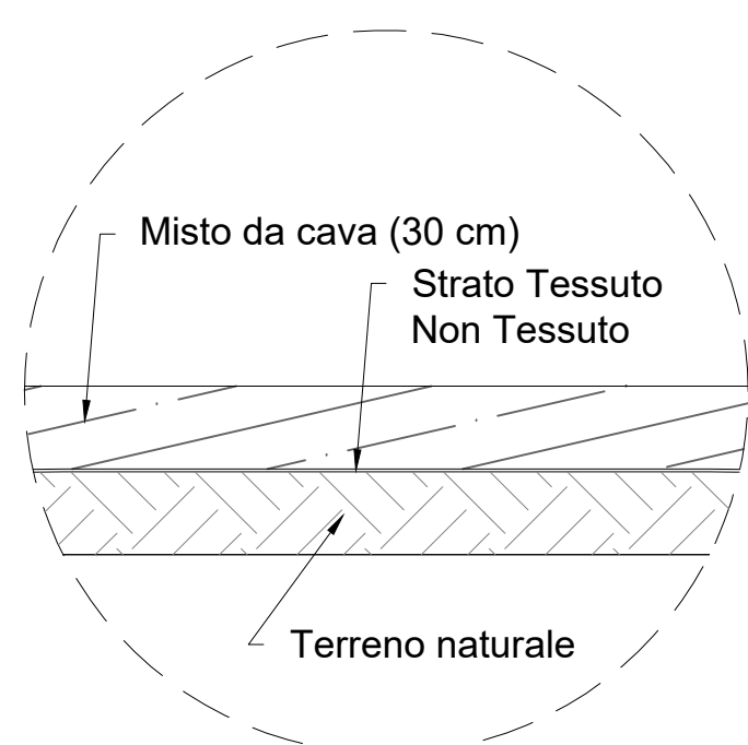
SEZIONE TIPO 3 - Area uffici e servizi
