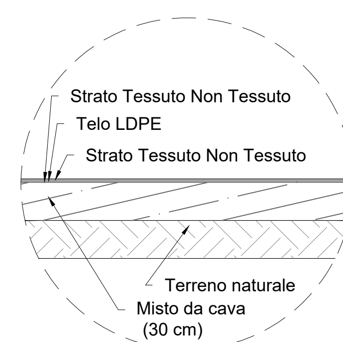
SEZIONE TIPO 5 - Area Deposito Fanghi Bentonitici.
