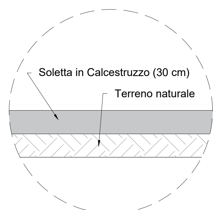
SEZIONE TIPO 2 - Area cisterna gasolio/rifornimento mezzi - Area Deposito Temporaneo Rifiuti
