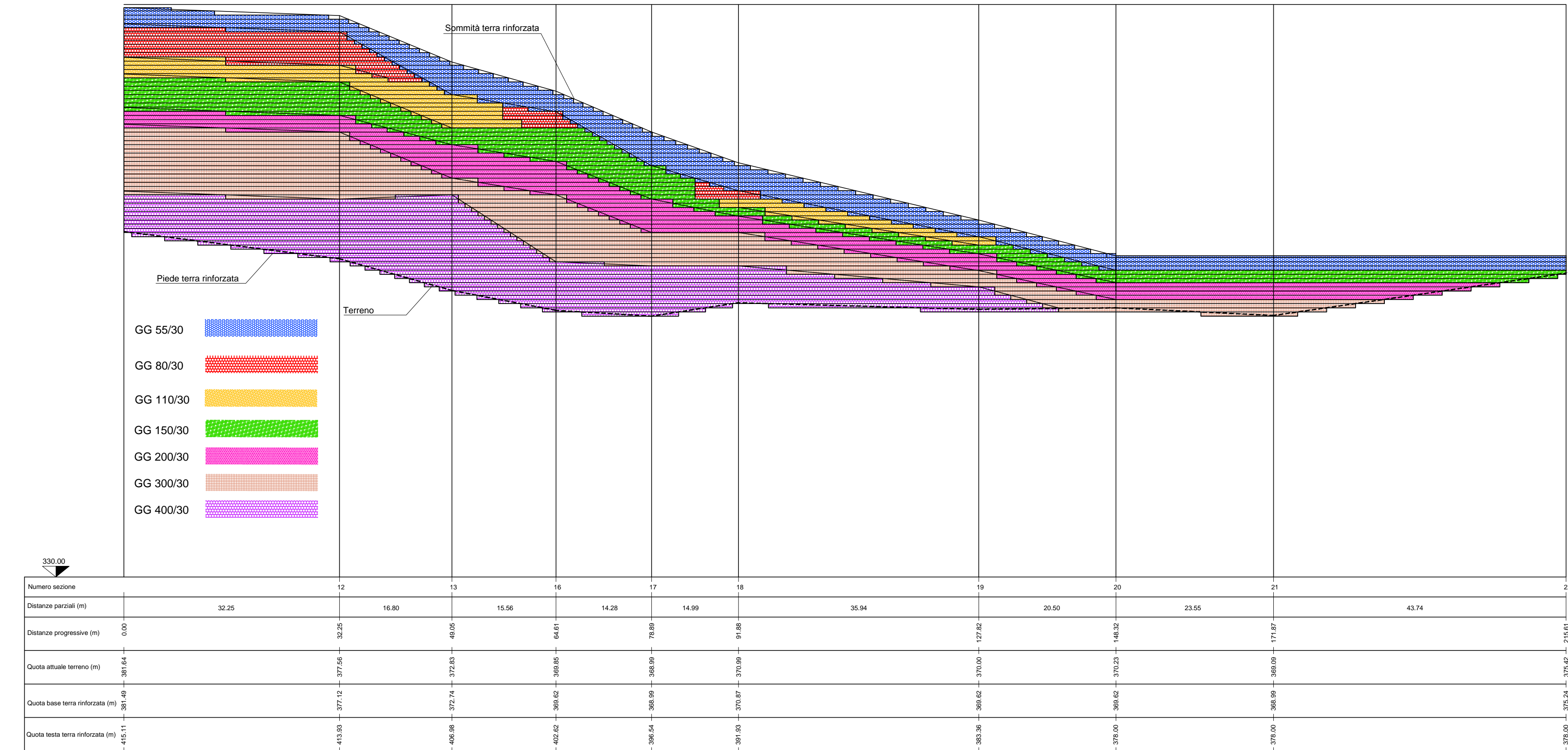
Profilo terra rinforzata lato vasca di accumulo - scala 1:500
