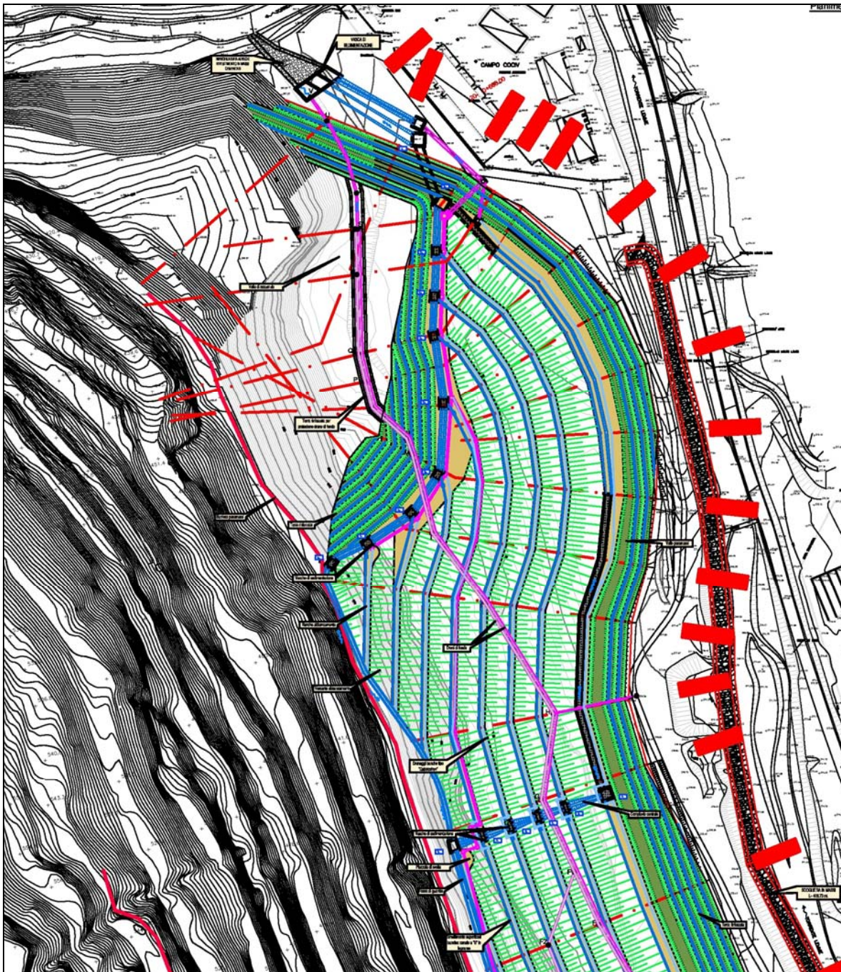
Figura 1: planimetria con ubicazione della vasca di accumulo
