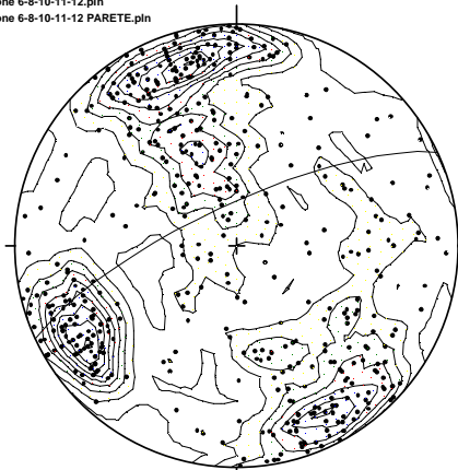
Figura 12: stereogramma delle discontinuità principali misurate nella subarea 4
