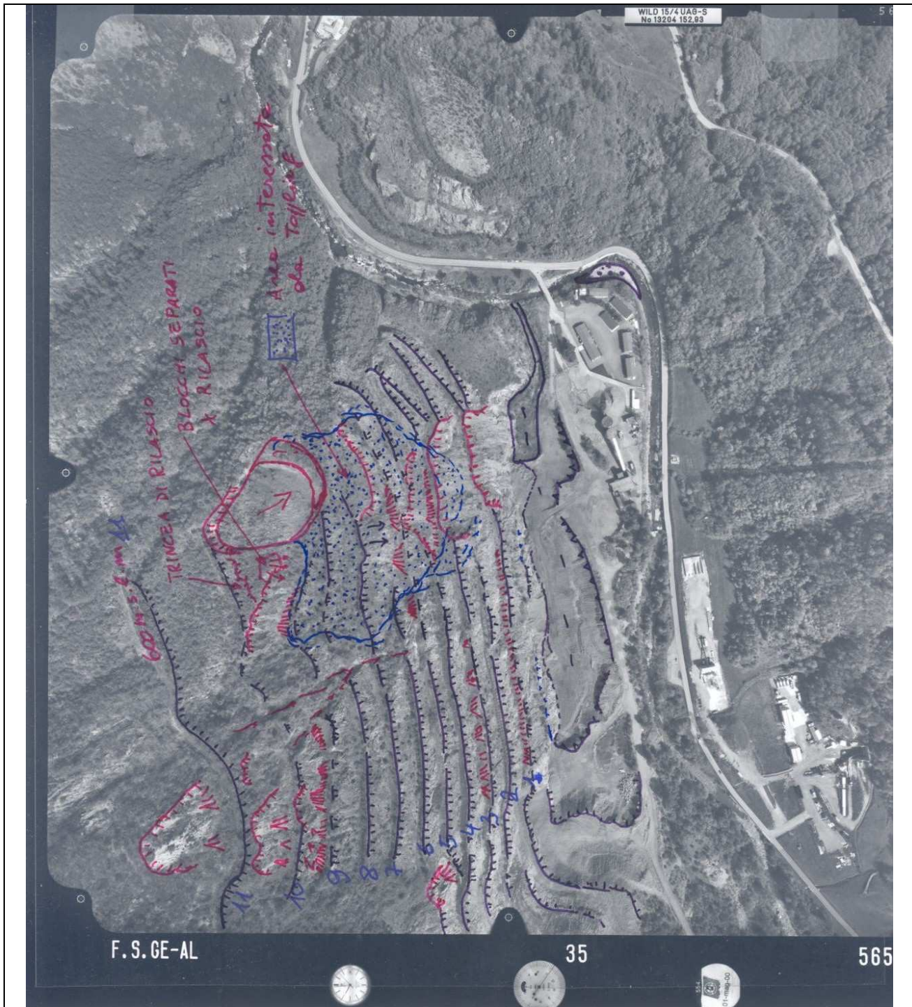
11 – Fotoaerea del 2000 ove sono evidenziate, sul margine inferiore, le banche da 1 a 11; in rosso sono evidenziate i processi erosivi che interessano il versante di coltivazione. Il puntinato azzurro evidenzia l'area interessata da ribaltamento (uncinatura) degli strati. In corrispondenza
