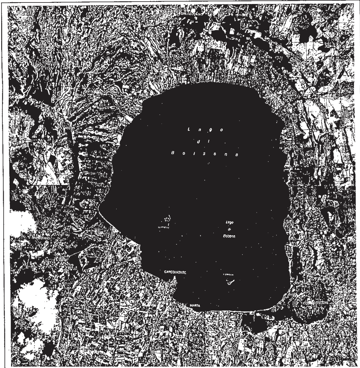
Sul versante est le fratture sono visibili, a ovest sono state coperte dalle ceneri del vulcano di Latera
