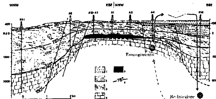
Fig. 35 - Sezione geologica schematica su una traccia prossima o in corrispondenza dei pozzi indicati. Spiegazione dei simboli: 1) Complesso vulcanico; 2) Complesso dei depositi marini pliocenici; 3) Complesso di facies ligure ed austroalpina interna; 4) Complesso di facies toscana; 5) Estensione della cappa di gas; 6) Isothermo in °C. - Schematic geologic cross section through the indicated wells. Explanation of the symbols: 1) Volcanic complex; 2) Complex of the Pliocene marine deposits; 3) Complexes of Ligurian and internal Austro-alpine facies; 4) Complex of Tuscan facies; 5) Extension of the gas cap; 6) Isotherms in °C.
