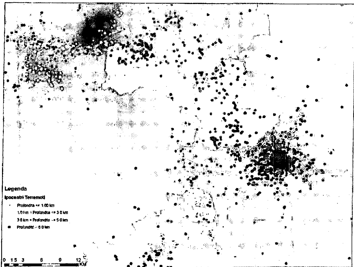
Figura 2 – Sismicità del Lazio Settentrionale – Toscana meridionale rilevata dalla rete ENEL nel periodo 1977-1992, per classi di profondità (Moia, 2008)
