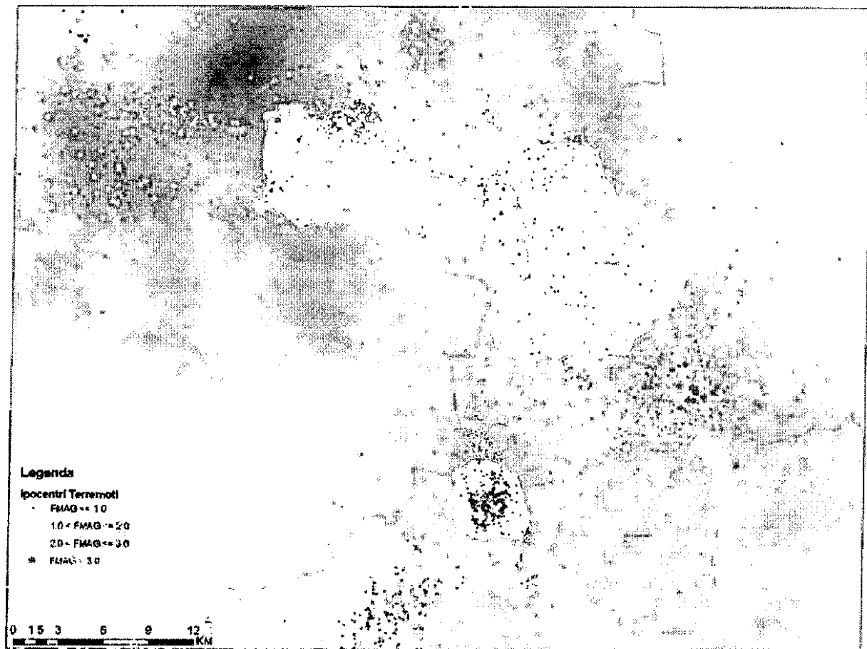
Figura 1 - Sismicità del Lazio Settentrionale - Toscana meridionale rilevata dalla rete ENEL nel periodo 1977-1992, per classi energetiche (Moia, 2008)
