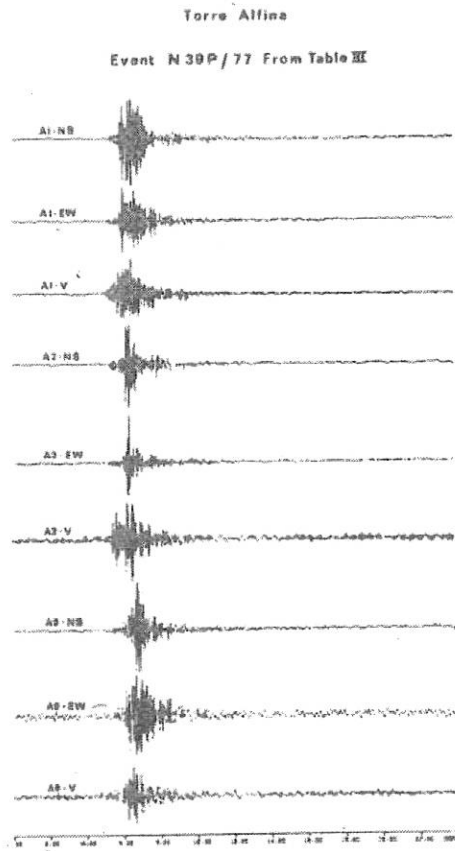
Figura 5 - Registrazione sismica di un evento occorso durante gli esperimenti di re-iniezione condotti da ENEL nel 1977 (Batini et al., 1980).
