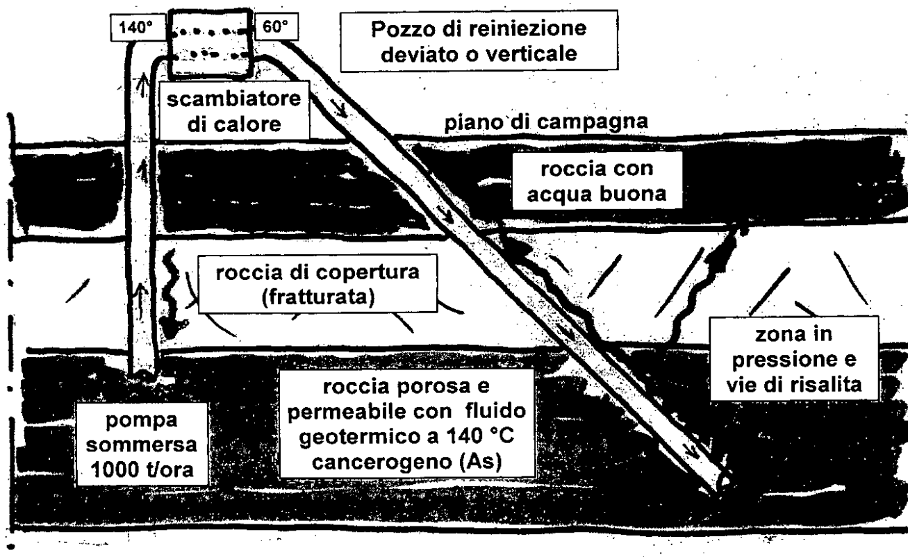
4 – SCHEMA DELL'IMPIANTO GEOTERMICO
