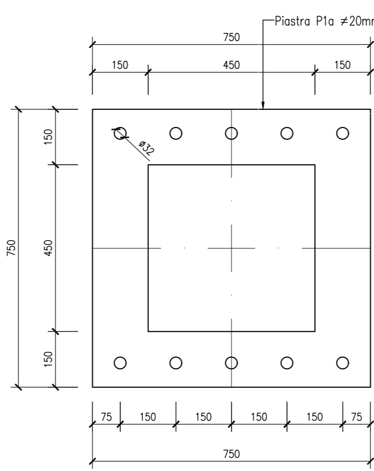
PIATTO P1a Scala 1:10
