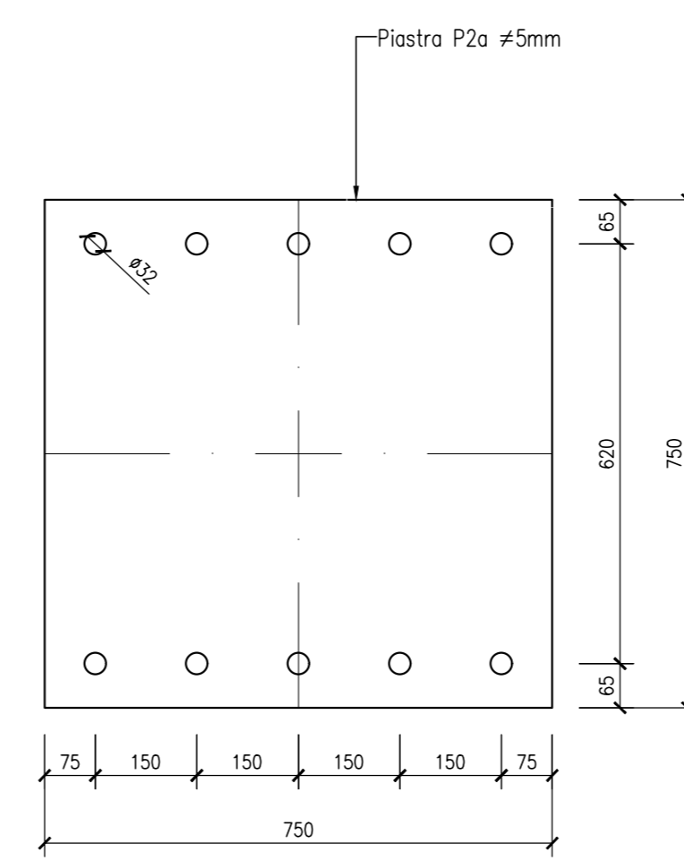
PIATTO P2a DIMA RECUPERABILE Scala 1:10
