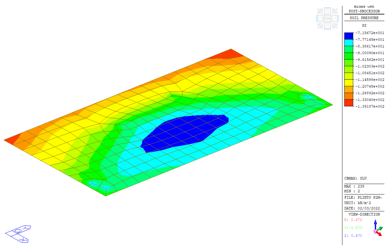
Involuppo combinazioni SLU – Massima pressione al suolo
