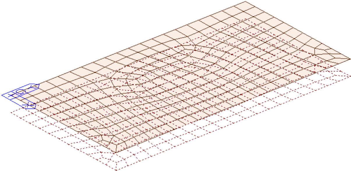
Vista modello FEM – molle lineari
