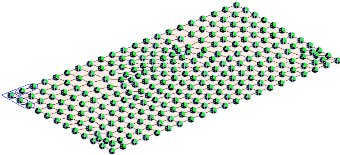
Vista modello FEM – vincoli fissi nelle direzioni orizzontali
