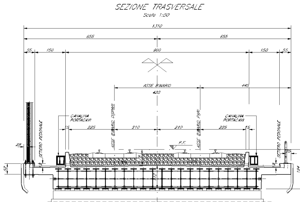
Fig. 1: Sezione trasversale dell'impalcato
