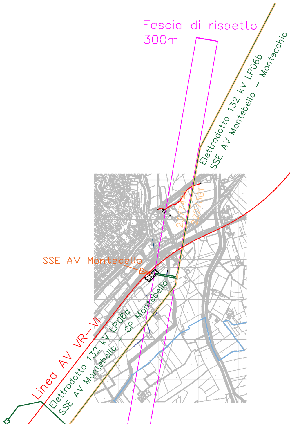
Figura 1 – Rappresentazione schematica dell'avvicinamento tra le tubazioni dell'acquedotto di Medio Chiampo nel comune di Montebello V. e elettrodotto 132kV per SSE AV Montebello (LP06a e LP06b)
