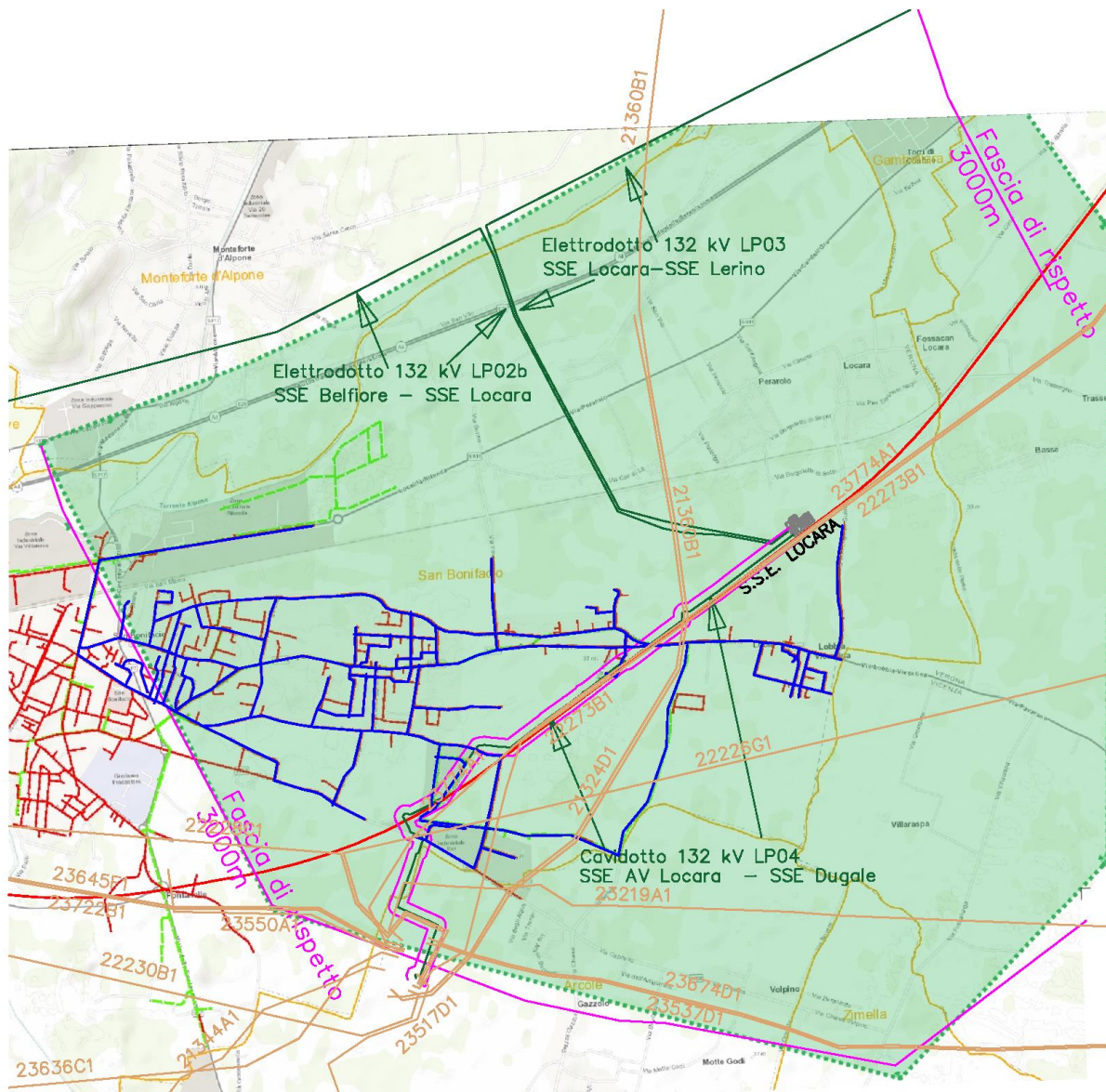
Figura 2 – Rappresentazione schematica dell'avvicinamento tra le tubazioni del metano di Erogasmet nel comune di San Bonifacio e elettrodotto 132kV per SSE Locara (LP02b e LP03) e cavidotto 132 kV per SSE Locara (LP04)
