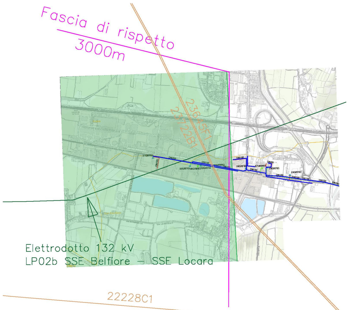
Figura 1 – Rappresentazione schematica dell'avvicinamento tra le tubazioni del metano di Erogasmet nel comune di San Bonifacio e elettrodotto 132kV per SSE Belfiore (LP02b - verso SSE Locara)
