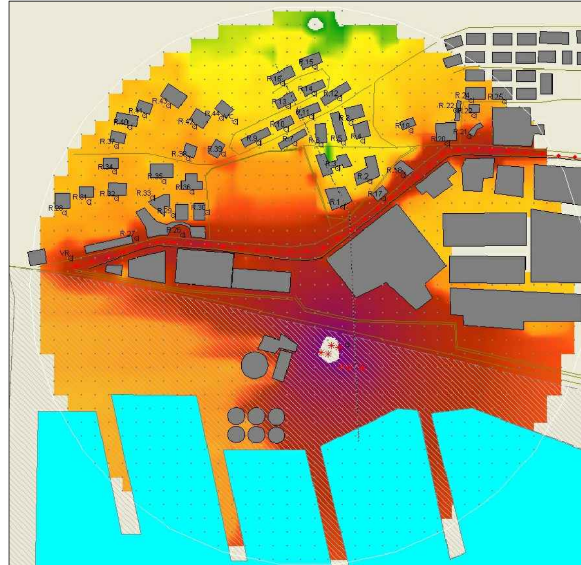
SCENARIO CANTIERE - PERIODO NOTTURNO - QUOTA DI RIFERIMENTO 4 M SENZA CONTENIMENTO ACUSTICO
