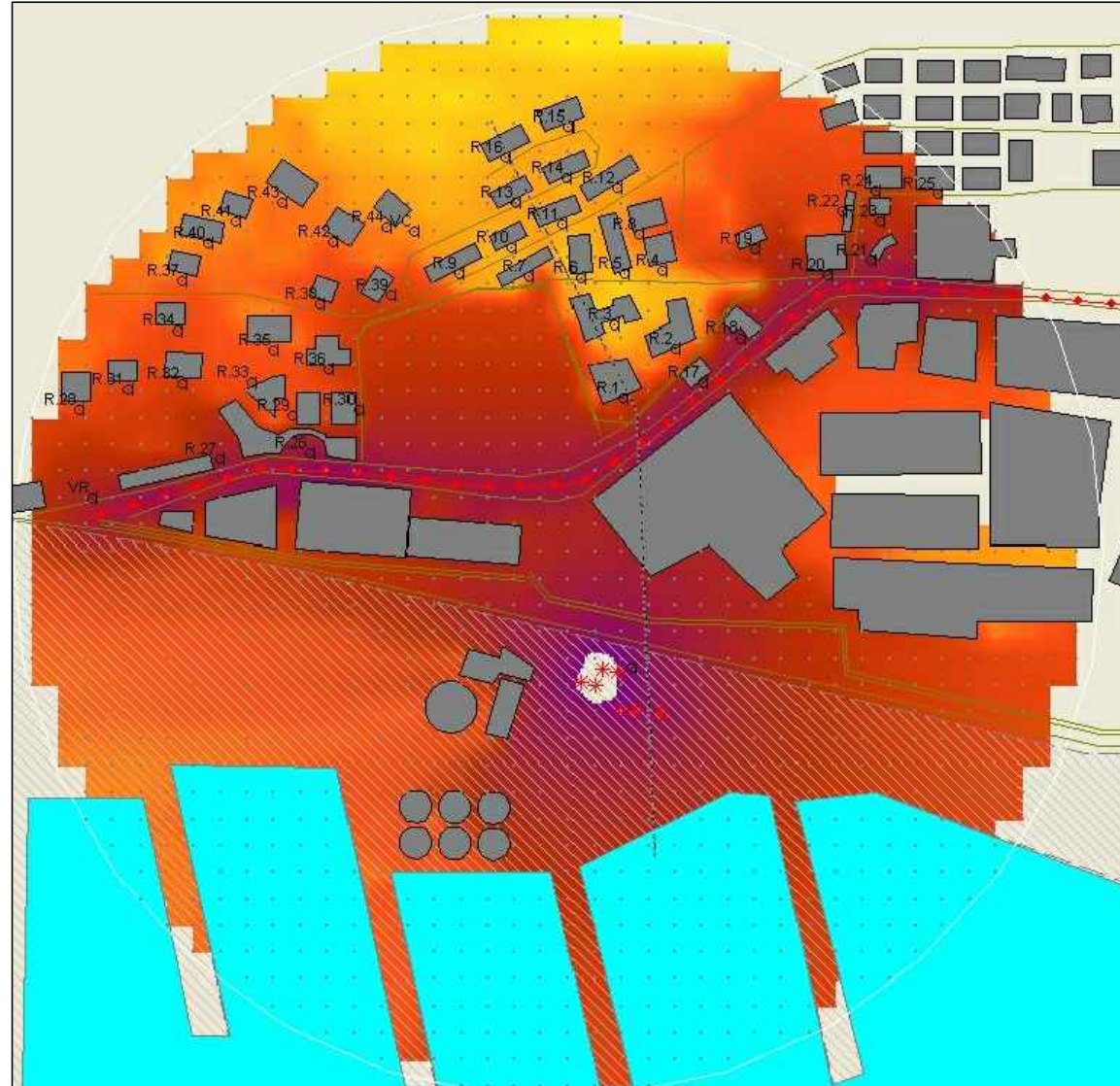
SCENARIO CANTIERE - PERIODO DIURNO - QUOTA DI RIFERIMENTO 4 M SENZA CONTENIMENTO ACUSTICO
