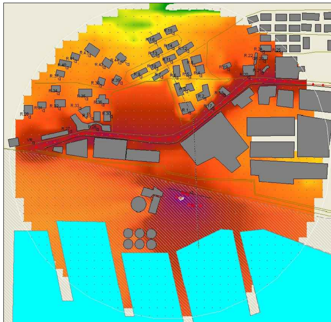
SCENARIO CANTIERE - PERIODO DIURNO - QUOTA DI RIFERIMENTO 4 M ADOZIONE BARRIERA ACUSTICA
