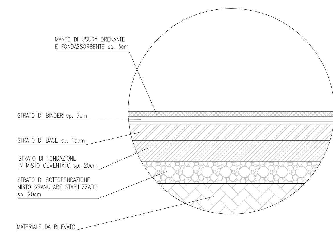
PARTICOLARE 1 1:20
