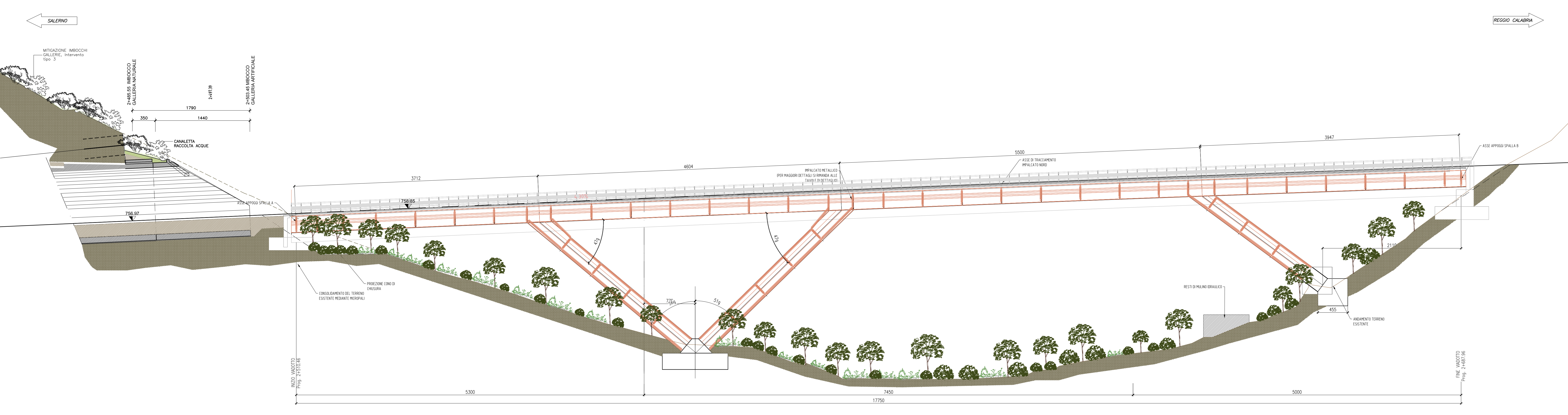
SEZIONI CARATTERISTICHE DEGLI INTERVENTI DI INSERIMENTO PAESAGGISTICI ED AMBIENTALI: Galleria Mormanno imbocco lato RC e viadotto La Pineta - Sc. 1:200
