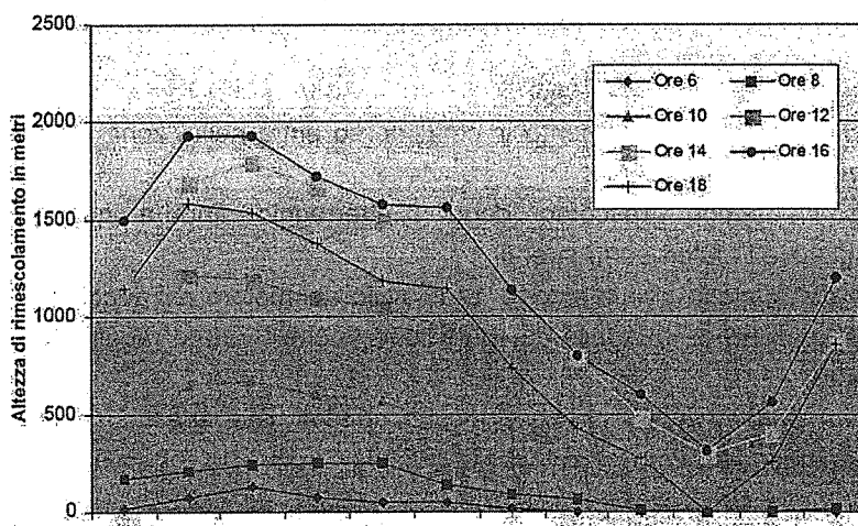
Andamento stagionale dell'altezza di rimescolamento secondo le misure dei palloni sonda a Milano Linate - Dati prof. Tebaldi - Relazione per PRQA 2000
