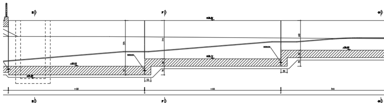
Figura 1.3: Profilo longitudinale muri di imbocco SL23
