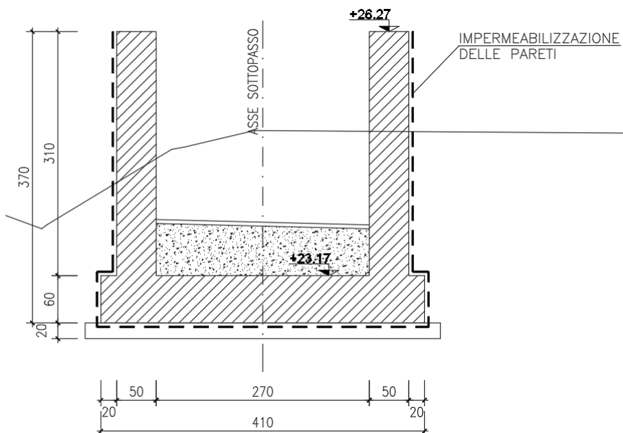
Figura 1.2: Sezione di calcolo 2 muri di imbocco SL23
