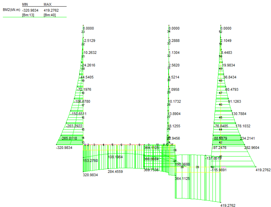
Figura 8.7: Involuppo SLU/Sisma: momenti flettenti
