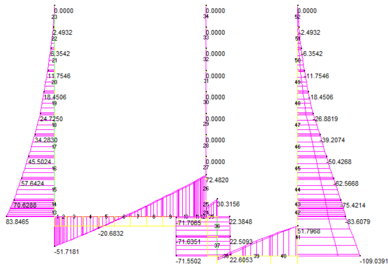
Figura 8.11: Involuppo SLE: sollecitazioni taglianti
