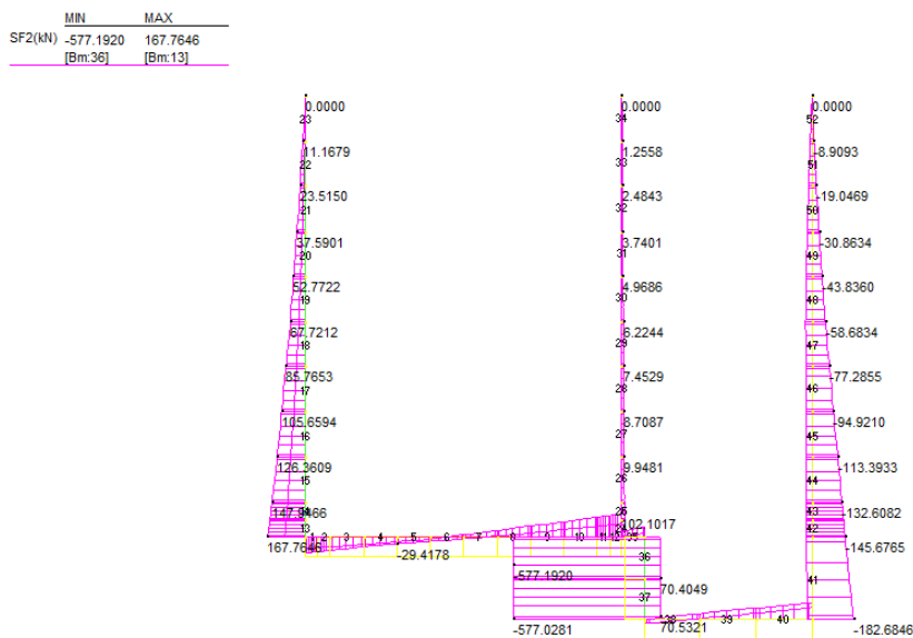
Figura 8.8: Involuppo SLU/Sisma: sollecitazioni taglianti
