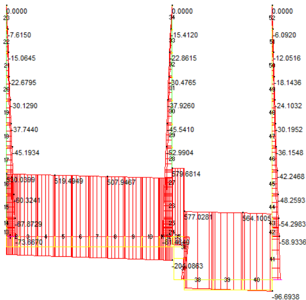
Figura 8.9: Involuppo SLU/Sisma: sforzo normale
