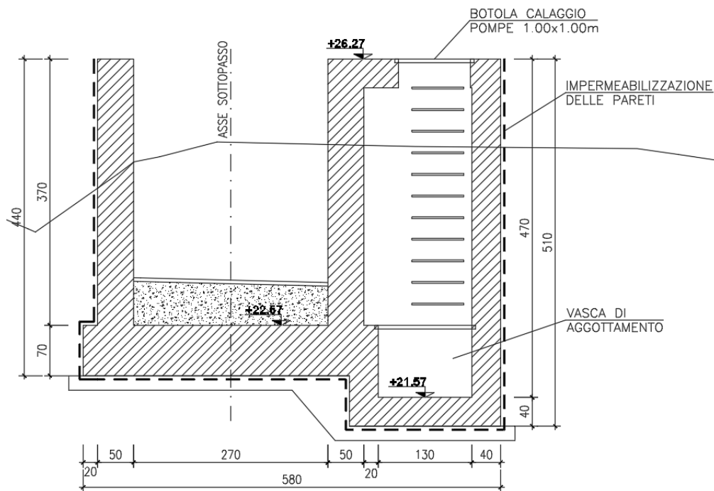
Figura 1.1: Sezione di calcolo 1 muri di imbocco SL23
