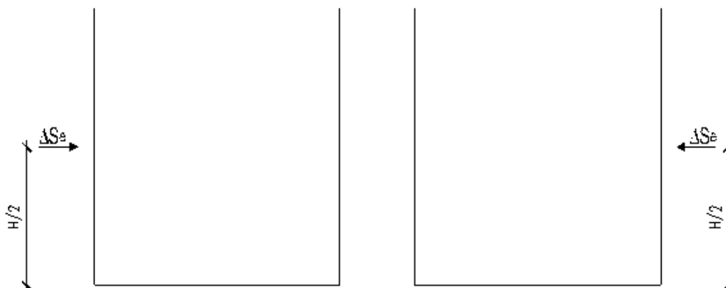
Figura 8.3: Spinta sismica del terreno secondo la teoria di Wood
