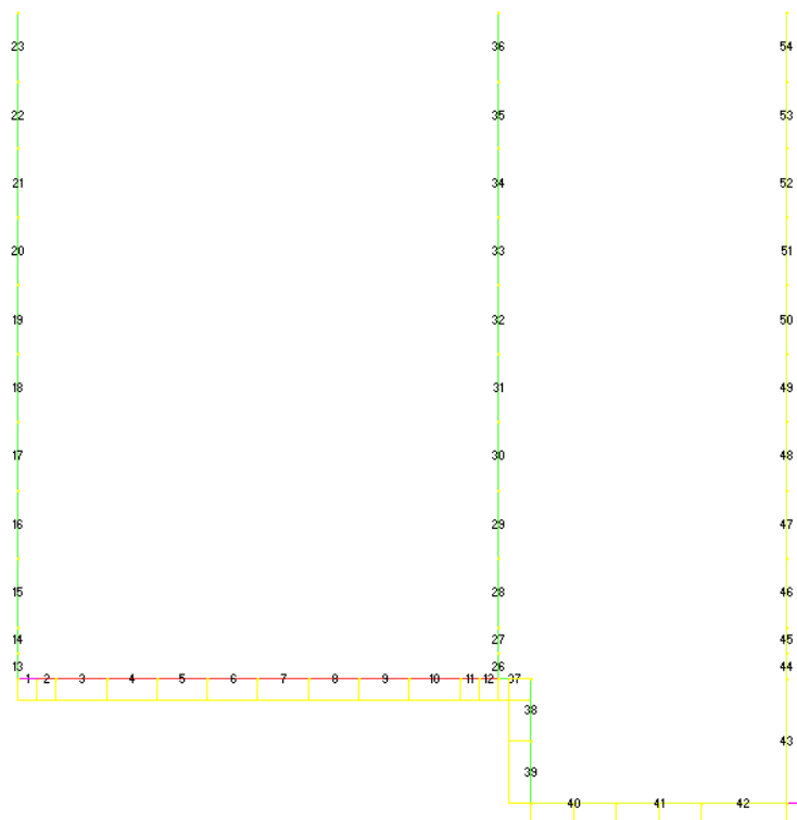
Figura 8.5: Modello F.E.M. struttura – numerazione aste
