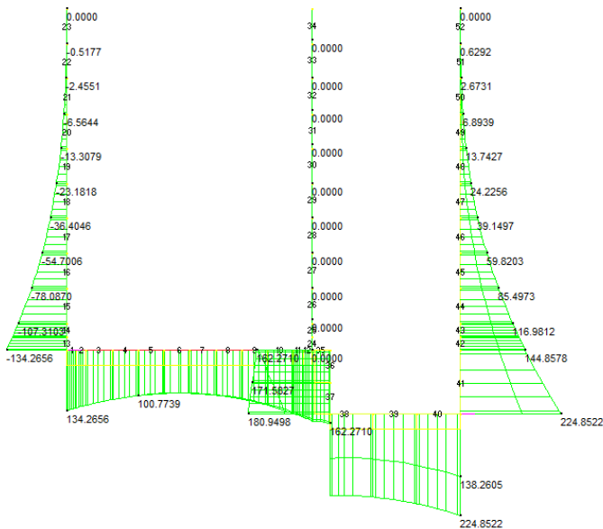
Figura 8.10: Involuppo SLE: momenti flettenti
