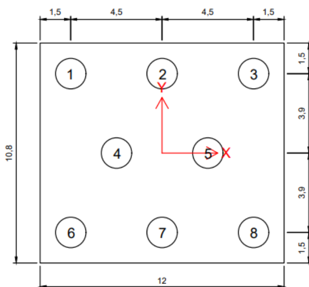
Figura 25 – Geometria del plinto di fondazione
