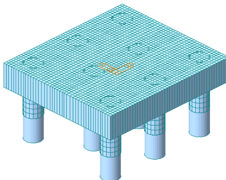
Figura 26 – Vista estrusa del modello agli elementi finiti
