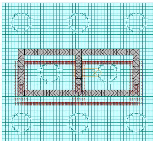
Figura 29 – Sistema di vincoli del modello agli elementi finiti
