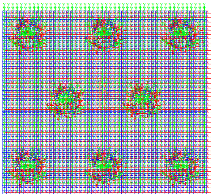
Figura 33 – Assi locali per gli elementi della platea di fondazione
