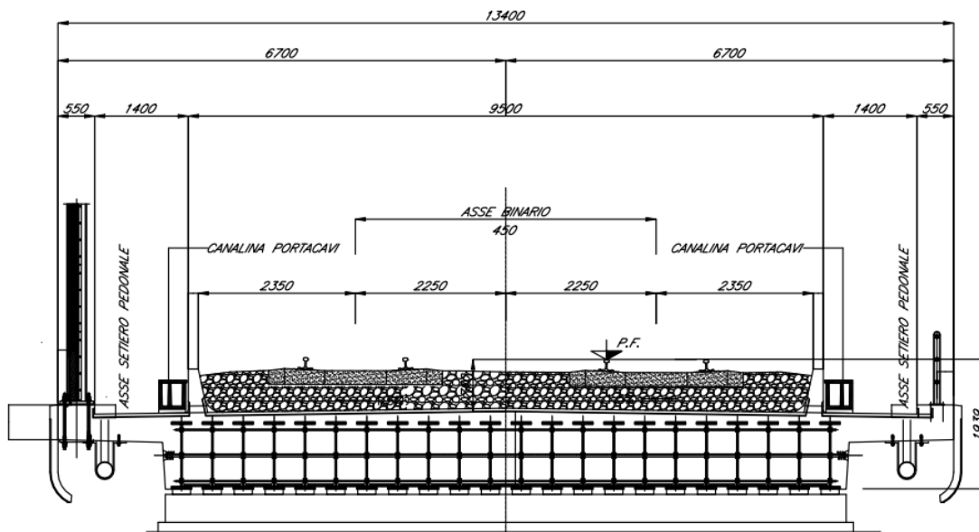
Figura 3 - Sezione impalcato travi incorporate
