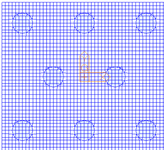
Figura 27 – Pianta del modello agli elementi finiti
