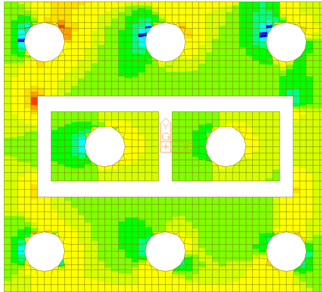
Figura 38 – Vxx, Inviluppo SLU/SLV
