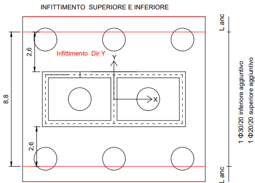
Figura 40 – Zone di infittimento dell'armatura a flessione della platea
