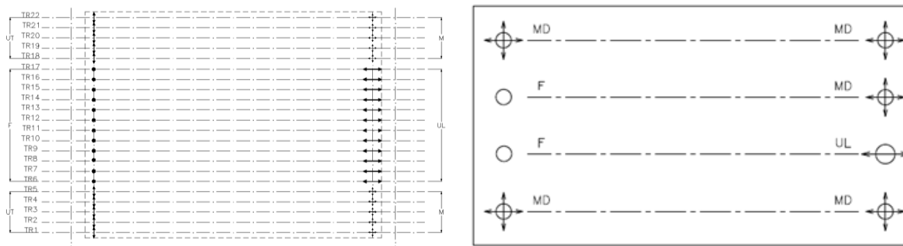
Figura 1 - Schema appoggi
