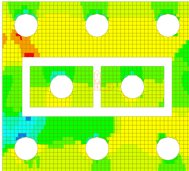
Figura 39 – Vyy, Inviluppo SLU/SLV
