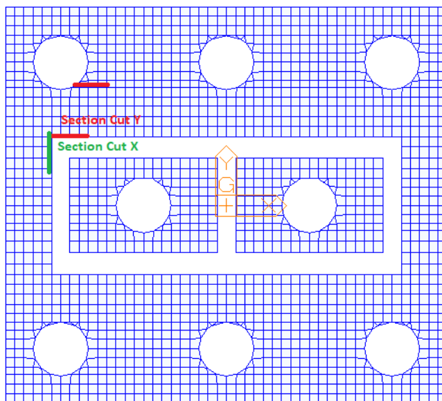
Figura 42 – Section cut considerate per la verifica a taglio
