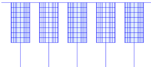
Figura 28 – Prospetto del modello agli elementi finiti
