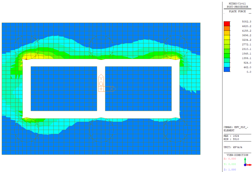
Figura 35 – Wood Armer Moment – Direction 2 – Bottom (Inviluppo SLU/SLV)
