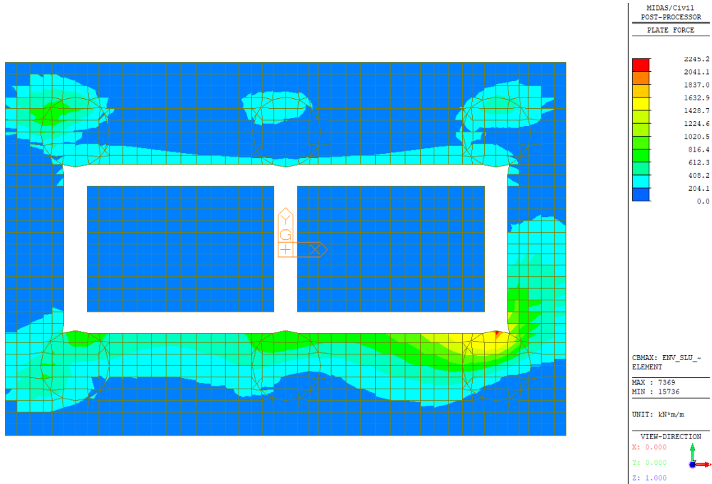
Figura 34 – Wood Armer Moment – Direction 2 – Top (Inviluppo SLU/SLV)
