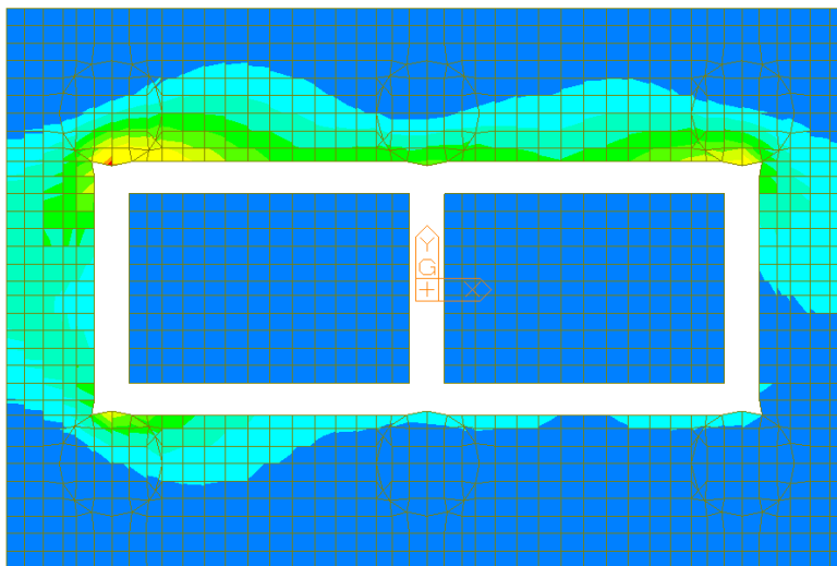
Figura 35 – Wood Armer Moment – Direction 2 – Bottom (Inviluppo SLU/SLV)
