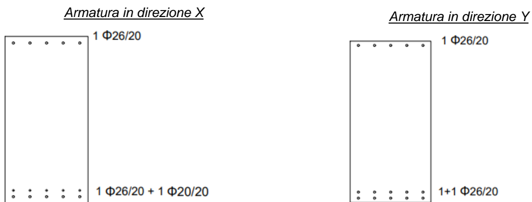
Figura 38 – Armatura a flessione del plinto
