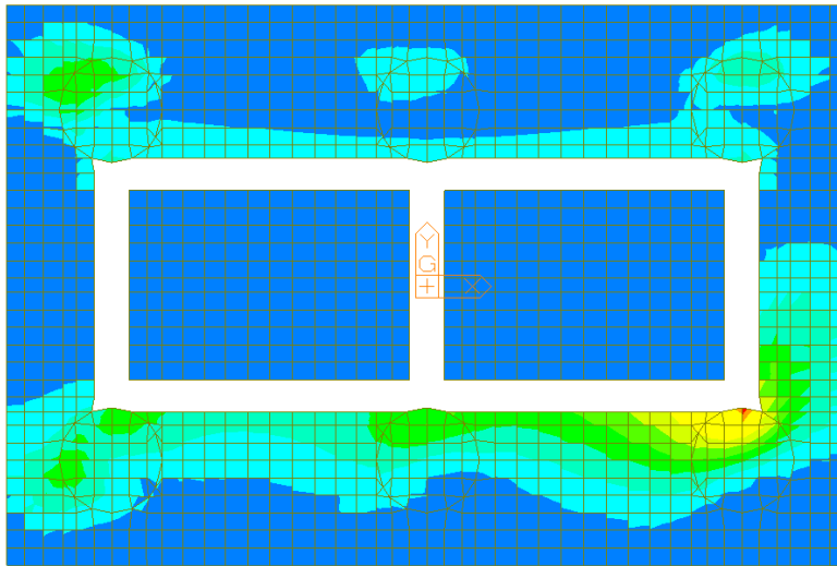
Figura 34 – Wood Armer Moment – Direction 2 – Top (Inviluppo SLU/SLV)
