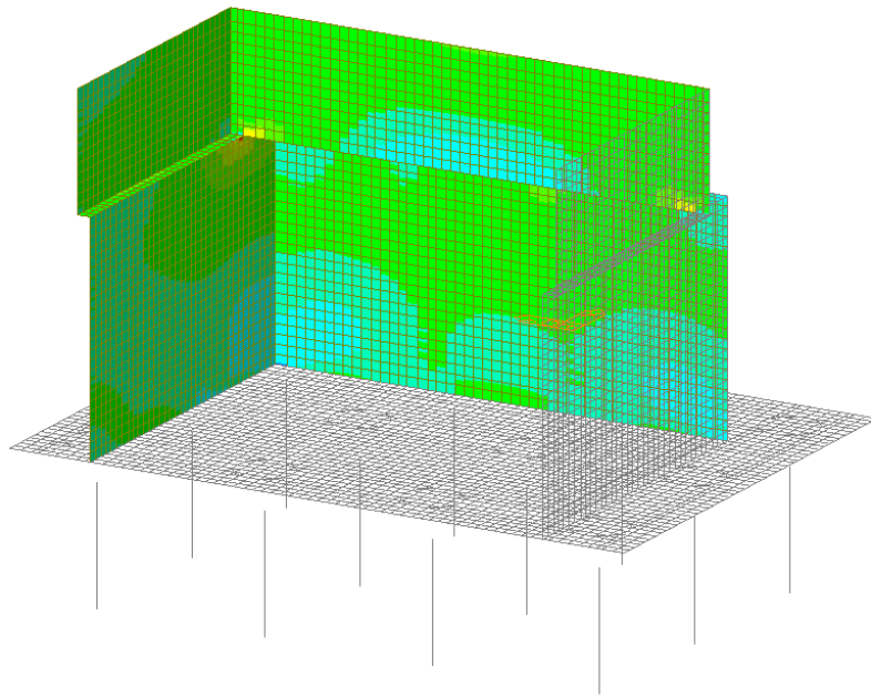
Figura 34 – Involuppo SLE Rara - Fxx
