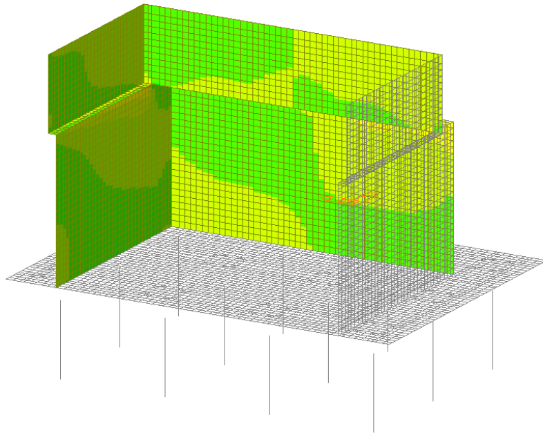
Figura 37 – Involuppo SLE Rara - Vxx
