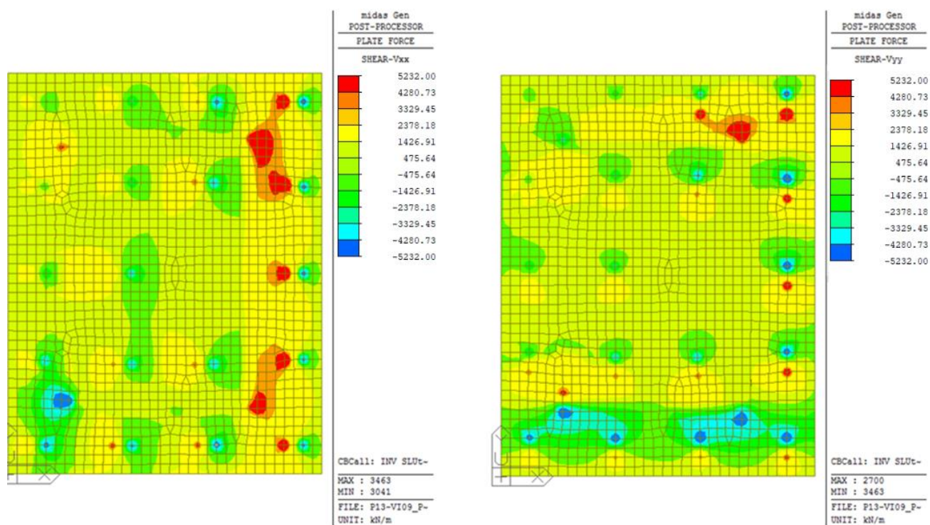
Figura 18: Involuppo delle combinazioni SLU statiche/sismiche – Taglio longitudinale (a sinistra) e trasversale (a destra)
