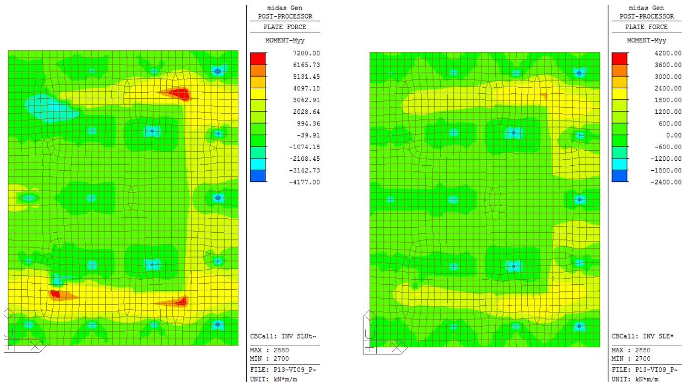
Figura 17: Momento flettente trasversale - Involuppo delle combinazioni SLU statiche/sismiche (a sinistra) e SLE (a destra)
