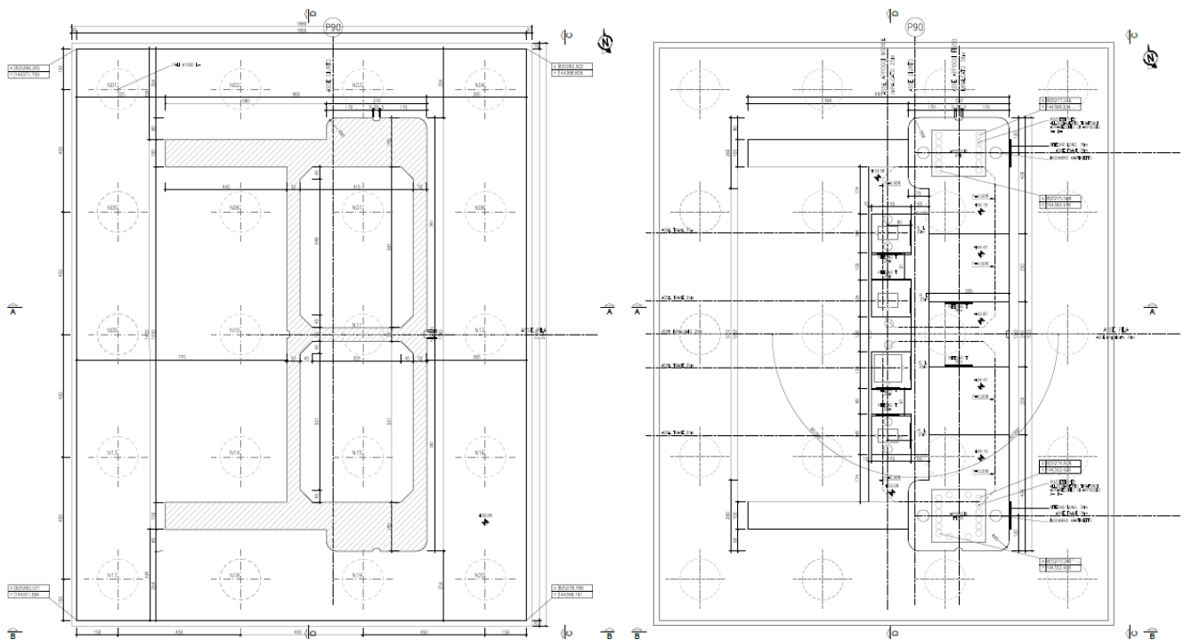
Figura 3: Pianta fondazioni (a sinistra) e pianta pulvino (a destra)
