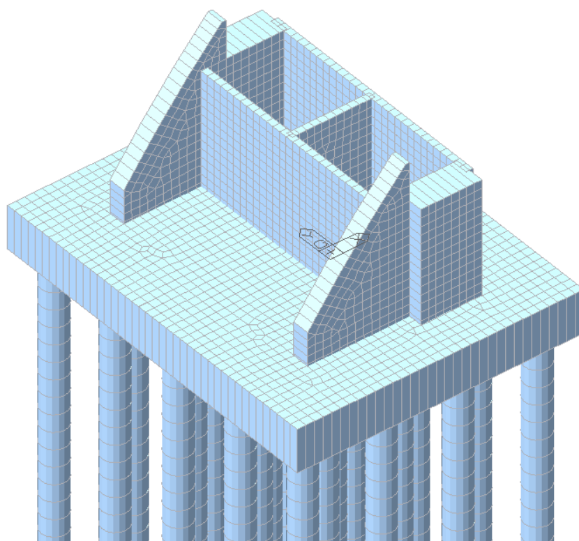
Figura 13: Modellazione tridimensionale agli Elementi Finiti – a) Vista 3D b) Spaccato
