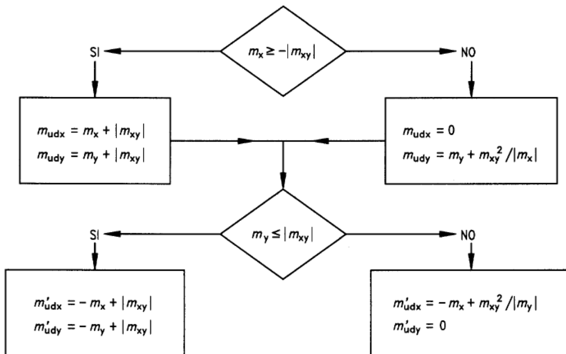
Figura 15: Diagramma di flusso per il calcolo dei momenti ultimi
