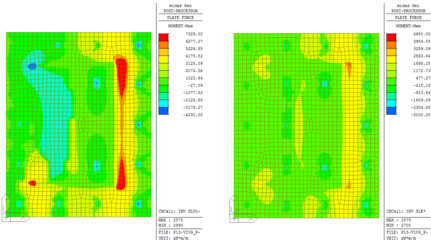
Figura 16: Momento flettente longitudinale - Inviluppo delle combinazioni SLU statiche/sismiche (a sinistra) e SLE (a destra)
