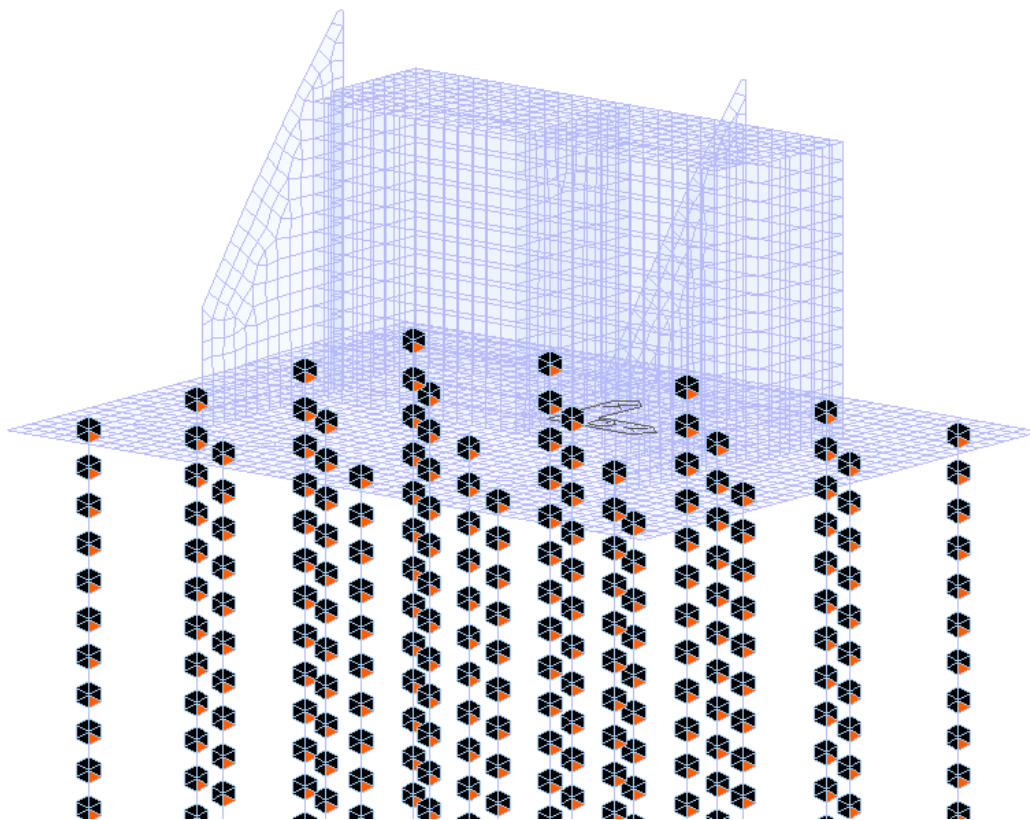
Figura 14: Modellazione tridimensionale agli Elementi Finiti – Vista wireframe – Sistema di vincolo
