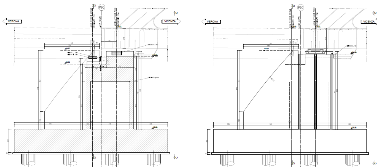
Figura 1: Sezione (a sinistra) e prospetto (a destra) longitudinali rispetto all’asse del viadotto
