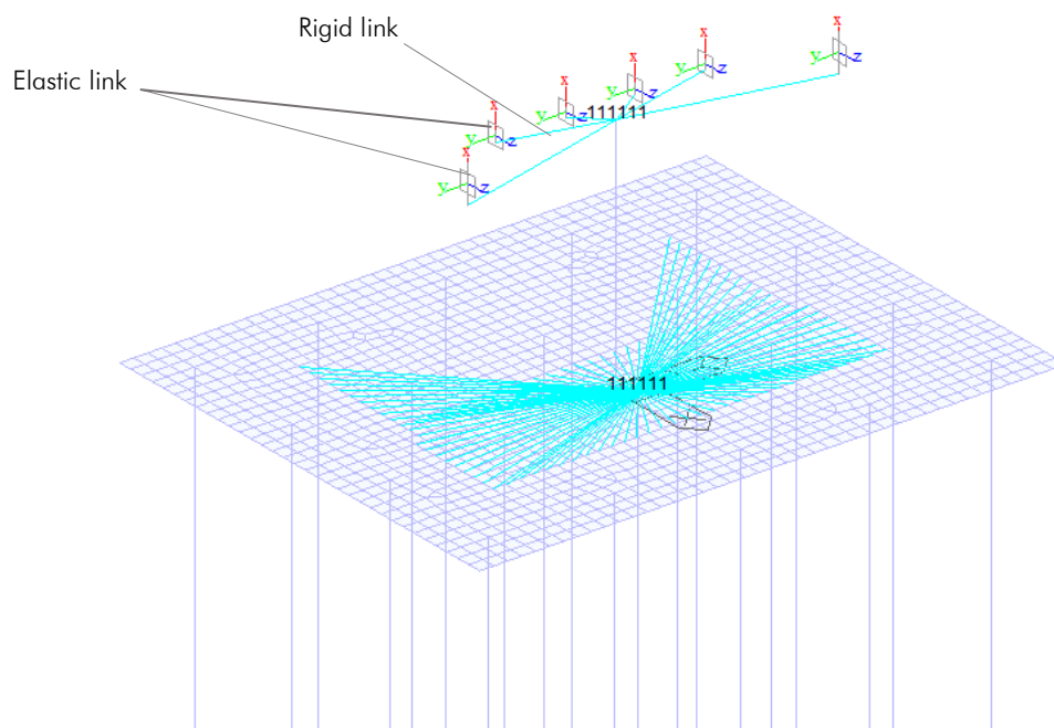
Figura 12: Modellazione tridimensionale agli Elementi Finiti – Vista 3D Wireframe – Sistema dei vincoli interni
