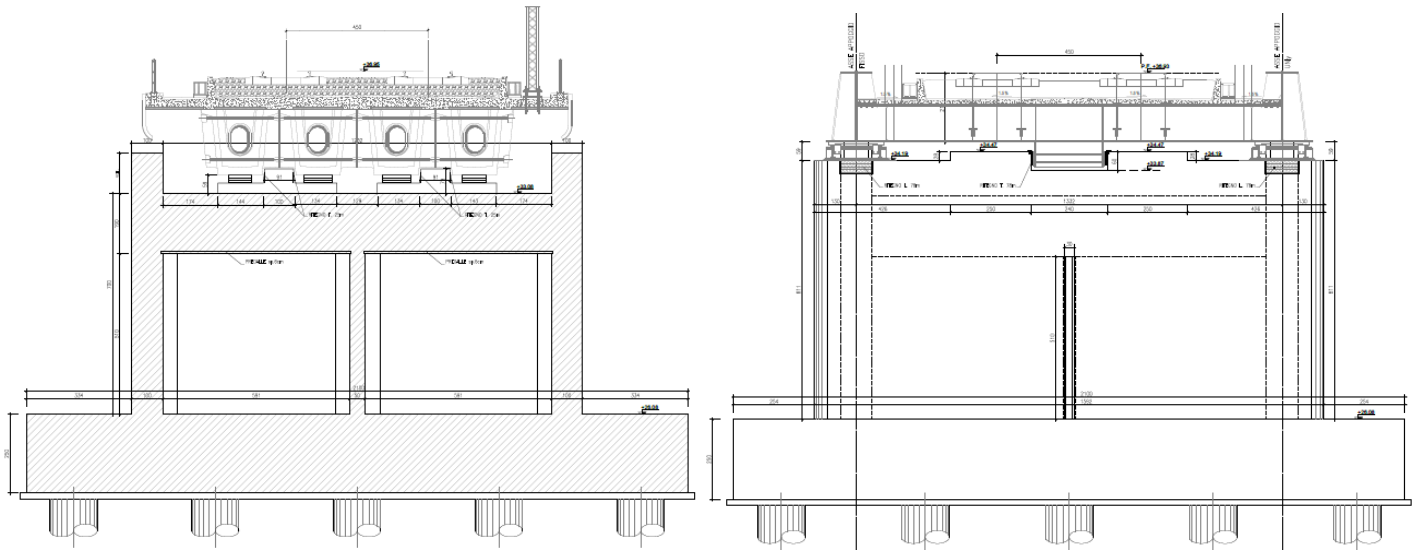
Figura 2: Sezione trasversale lato impalcato L=25m (a sinistra) e lato impalcato metallico L=78m (a destra)
