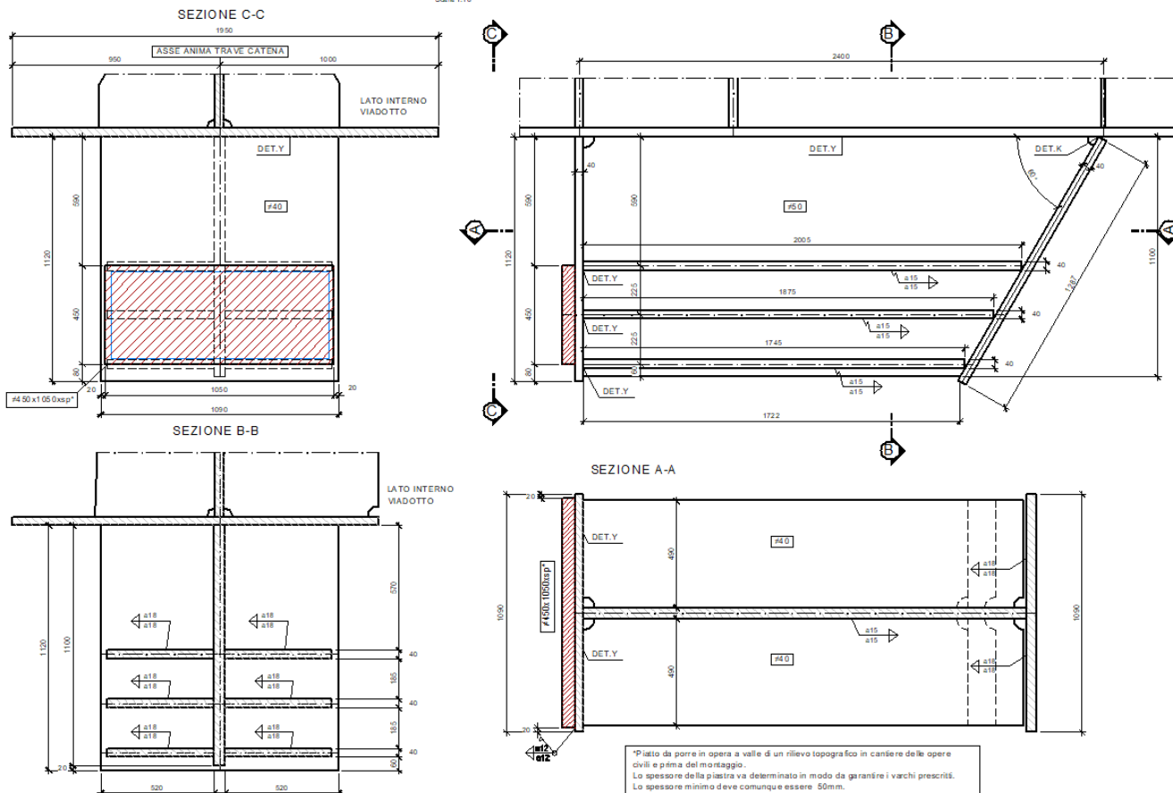
DETTAGLIO RITEGNO LONGITUDINALE LATO APPOGGIO FISSO (PILA P13) Scala 1:10
