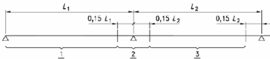
Fig. 2.7.1.2.1-1 – Aree dove si considerano la sezione di mezzzeria o la sezione sull'appoggio
