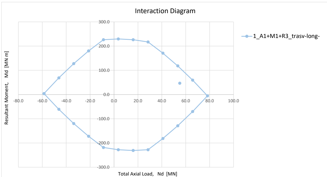
Figura 6 – Dominio di resistenza – condizioni di carico 1_A1+M1+R3_trasv-long
