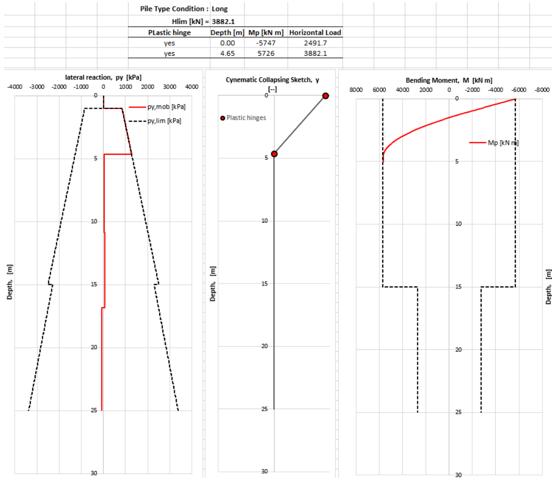
Figura 9 – Verifica carico limite orizzontale – Spalla A- verifica 2
