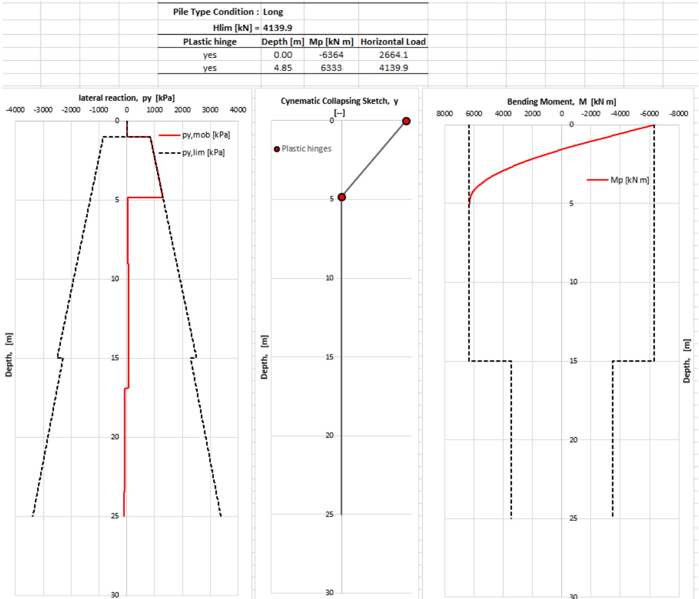
Figura 8 – Verifica carico limite orizzontale – Spalla A- verifica 1
