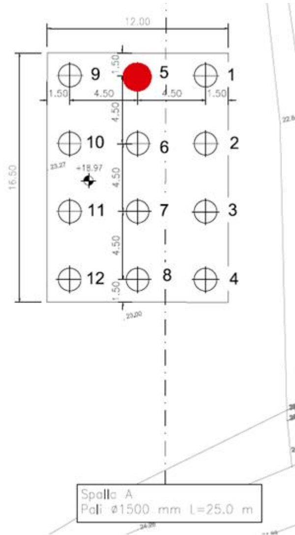
Figura 1 – palificata a 12 pali spalla A - PE
