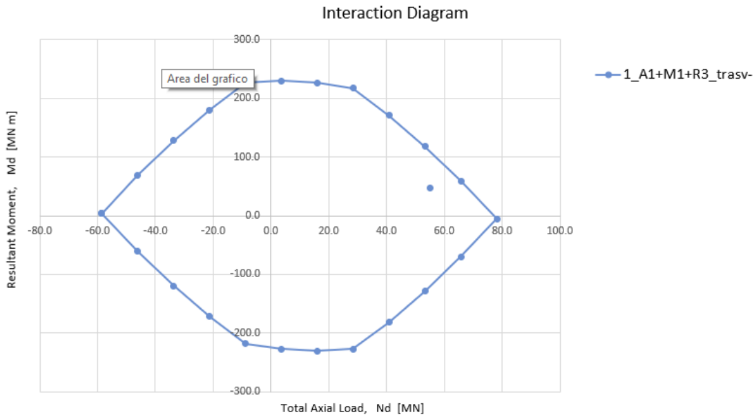
Figura 5 – Dominio di resistenza – condizioni di carico 1_A1+M1+R3_trasv-
