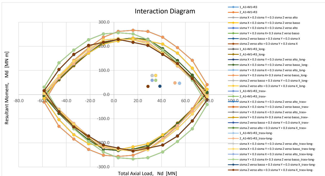
Figura 4 – Dominio di resistenza – tutte le condizioni di carico
