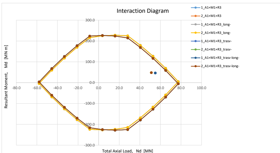
Figura 7 – Dominio di resistenza –in presenza di liquefazione
