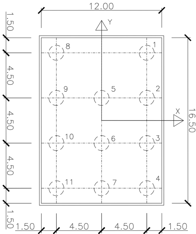
Figura 2 – palificata a 11 pali spalla A come eseguita
