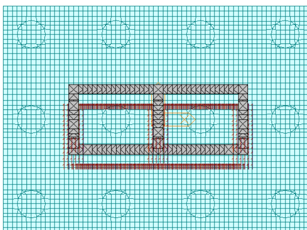
Figura 27 – Sistema di vincoli del modello agli elementi finiti
