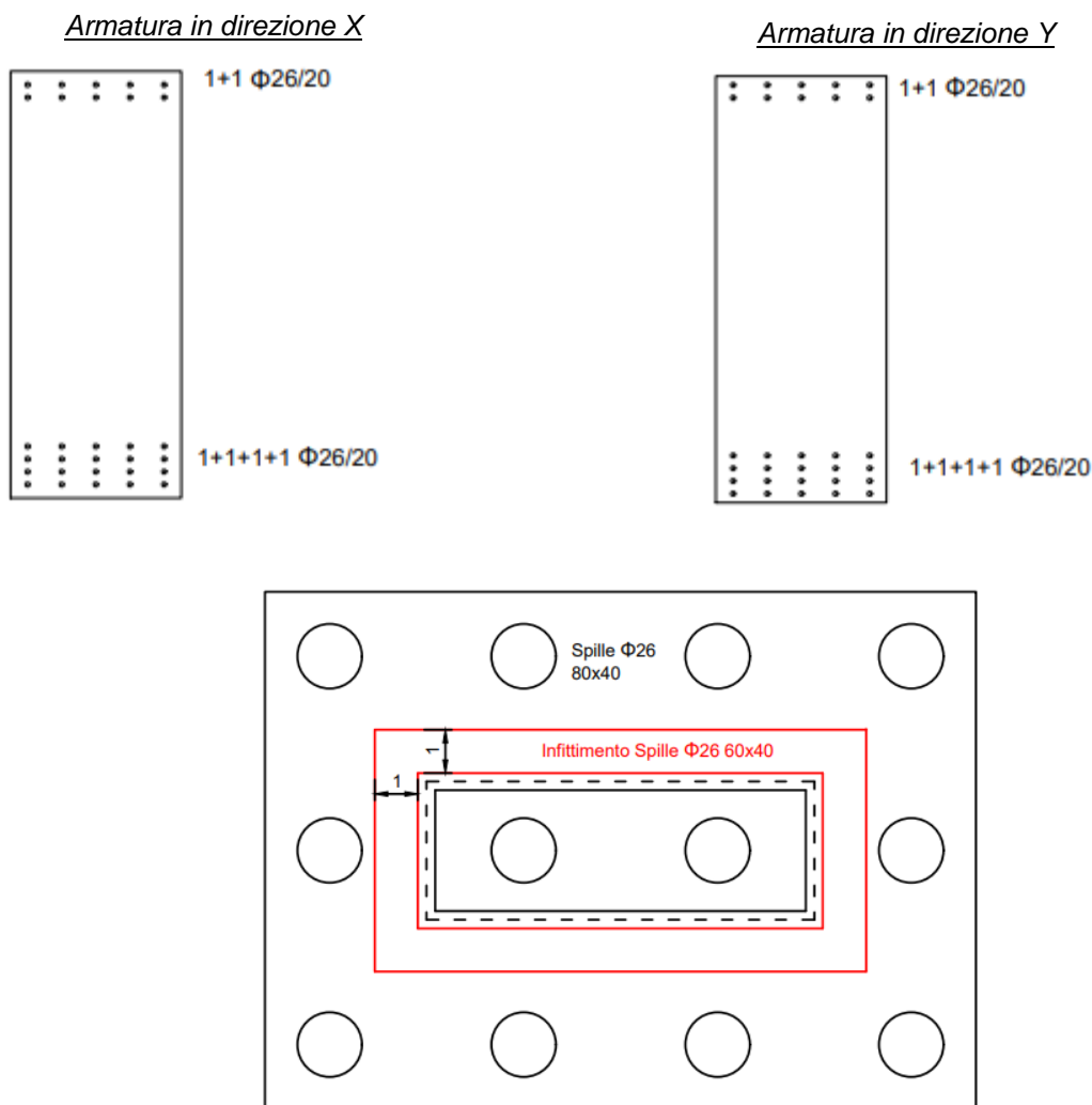
Figura 39 – Armatura a taglio del plinto
