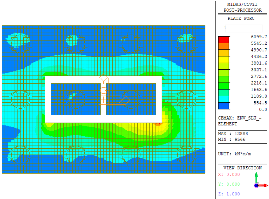
Figura 34 – Wood Armer Moment – Direction 2 – Top (Inviluppo SLU/SLV)
