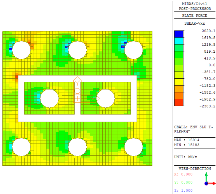
Figura 36 – Vxx, Inviluppo SLU/SLV
