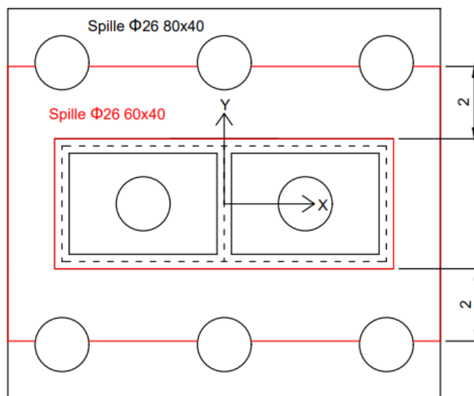
Figura 39 – Armatura a taglio della platea
