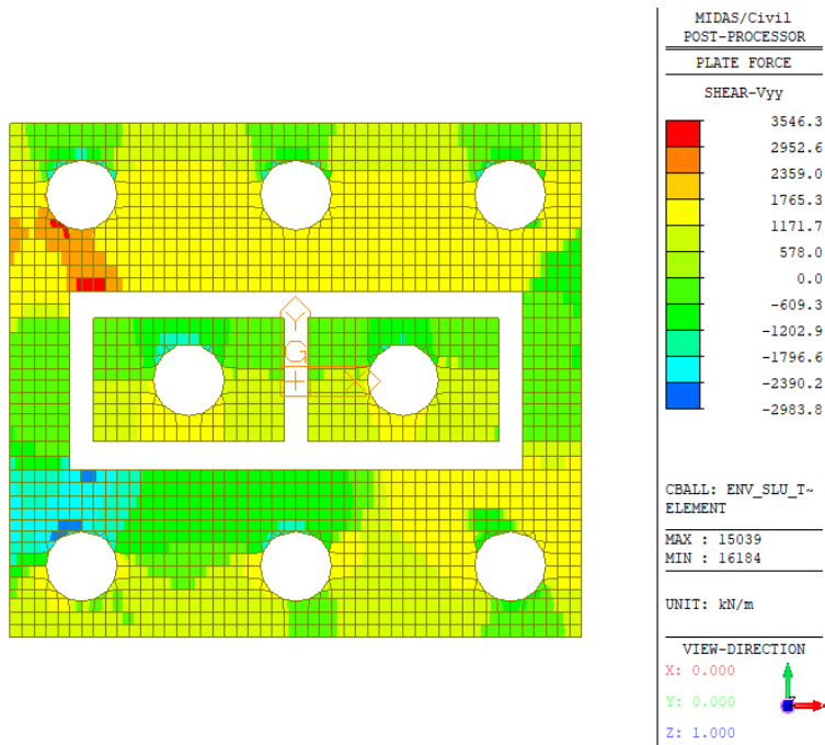
Figura 37 – Vyy, Inviluppo SLU/SLV
