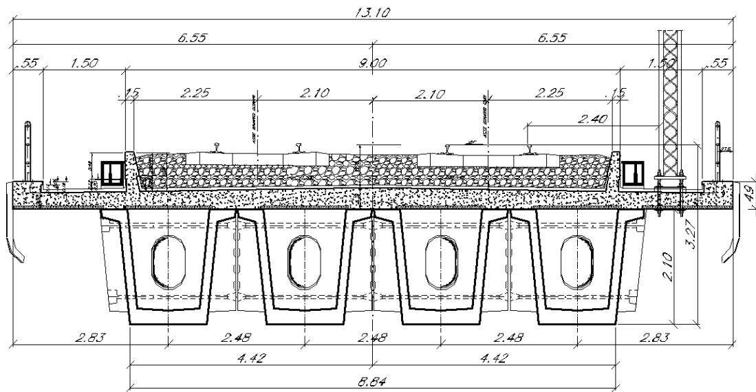
Figura 2 - Sezione impalcato
