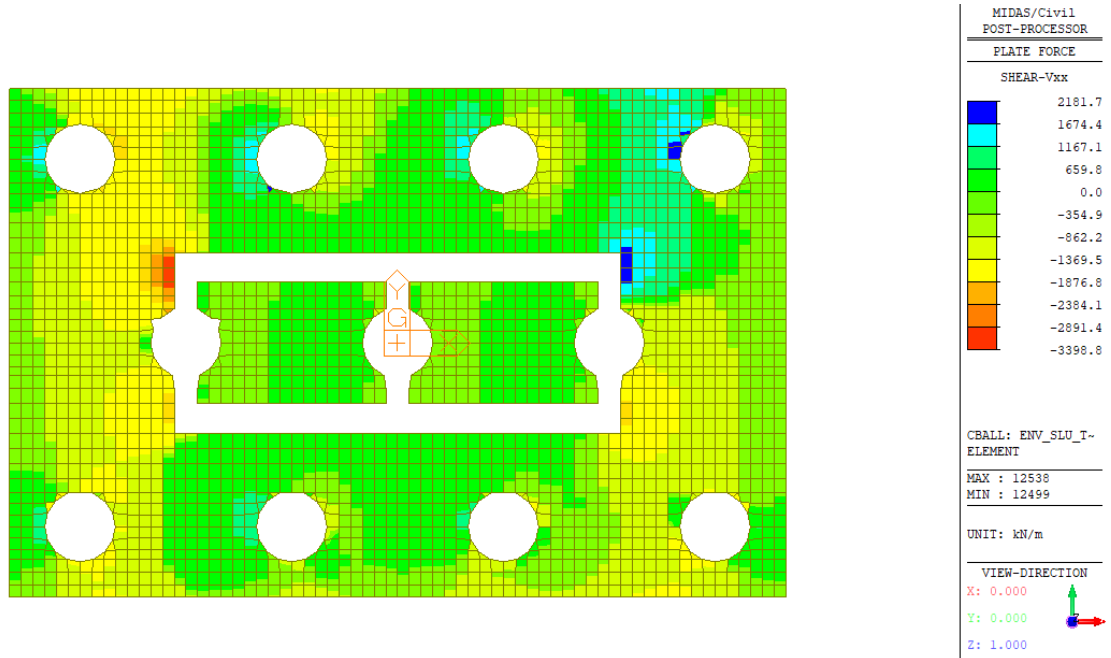
Figura 36 – Vxx, Inviluppo SLU/SLV
