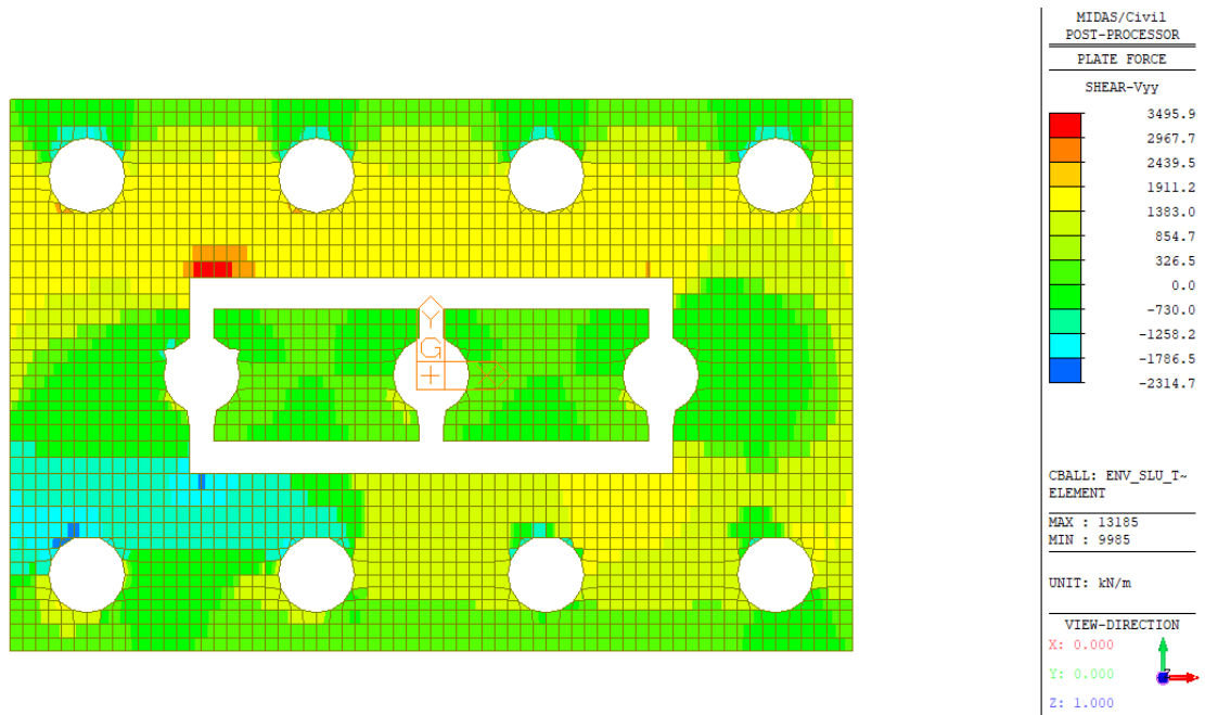
Figura 37 – Vyy, Inviluppo SLU/SLV
