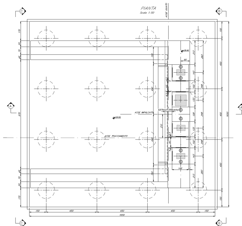
Figura 3 - Pianta Spalla A
