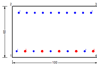
Figura 70 – Sezione implementata in RC-SEC
