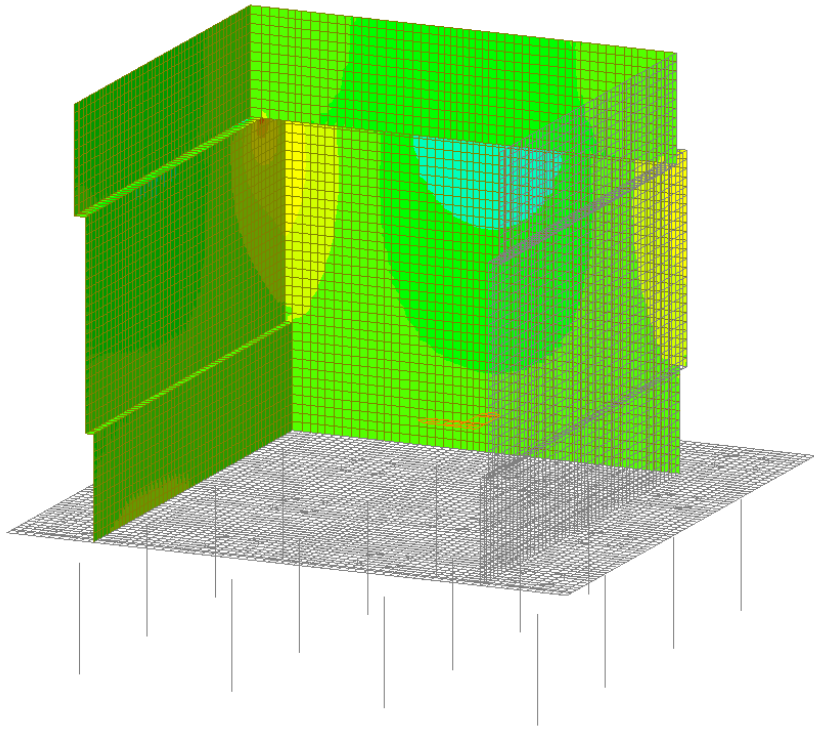
Figura 33 – Involuppo SLE Rara - Mxx
