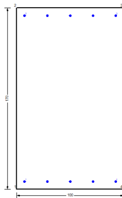
Figura 91 – Sezione implementata in RC-SEC
