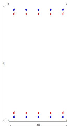
Figura 127 – Sezione implementata in RC-SEC
