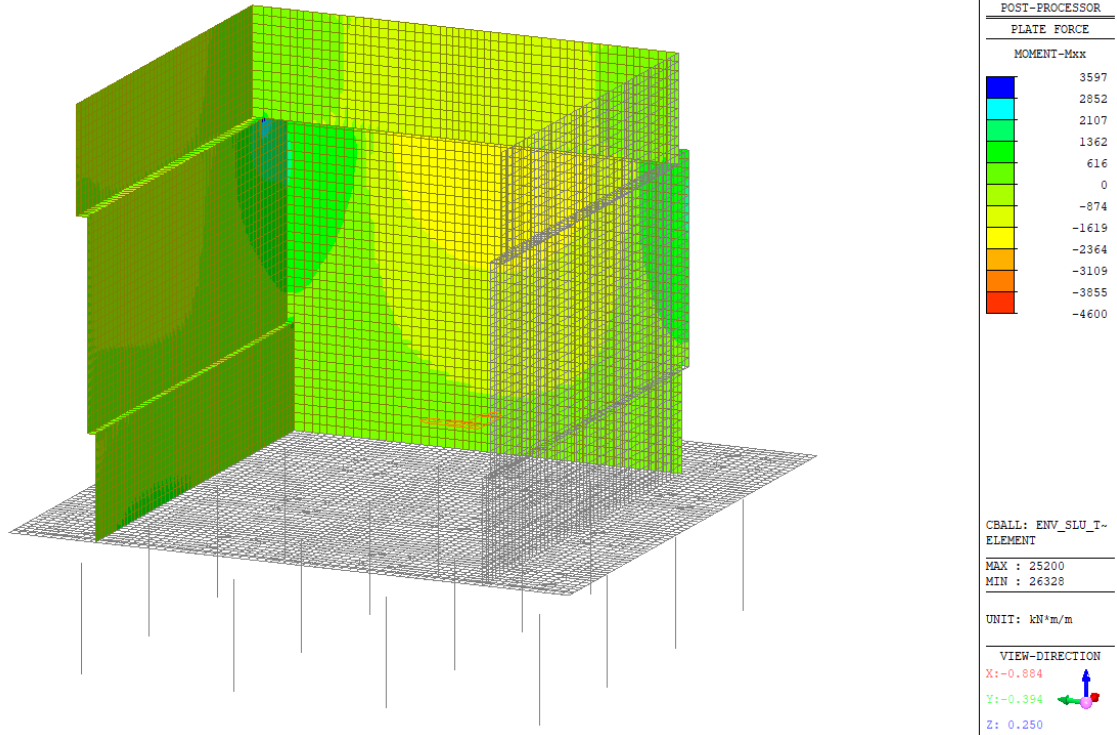
Figura 27 – Involuppo SLU - Mxx
