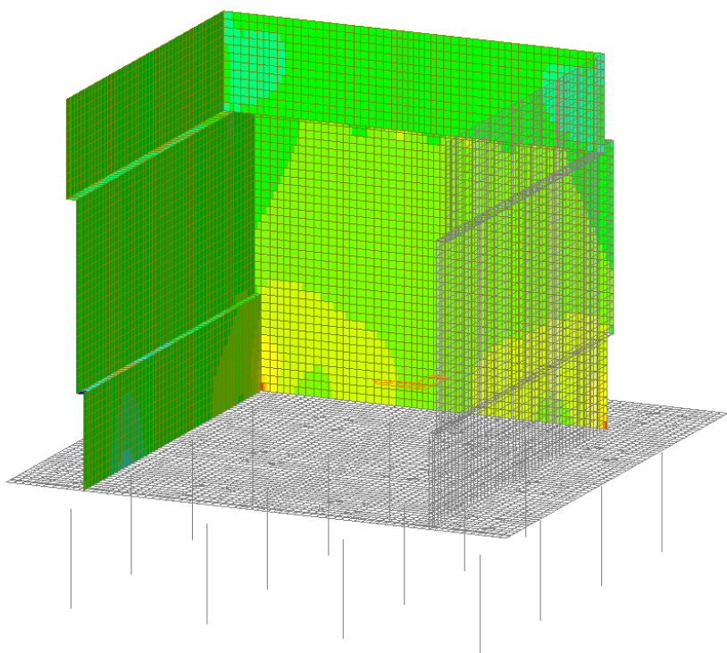
Figura 48 – Involuppo SLE Quasi Permanente - Fyy
