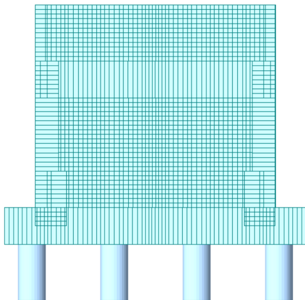
Figura 7 – Vista frontale del modello della spalla
