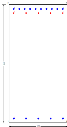
Figura 63 – Sezione implementata in RC-SEC
