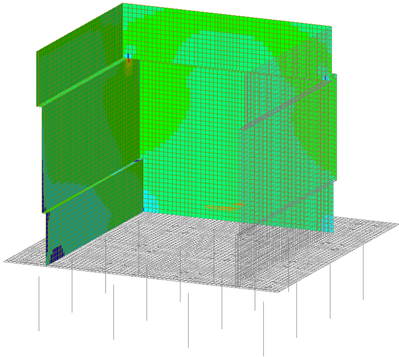
Figura 38 – Involuppo SLE Rara - Vyy
