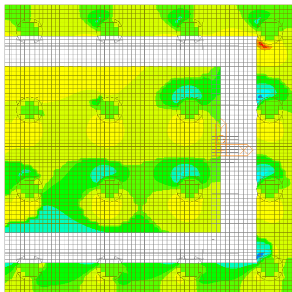
Figura 129 – Involuppo SLU - Vyy
