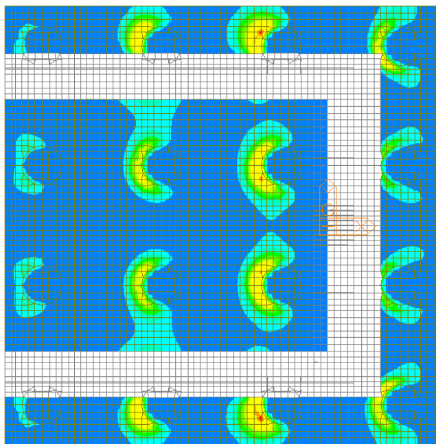
Figura 118 – Involuppo SLE Frequente – W-A Moment Top Direzione 1
