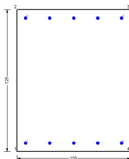
Figura 98 – Sezione implementata in RC-SEC
