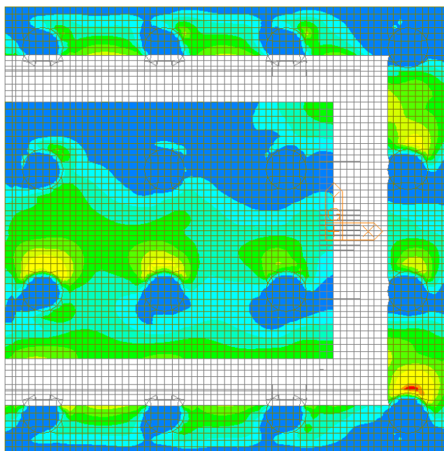
Figura 113 – Involuppo SLU – W-A Moment Bottom Direzione 2
