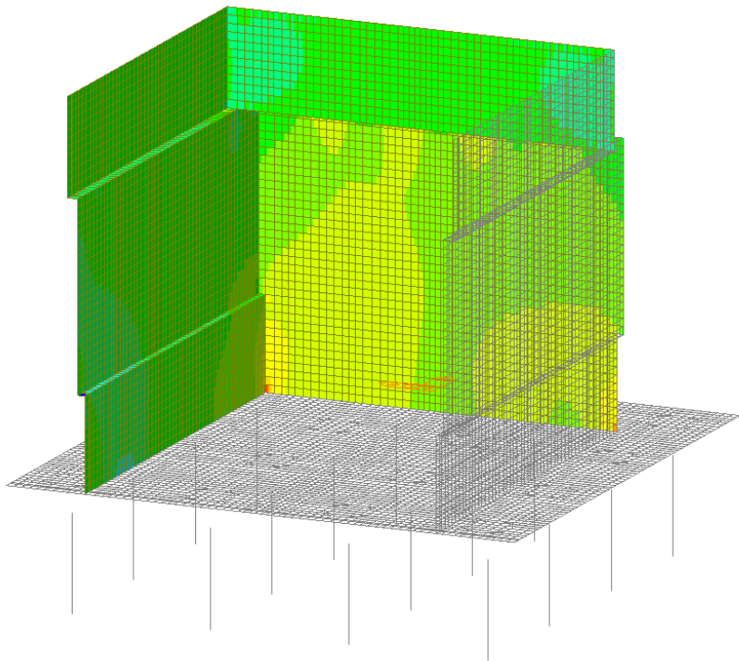
Figura 36 – Involuppo SLE Rara - Fyy
