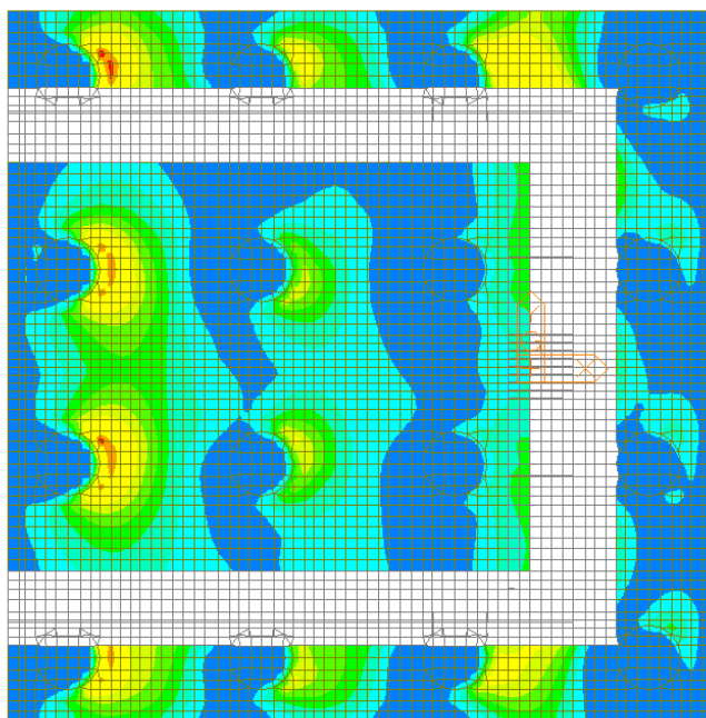
Figura 111 – Involuppo SLU – W-A Moment Bottom Direzione 1
