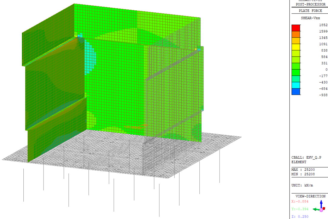
Figura 49 – Involuppo SLE Quasi Permanente - Vxx
