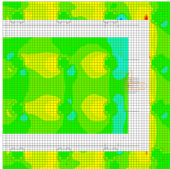
Figura 128 – Involuppo SLU - Vxx
