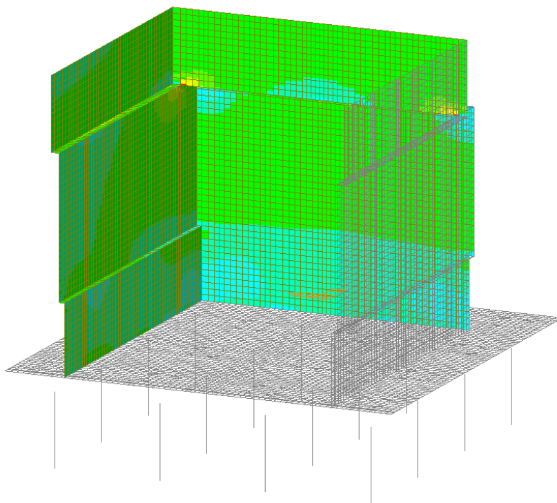
Figura 40 – Involuppo SLE Frequente - Fxx
