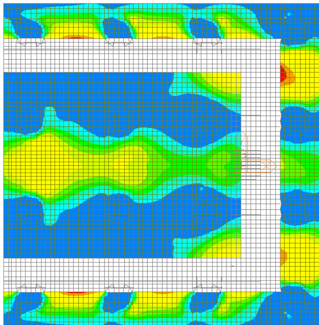
Figura 117 – Involuppo SLE Rara – W-A Moment Bottom Direzione 2
