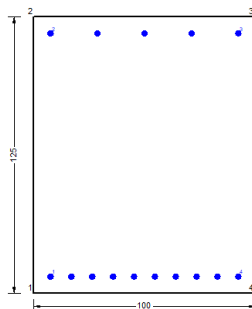
Figura 101 – Sezione implementata in RC-SEC
