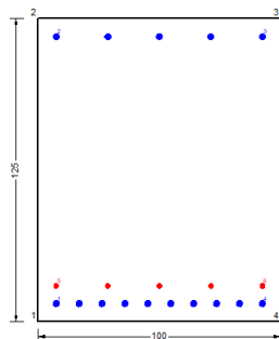
Figura 95 – Sezione implementata in RC-SEC
