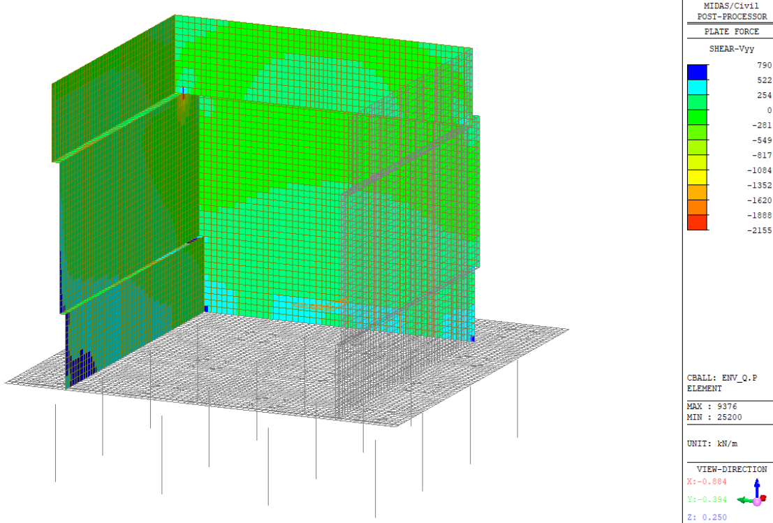
Figura 50 – Involuppo SLE Quasi Permanente - Vyy
