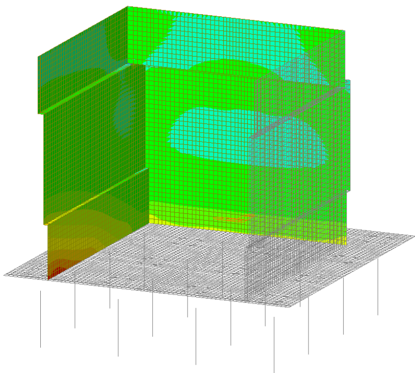
Figura 47 – Involuppo SLE Quasi Permanente - Myy
