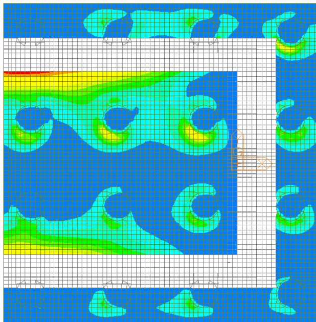
Figura 112 – Involuppo SLU – W-A Moment Top Direzione 2
