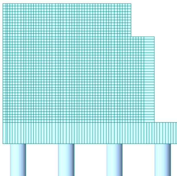
Figura 8 – Vista laterale del modello della spalla
