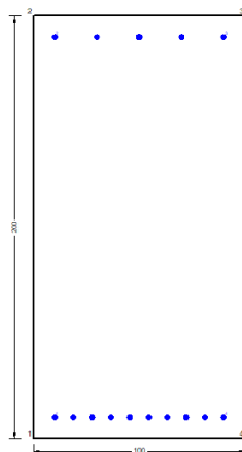
Figura 54 – Sezione implementata in RC-SEC
