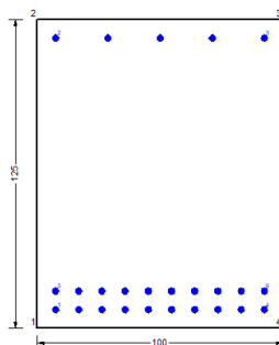
Figura 100 – Sezione implementata in RC-SEC
