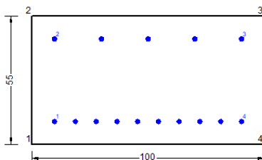
Figura 85 – Sezione implementata in RC-SEC
