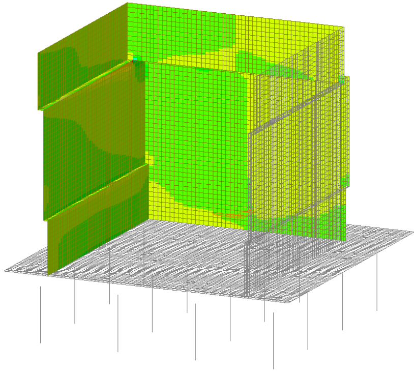
Figura 37 – Involuppo SLE Rara - Vxx
