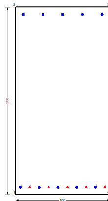
Figura 62 – Sezione implementata in RC-SEC
