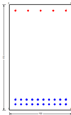
Figura 77 – Sezione implementata in RC-SEC
