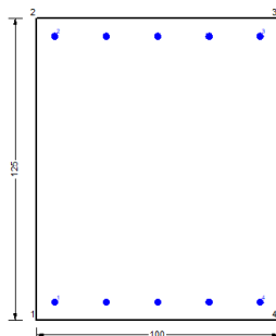
Figura 96 – Sezione implementata in RC-SEC
