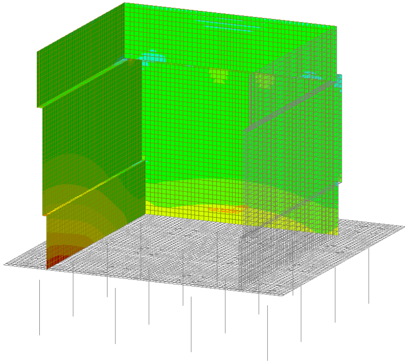
Figura 29 – Involuppo SLU - Myy
