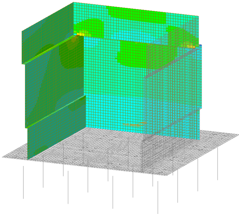
Figura 34 – Involuppo SLE Rara - Fxx
