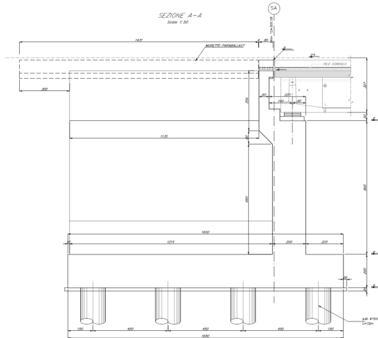
Figura 4 – Sezione longitudinale Spalla A
