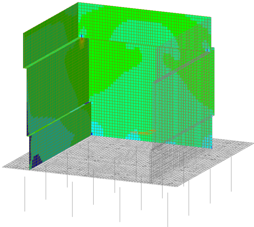
Figura 44 – Involuppo SLE Frequente - Vyy
