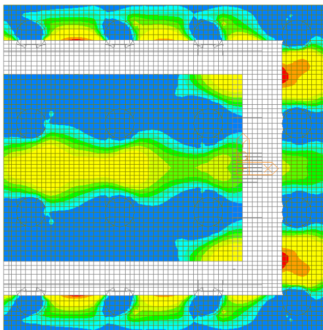
Figura 125 – Involuppo SLE Quasi Permanente – W-A Moment Bottom Direzione 2
