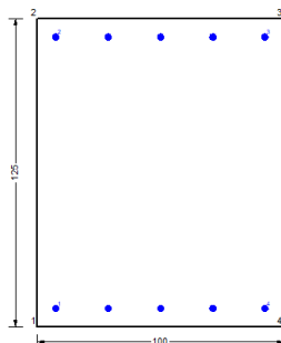
Figura 103 – Sezione implementata in RC-SEC
