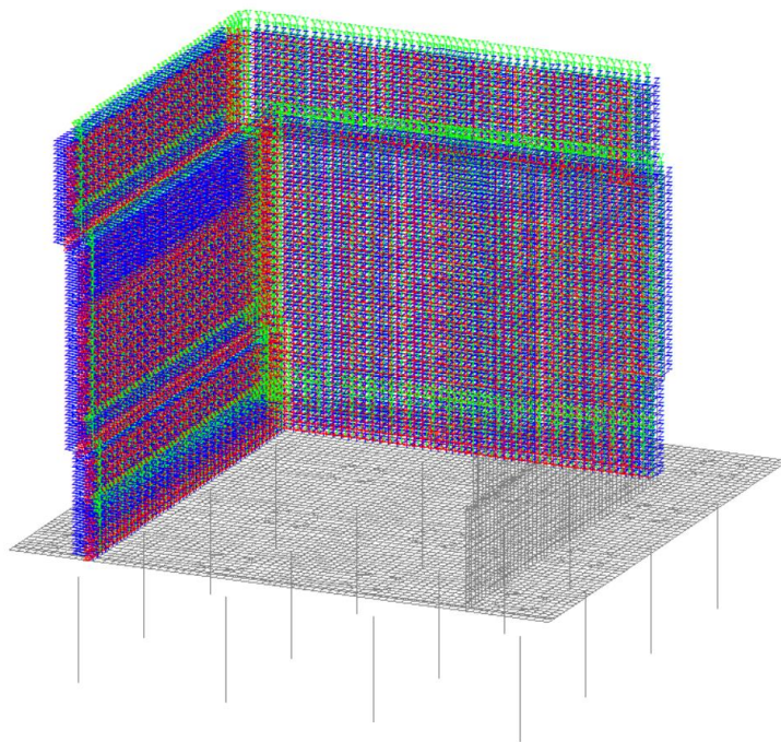
Figura 25 – Assi locali per gli elementi dei muri
