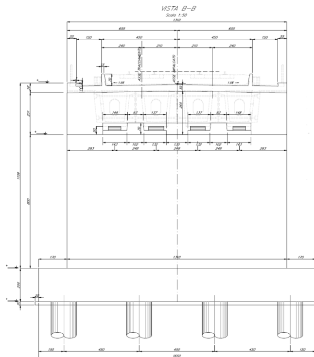
Figura 5 – Sezione trasversale Spalla A
