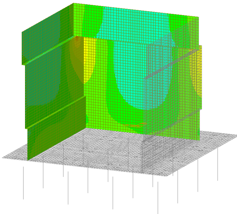
Figura 39 – Involuppo SLE Frequente - Mxx
