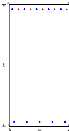
Figura 61 – Sezione implementata in RC-SEC
