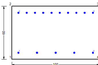
Figura 71 – Sezione implementata in RC-SEC
