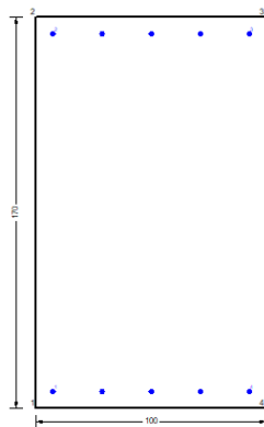
Figura 93 – Sezione implementata in RC-SEC
