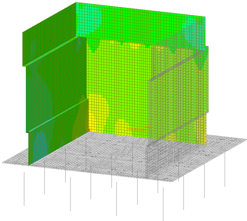
Figura 30 – Involuppo SLU - Fyy
