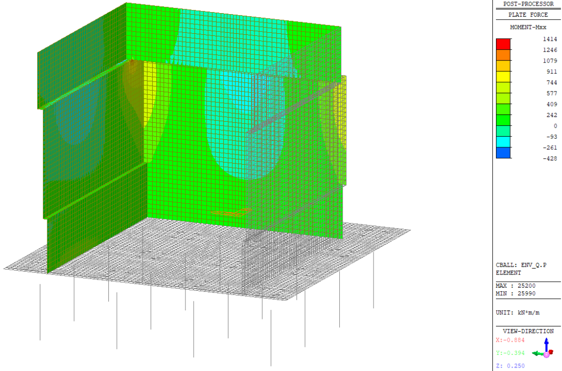
Figura 45 – Involuppo SLE Quasi Permanente - Mxx
