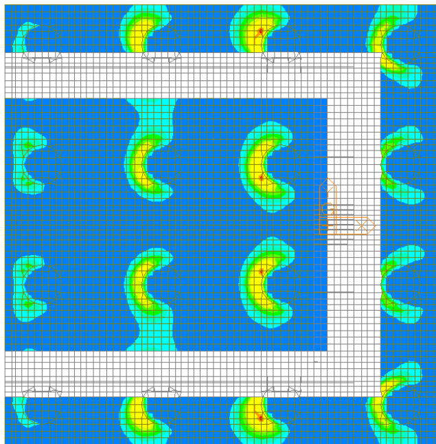
Figura 122 – Involuppo SLE Quasi Permanente – W-A Moment Top Direzione 1
