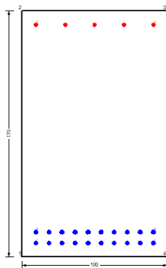
Figura 78 – Sezione implementata in RC-SEC
