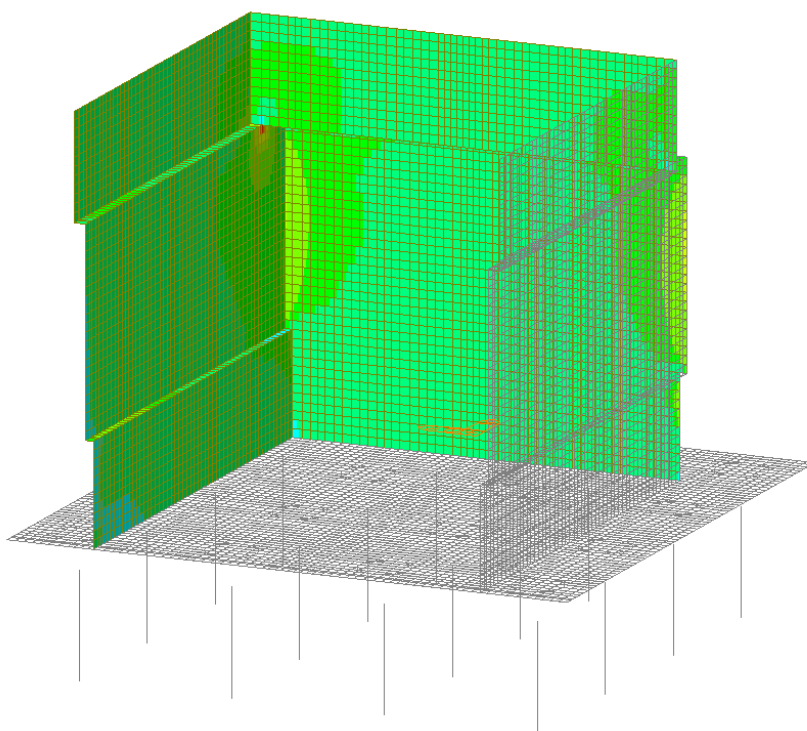
Figura 32 – Involuppo SLU - Vyy
