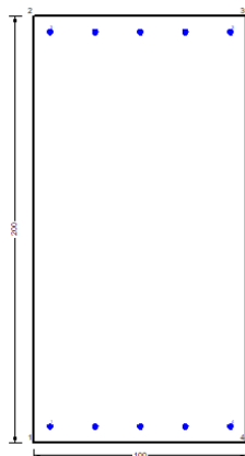
Figura 58 – Sezione implementata in RC-SEC
