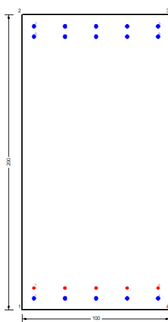
Figura 126 – Sezione implementata in RC-SEC
