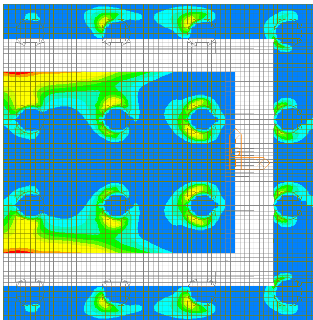
Figura 124 – Involuppo SLE Quasi Permanente – W-A Moment Top Direzione 2
