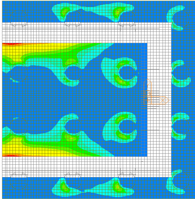
Figura 116 – Involuppo SLE Rara – W-A Moment Top Direzione 2
