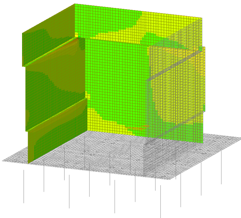
Figura 31 – Involuppo SLU - Vxx
