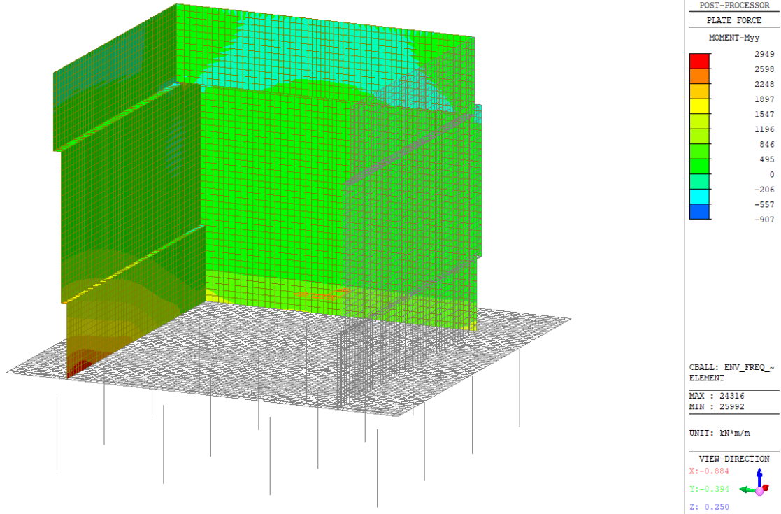
Figura 41 – Involuppo SLE Frequente - Myy
