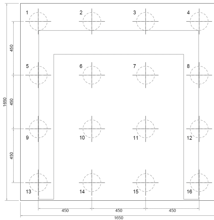
Figura 131 – Disposizione e numerazione dei pali di fondazione
