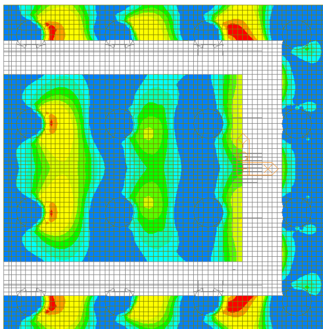
Figura 123 – Involuppo SLE Quasi Permanente – W-A Moment Bottom Direzione 1
