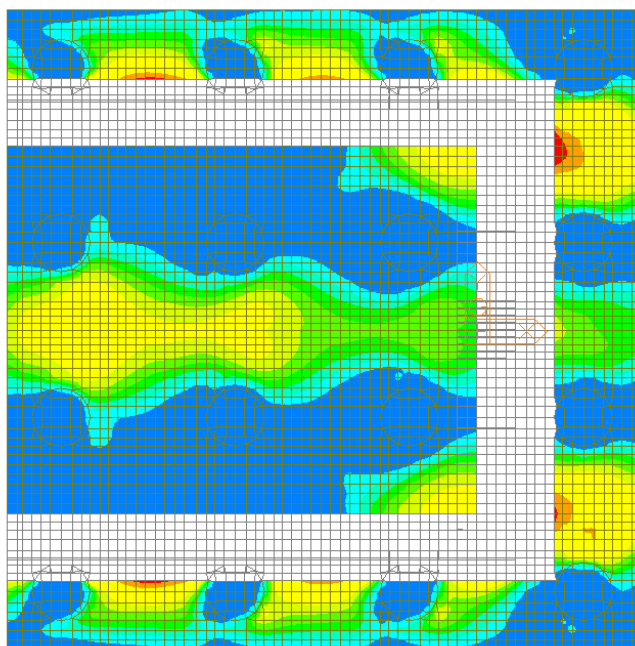
Figura 121 – Involuppo SLE Frequente – W-A Moment Bottom Direzione 2
