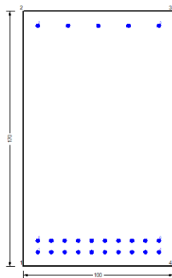
Figura 76 – Sezione implementata in RC-SEC
