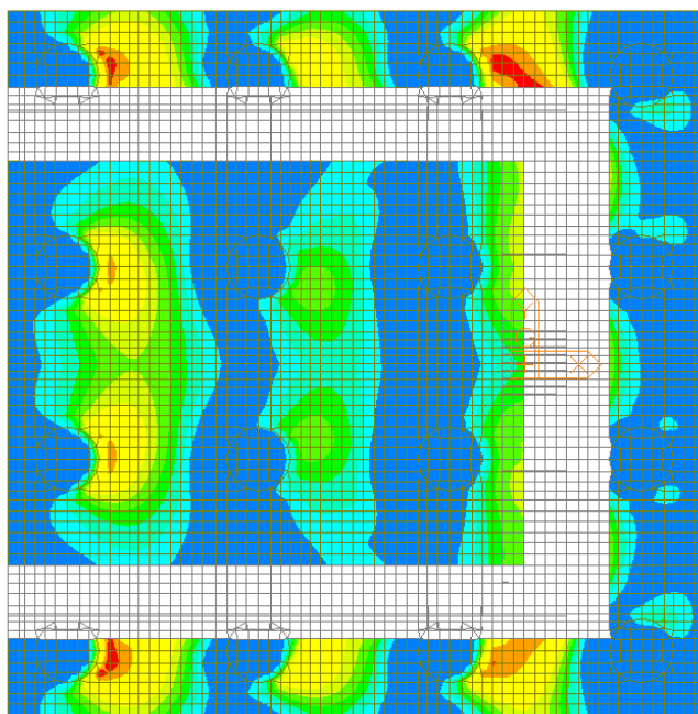
Figura 119 – Involuppo SLE Frequente – W-A Moment Bottom Direzione 1
