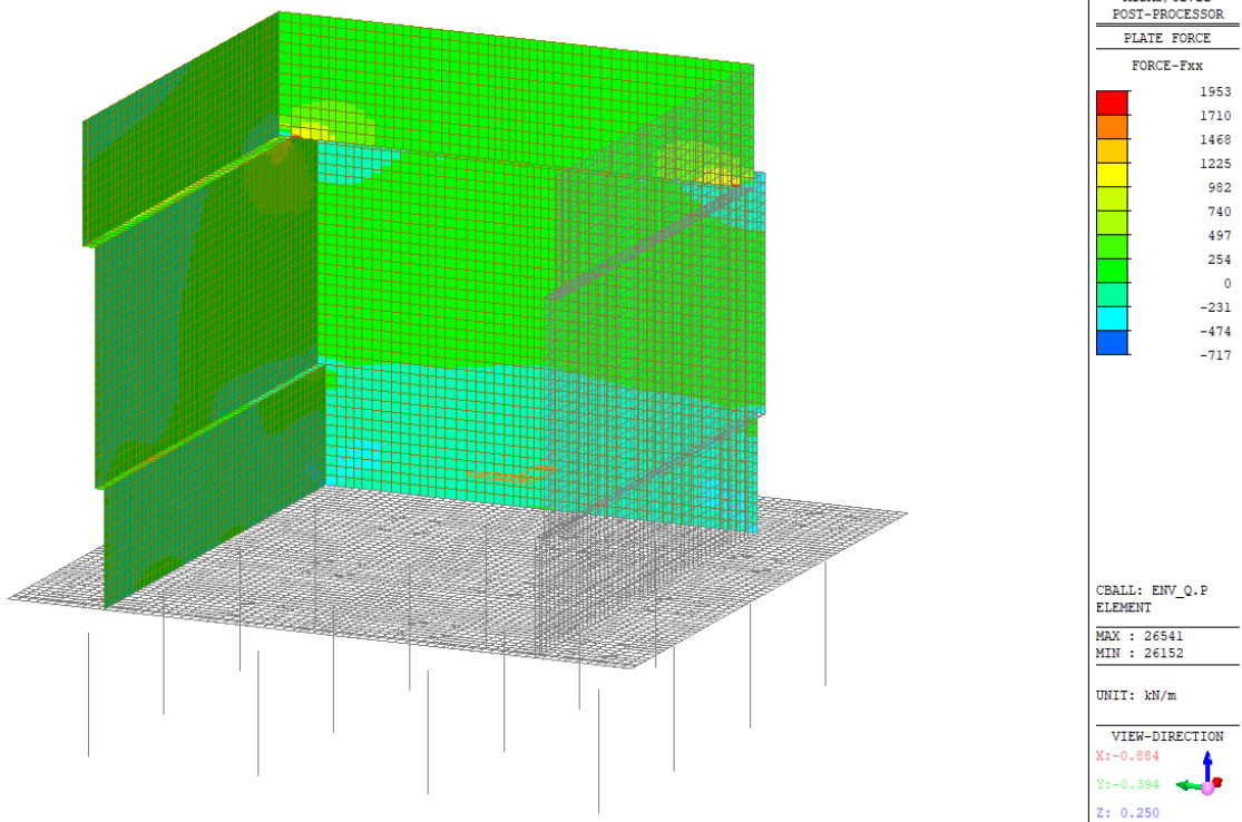
Figura 46 – Involuppo SLE Quasi Permanente - Fxx
