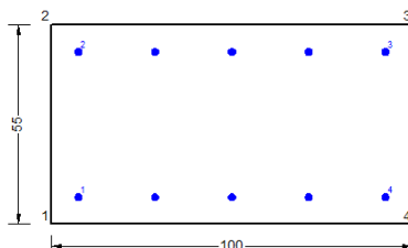
Figura 109 – Sezione implementata in RC-SEC
