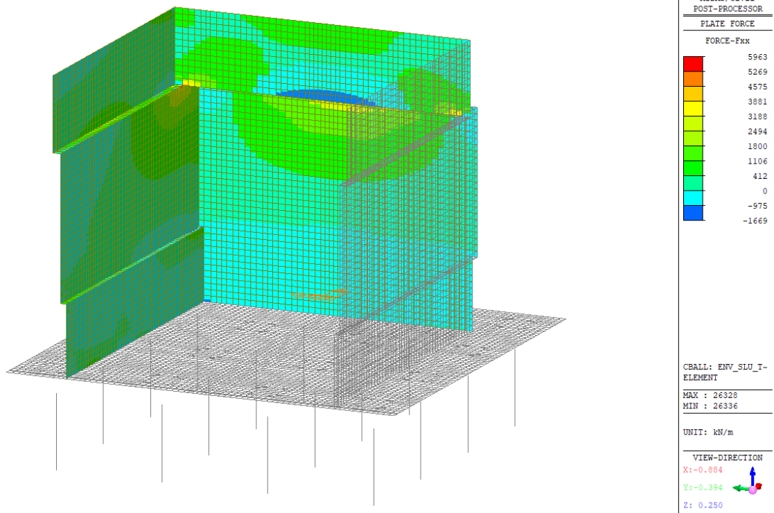
Figura 28 – Involuppo SLU - Fxx
