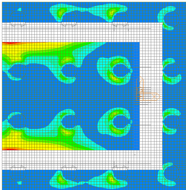
Figura 120 – Involuppo SLE Frequente – W-A Moment Top Direzione 2
