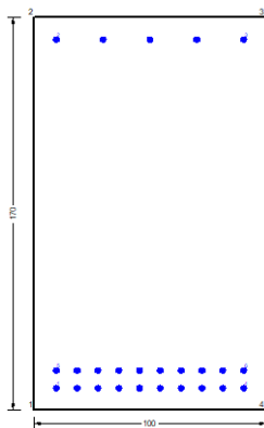
Figura 75 – Sezione implementata in RC-SEC
