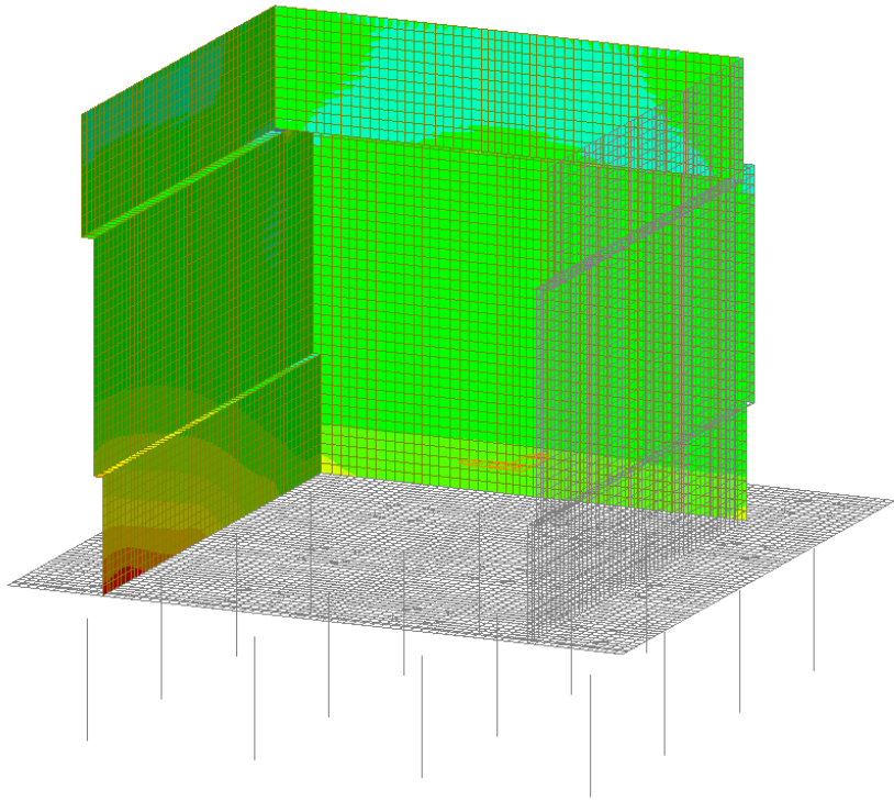
Figura 35 – Involuppo SLE Rara - Myy
