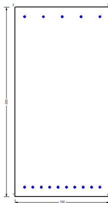
Figura 53 – Sezione implementata in RC-SEC
