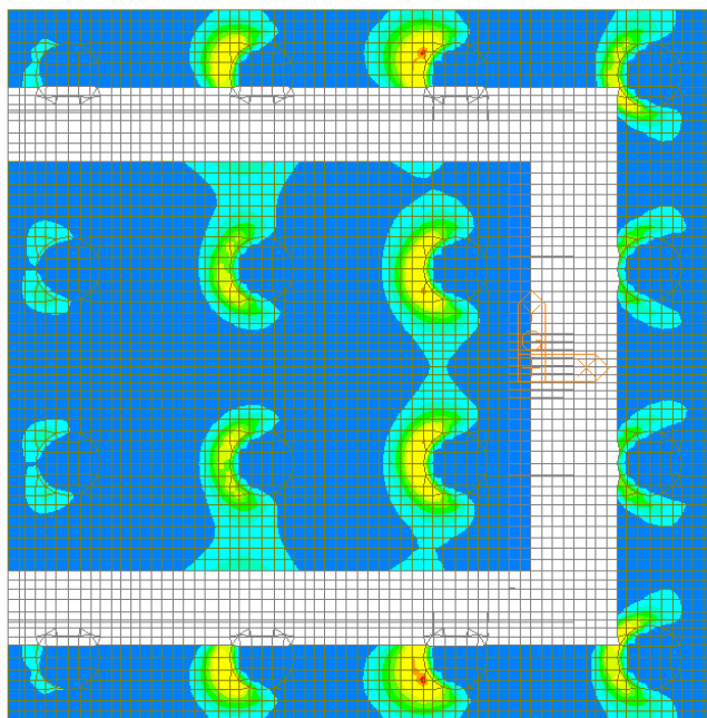
Figura 114 – Involuppo SLE Rara – W-A Moment Top Direzione 1
