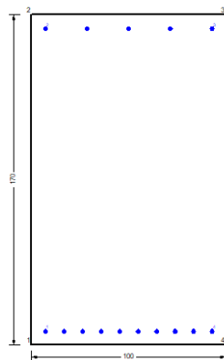
Figura 90 – Sezione implementata in RC-SEC
