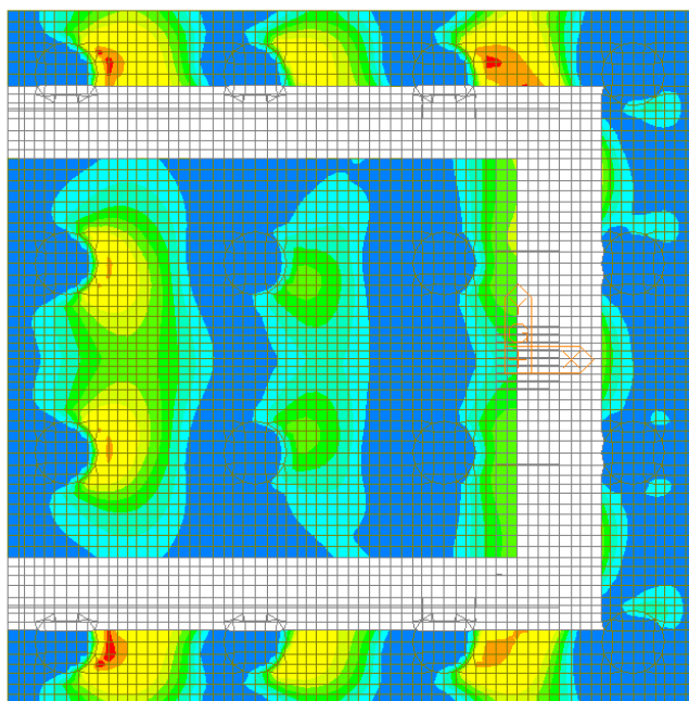
Figura 115 – Involuppo SLE Rara – W-A Moment Bottom Direzione 1
