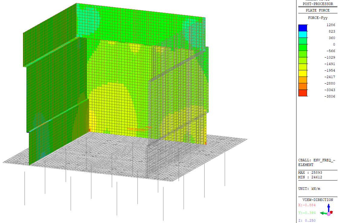
Figura 42 – Involuppo SLE Frequente - Fyy
