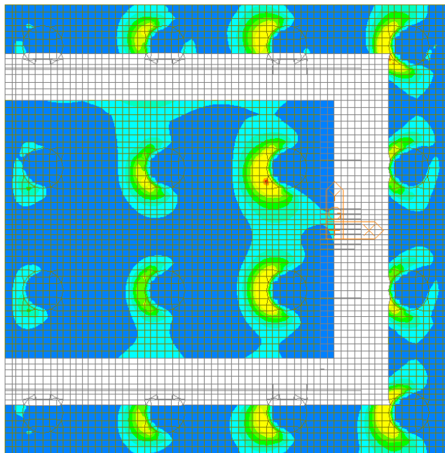
Figura 110 – Involuppo SLU – W-A Moment Top Direzione 1
