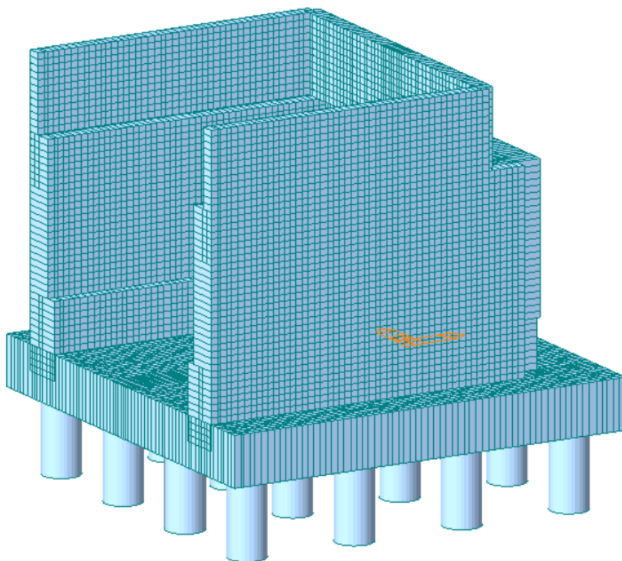
Figura 6 – Vista prospettica del modello della spalla
