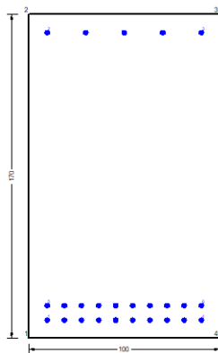
Figura 74 – Sezione implementata in RC-SEC
