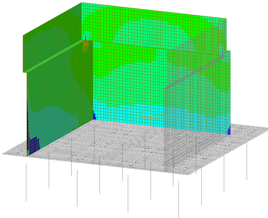
Figura 50 – Involuppo SLE Quasi Permanente - V yy
