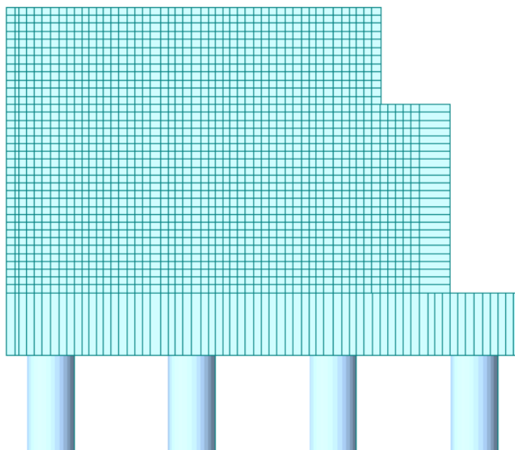
Figura 8 – Vista laterale del modello della spalla
