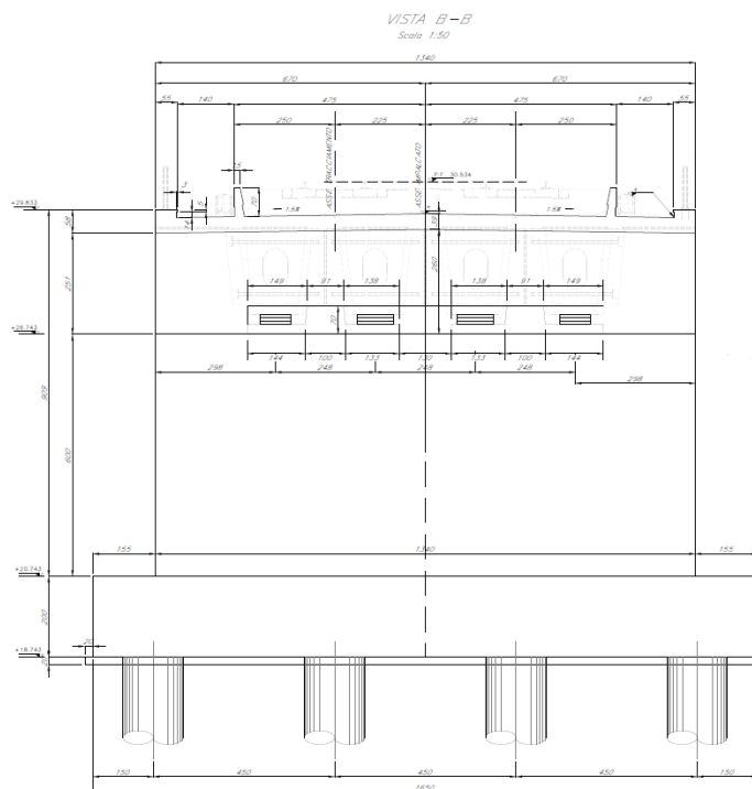
Figura 5 – Sezione trasversale Spalla B
