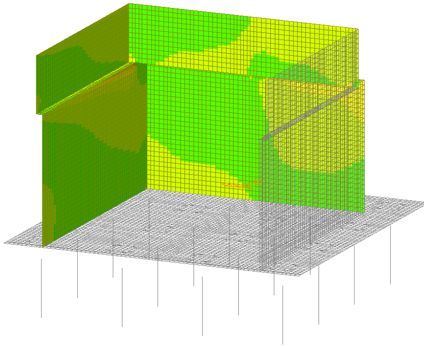
Figura 31 – Involuppo SLU - Vxx
