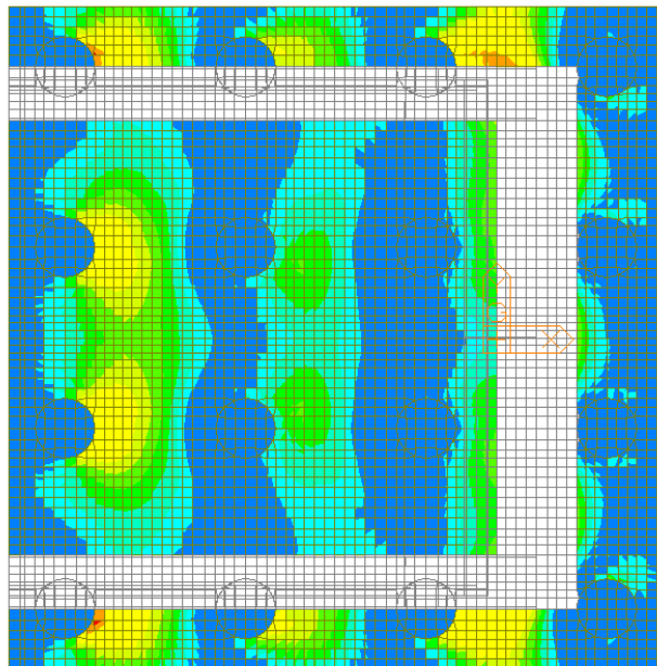
Figura 106 – Involuppo SLE Frequente – W-A Moment Bottom Direzione 1
