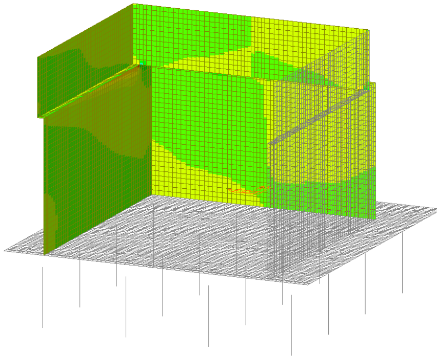
Figura 43 – Involuppo SLE Frequente - V xx
