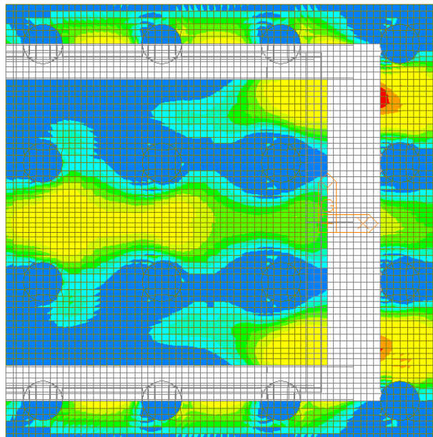
Figura 108 – Involuppo SLE Frequente – W-A Moment Bottom Direzione 2
