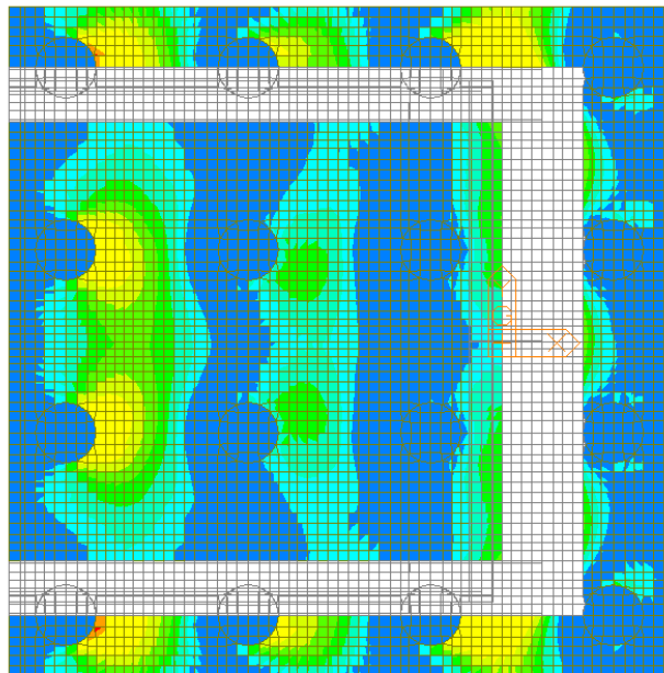
Figura 102 – Involuppo SLE Rara – W-A Moment Bottom Direzione 1
