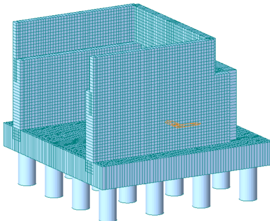
Figura 6 – Vista prospettica del modello della spalla
