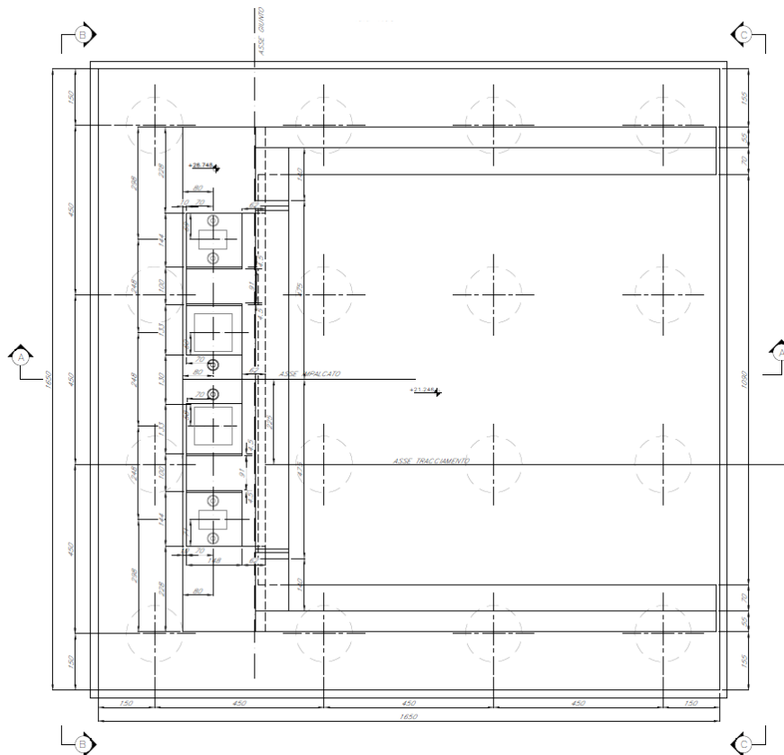
Figura 3 - Pianta Spalla B
