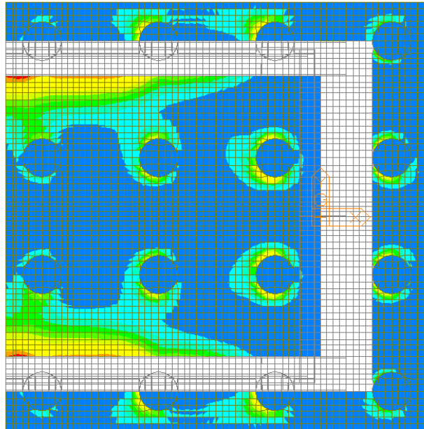
Figura 103 – Involuppo SLE Rara – W-A Moment Top Direzione 2
