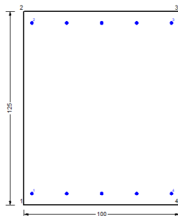
Figura 88 – Sezione implementata in RC-SEC
