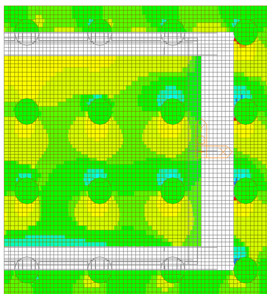
Figura 116 – Involuppo SLU - Vyy
