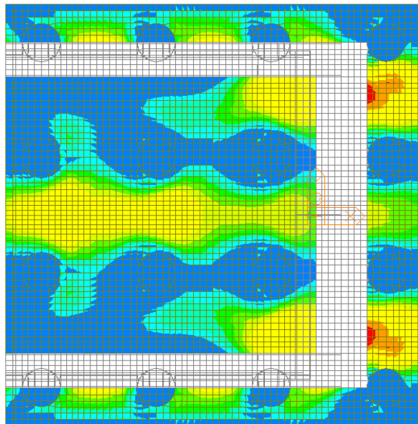
Figura 112 – Involuppo SLE Quasi Permanente – W-A Moment Bottom Direzione 2
