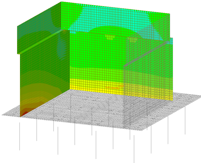
Figura 47 – Involuppo SLE Quasi Permanente - Myy
