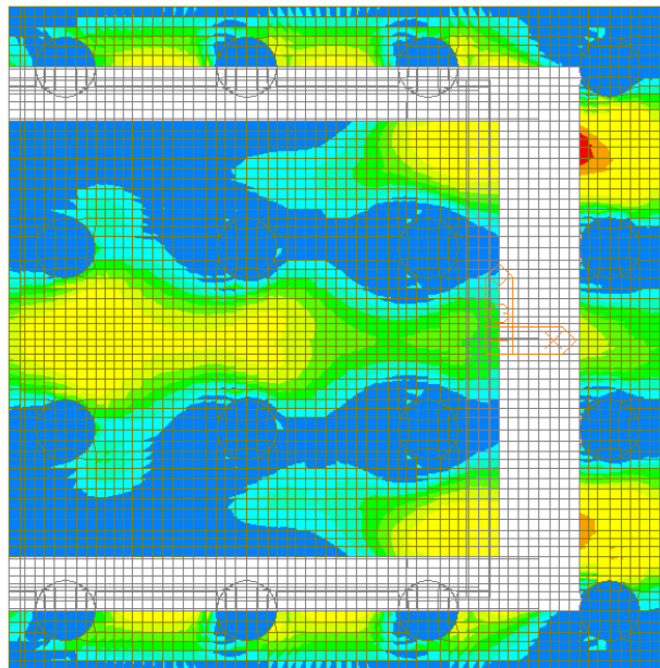
Figura 104 – Involuppo SLE Rara – W-A Moment Bottom Direzione 2
