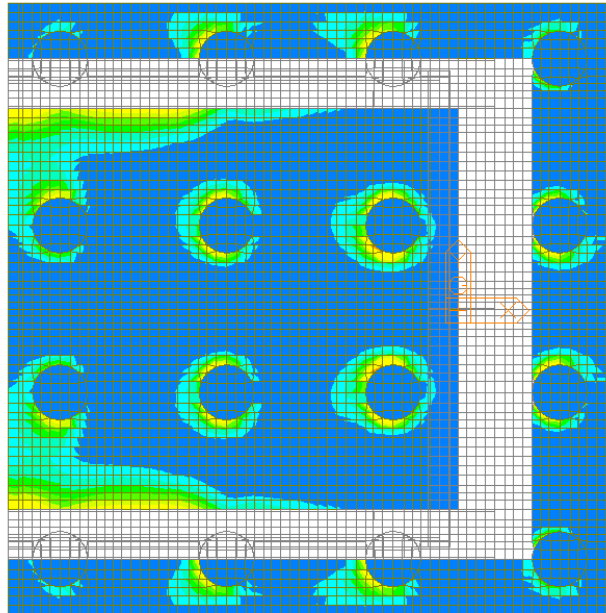
Figura 111 – Involuppo SLE Quasi Permanente – W-A Moment Top Direzione 2
