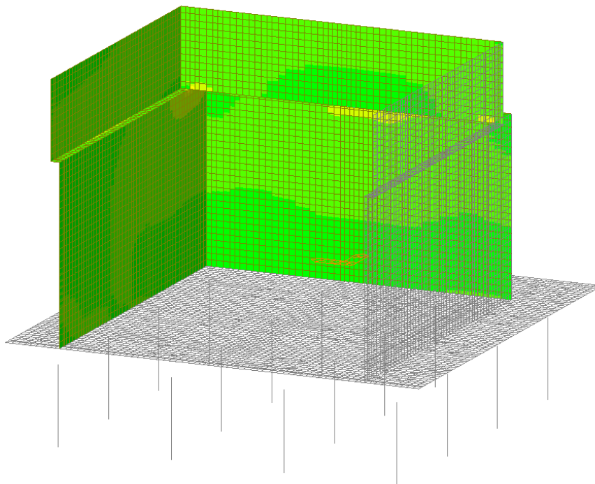
Figura 28 – Involuppo SLU - Fxx
