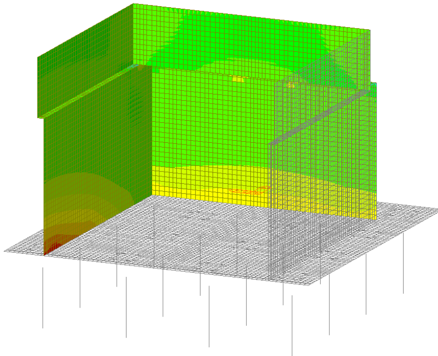
Figura 41 – Involuppo SLE Frequente - Myy
