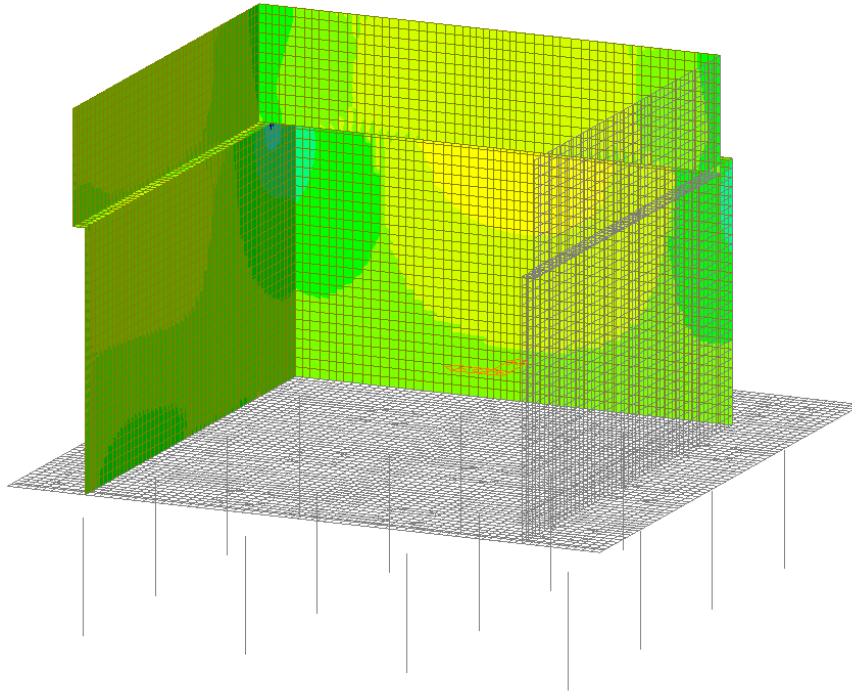
Figura 27 – Involuppo SLU - Mxx
