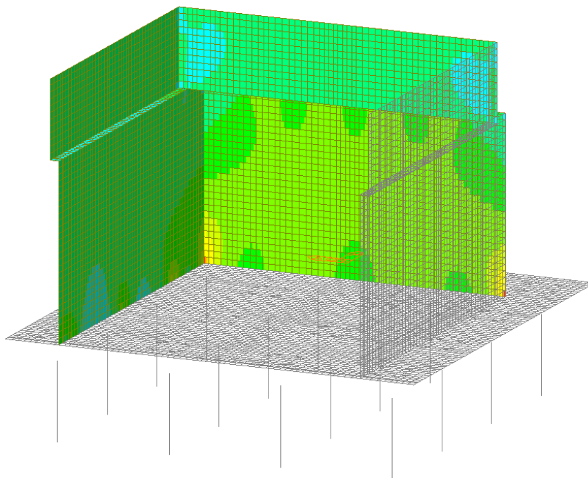
Figura 48 – Involuppo SLE Quasi Permanente - Fyy
