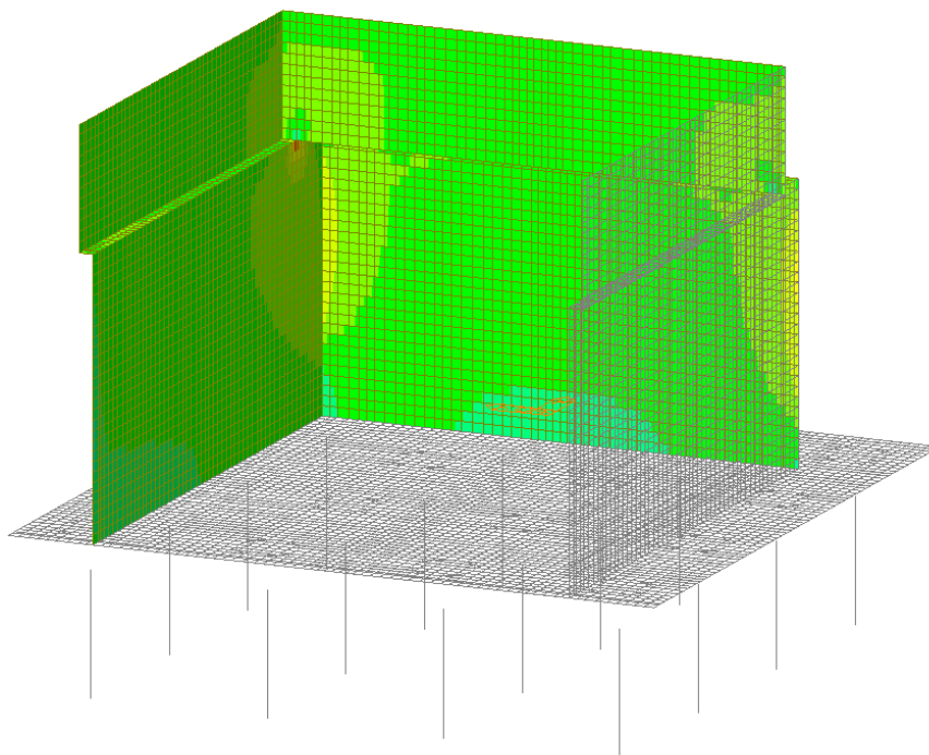
Figura 32 – Involuppo SLU - Vyy
