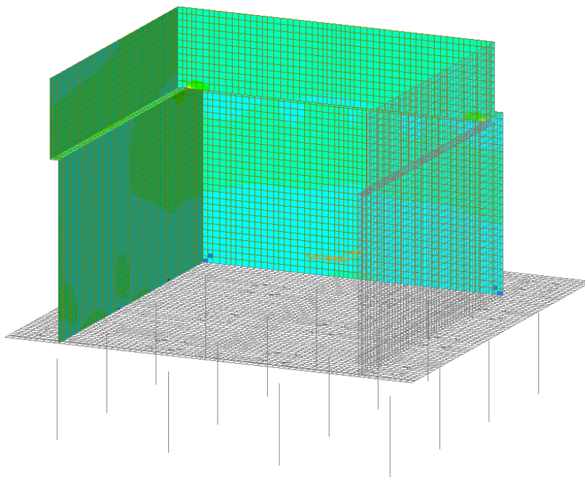
Figura 46 – Involuppo SLE Quasi Permanente - Fxx
