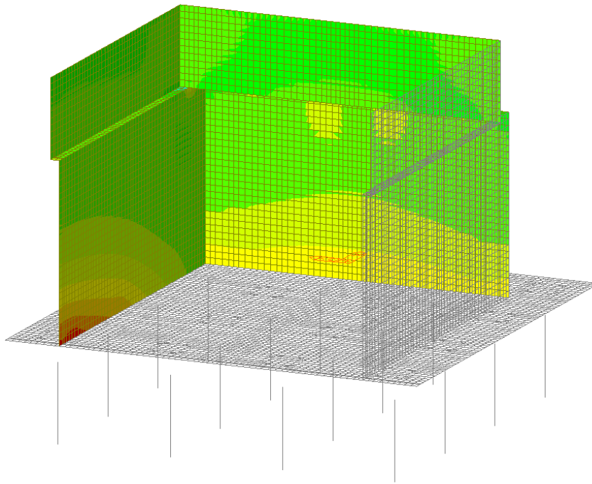
Figura 35 – Involuppo SLE Rara - Myy
