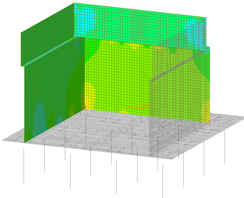
Figura 42 – Involuppo SLE Frequente - Fyy
