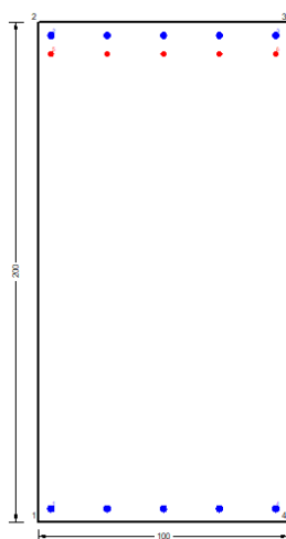
Figura 114 – Sezione implementata in RC-SEC
