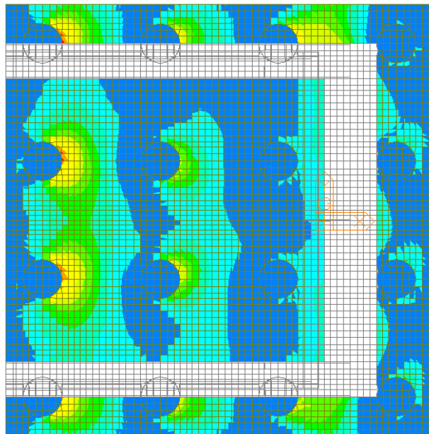
Figura 98 – Inviluppo SLU – W-A Moment Bottom Direzione 1
