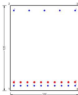
Figura 87 – Sezione implementata in RC-SEC
