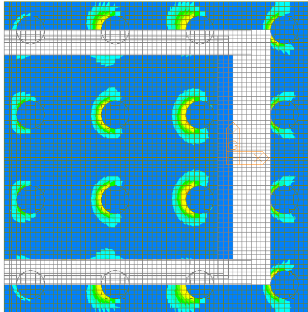
Figura 109 – Inviluppo SLE Quasi Permanente – W-A Moment Top Direzione 1
