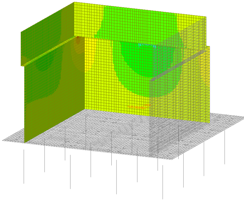
Figura 33 – Involuppo SLE Rara - Mxx
