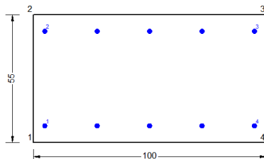
Figura 93 – Sezione implementata in RC-SEC
