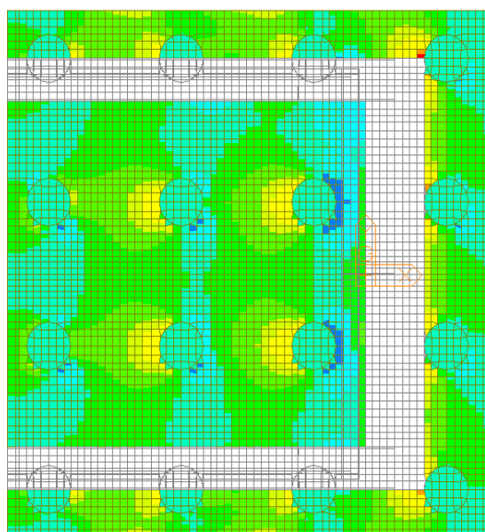
Figura 115 – Involuppo SLU - Vxx
