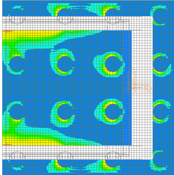
Figura 107 – Involuppo SLE Frequente – W-A Moment Top Direzione 2
