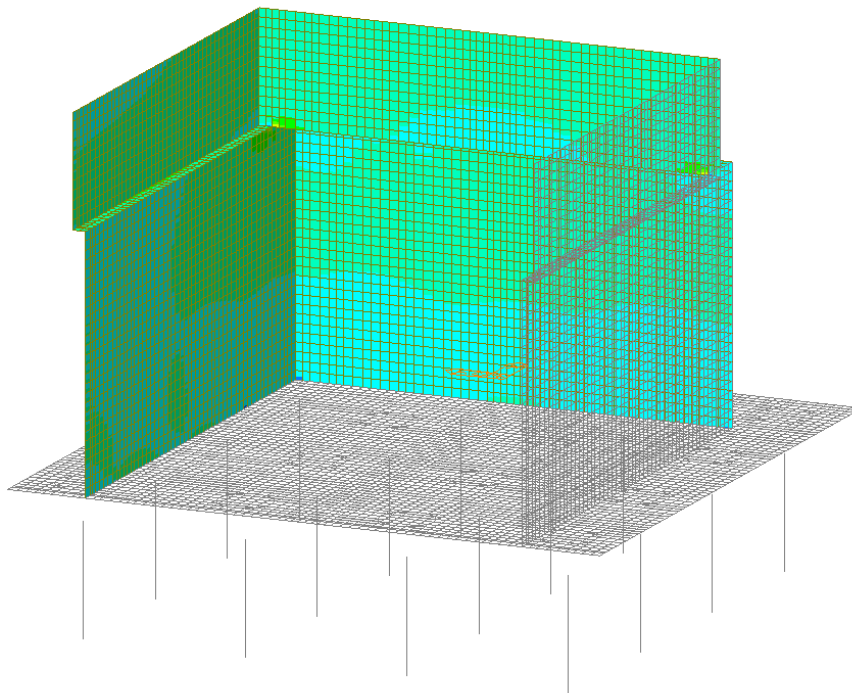
Figura 40 – Involuppo SLE Frequente - Fxx
