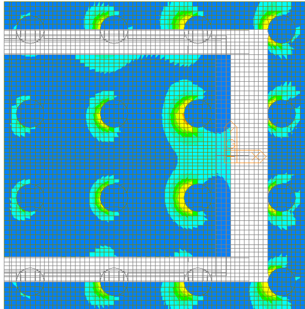
Figura 97 – Inviluppo SLU – W-A Moment Top Direzione 1
