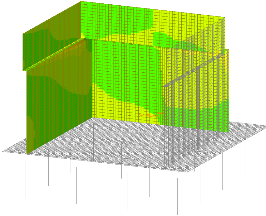
Figura 37 – Involuppo SLE Rara - Vxx
