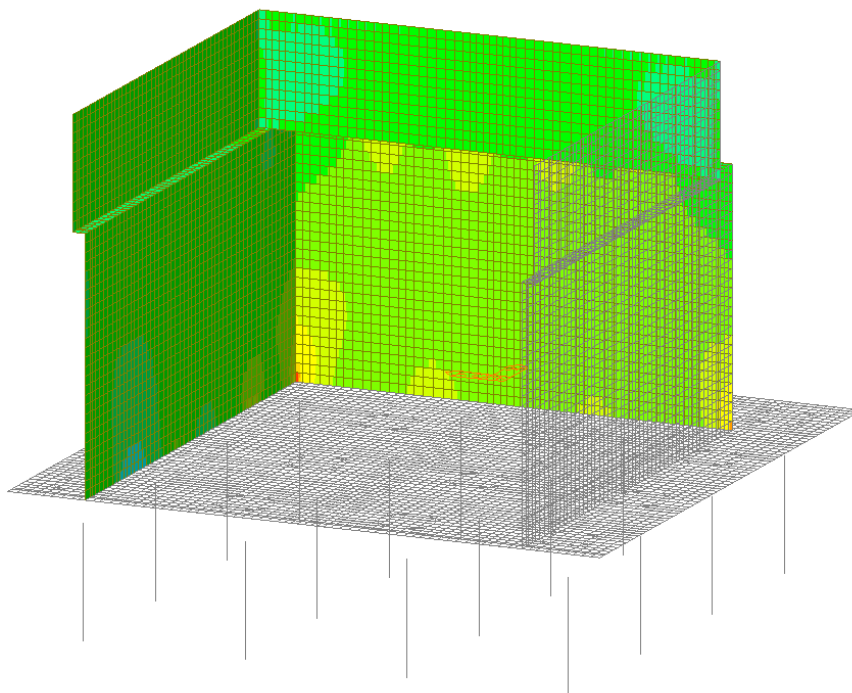
Figura 36 – Involuppo SLE Rara - Fyy
