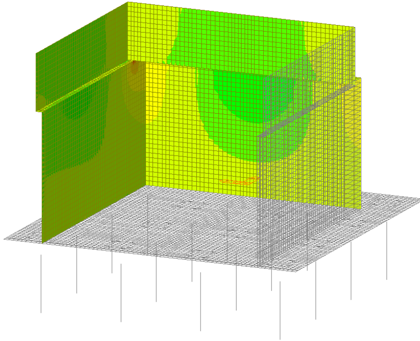
Figura 39 – Involuppo SLE Frequente - Mxx
