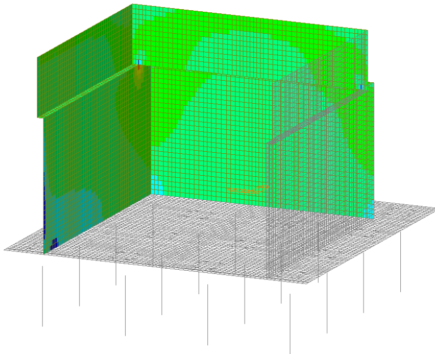
Figura 44 – Involuppo SLE Frequente - V yy
