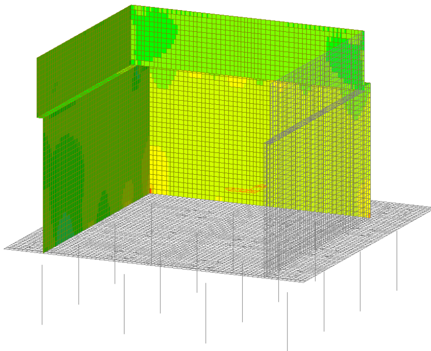
Figura 30 – Involuppo SLU - Fyy
