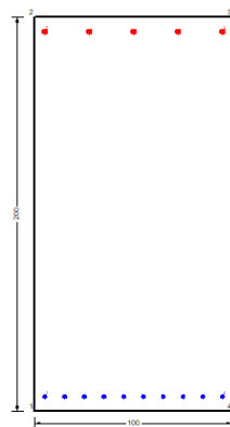
Figura 59 – Sezione implementata in RC-SEC
