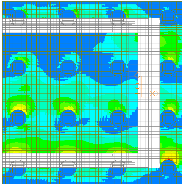
Figura 100 – Inviluppo SLU – W-A Moment Bottom Direzione 2
