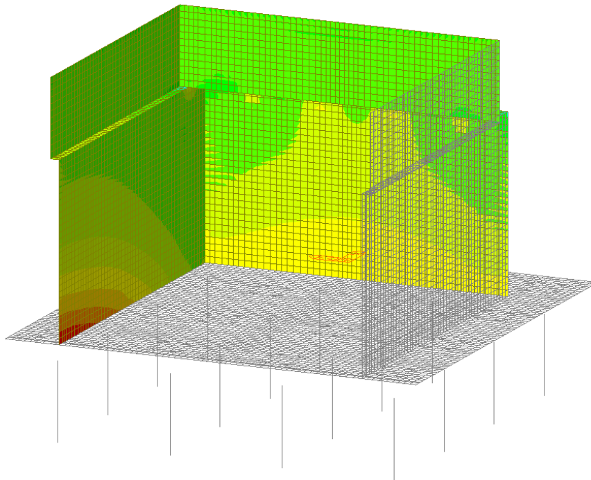
Figura 29 – Involuppo SLU - Myy
