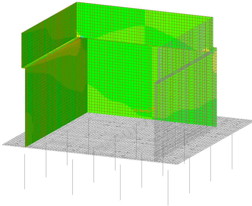
Figura 49 – Involuppo SLE Quasi Permanente - V xx
