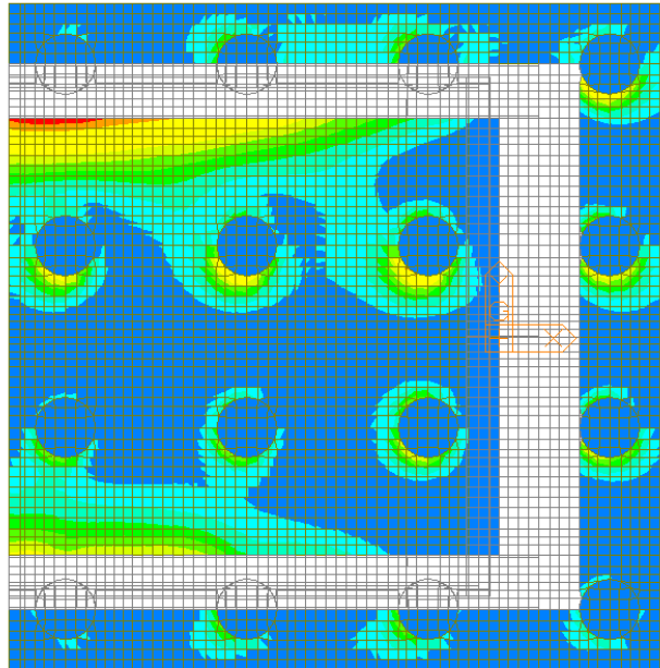
Figura 99 – Inviluppo SLU – W-A Moment Top Direzione 2
