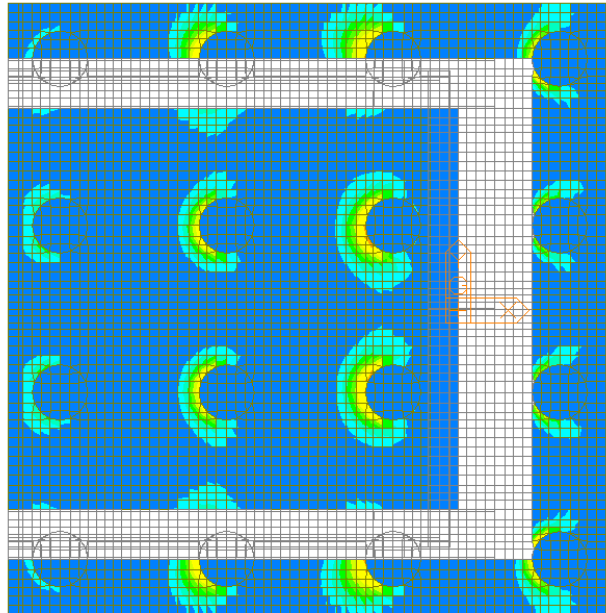
Figura 105 – Involuppo SLE Frequente – W-A Moment Top Direzione 1
