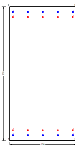
Figura 113 – Sezione implementata in RC-SEC
