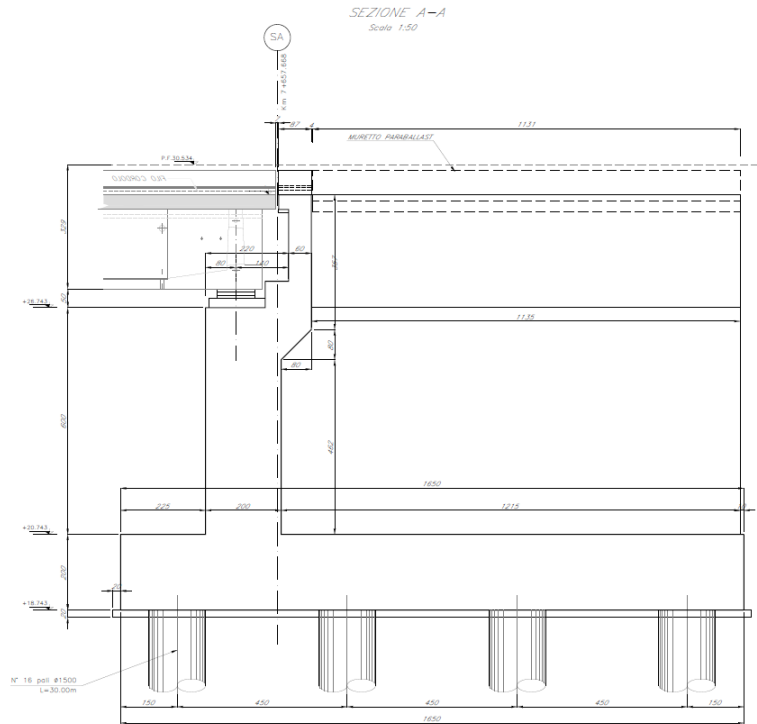
Figura 4 – Sezione longitudinale Spalla B
