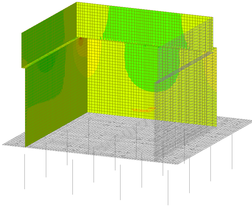
Figura 45 – Involuppo SLE Quasi Permanente - Mxx
