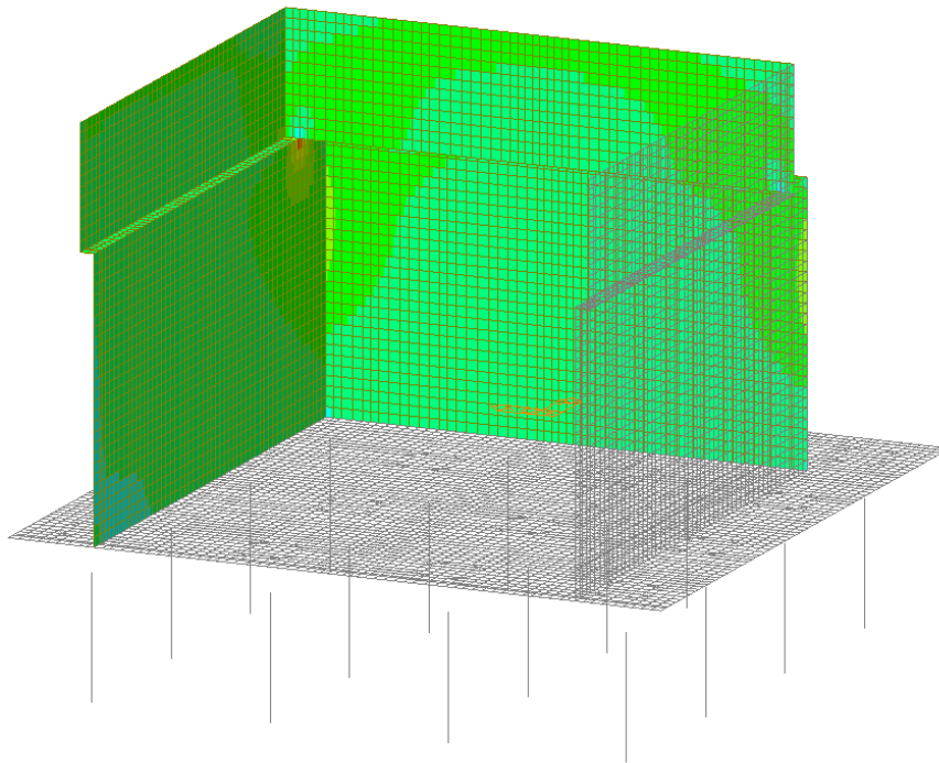
Figura 38 – Involuppo SLE Rara - Vyy
