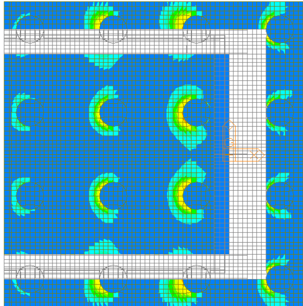
Figura 101 – Involuppo SLE Rara – W-A Moment Top Direzione 1
