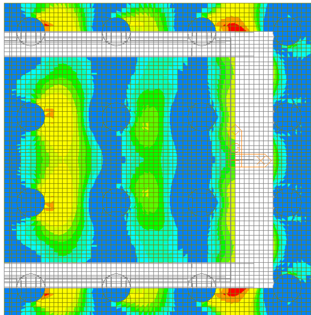
Figura 110 – Inviluppo SLE Quasi Permanente – W-A Moment Bottom Direzione 1
