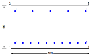
Figura 92 – Sezione implementata in RC-SEC
