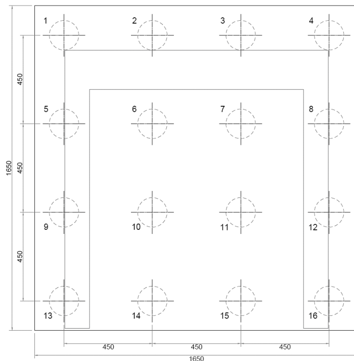
Figura 118 – Disposizione e numerazione dei pali di fondazione
