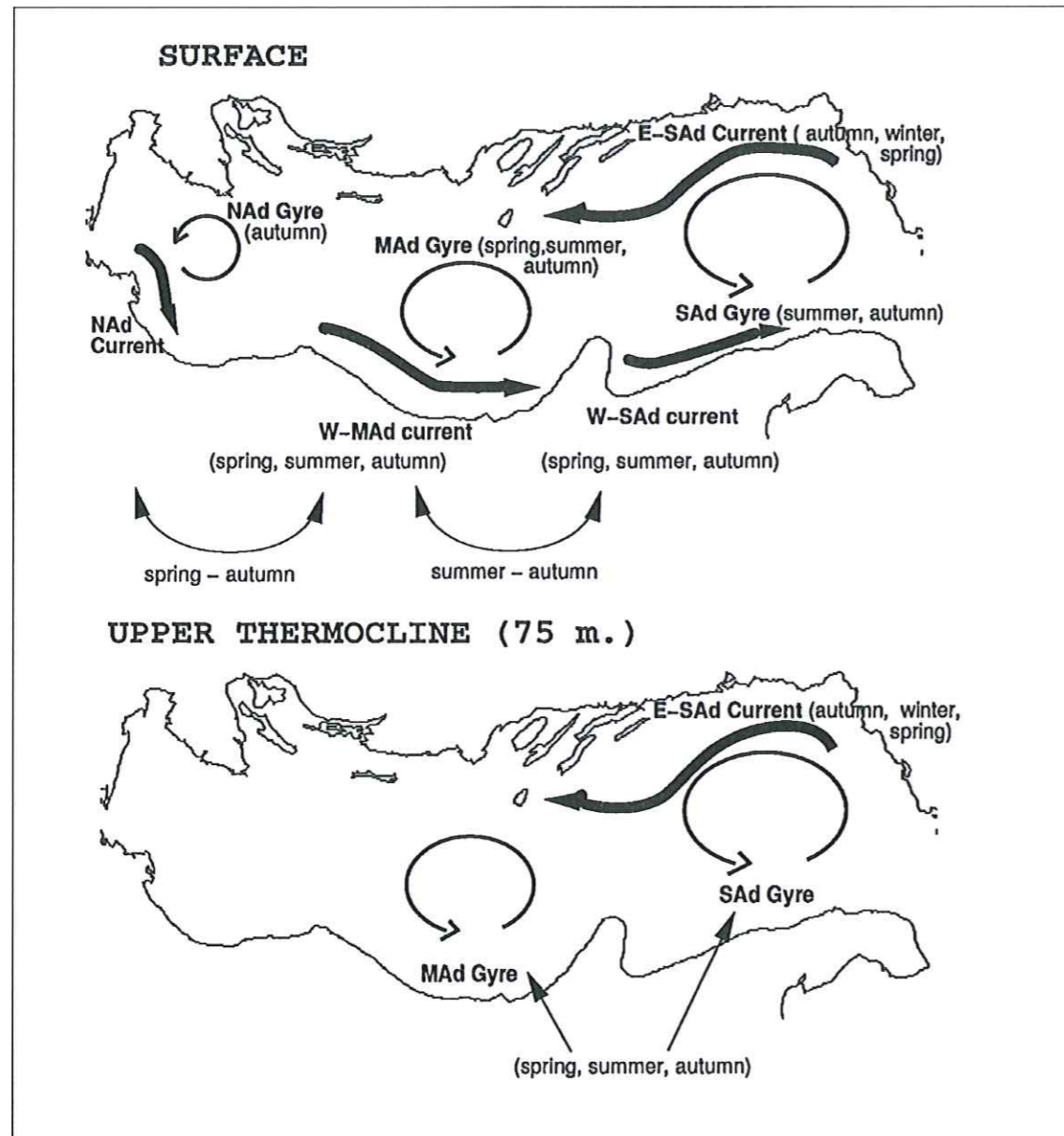
CIRCOLAZIONE GENERALE DEL MARE ADRIATICO
