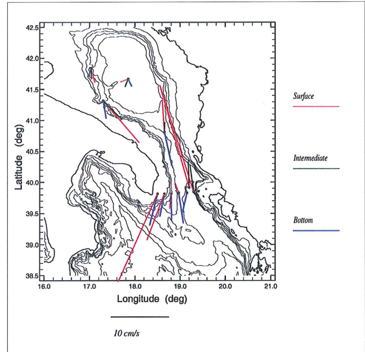
CIRCOLAZIONE DI DETTAGLIO DEL BASSO ADRIATICO
