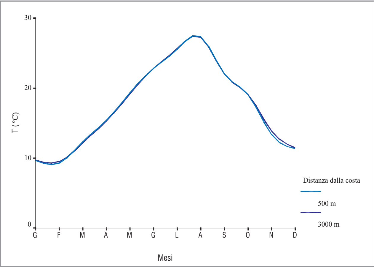
TEMPERATURA: ANDAMENTO MEDIA MENSILE RILEVATA A 500 m E 3,000 m DALLA COSTA ADRIATICA
