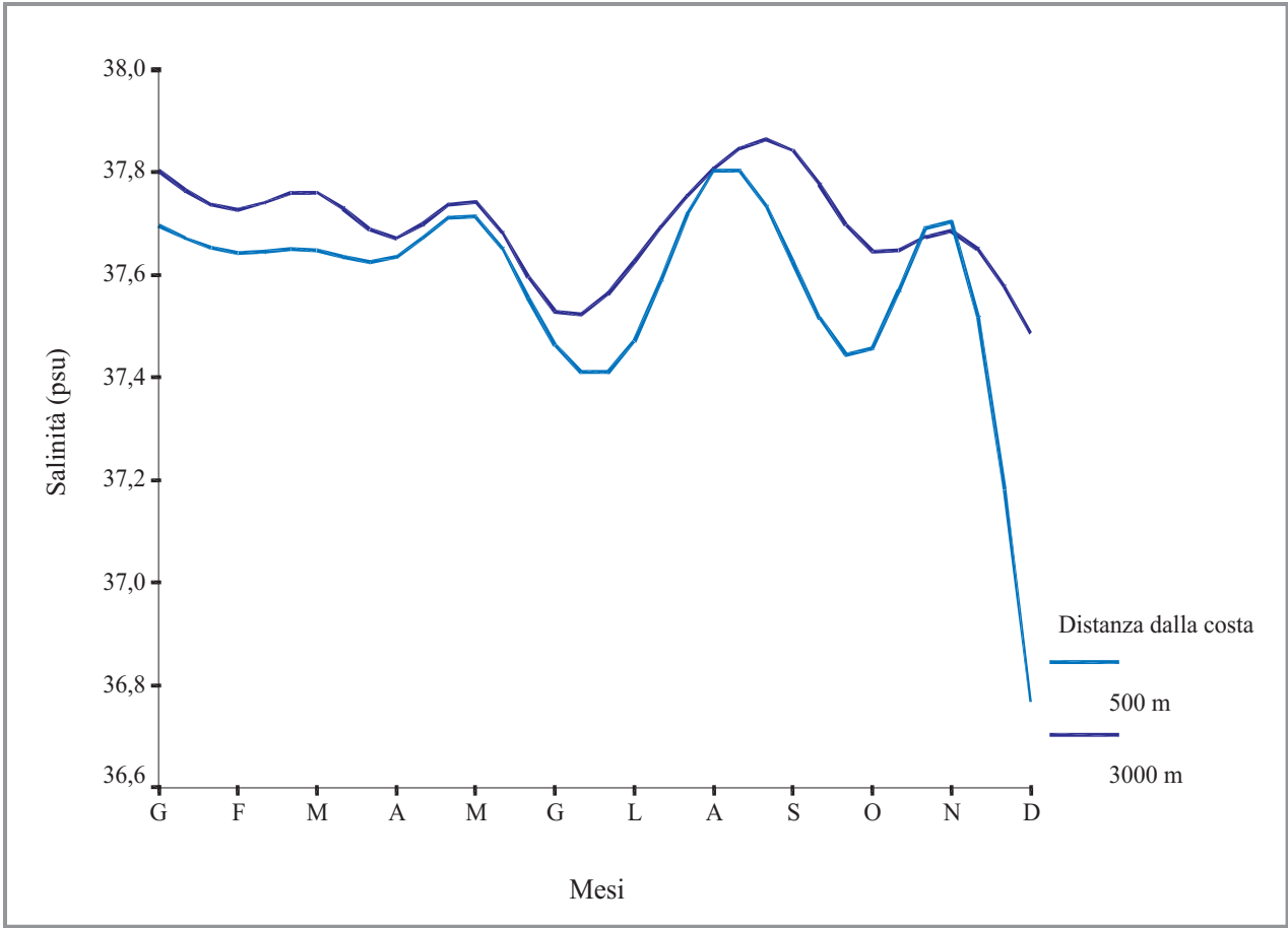
SALINITÀ: ANDAMENTO MEDIA MENSILE RILEVATA A 500 m E 3,000 m DALLA COSTA ADRIATICA
