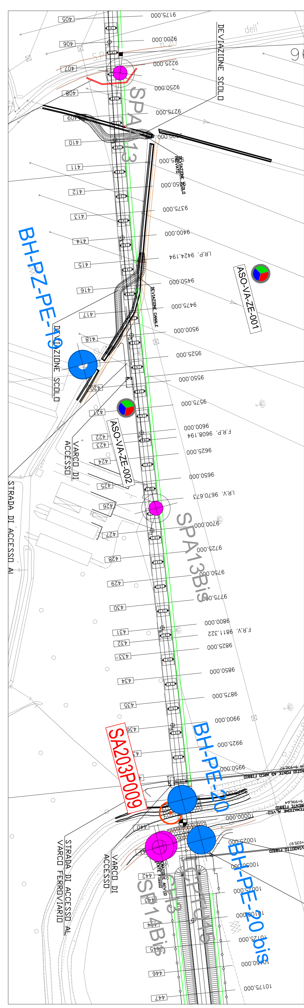
PLANIMETRIA Scala 1:2000
