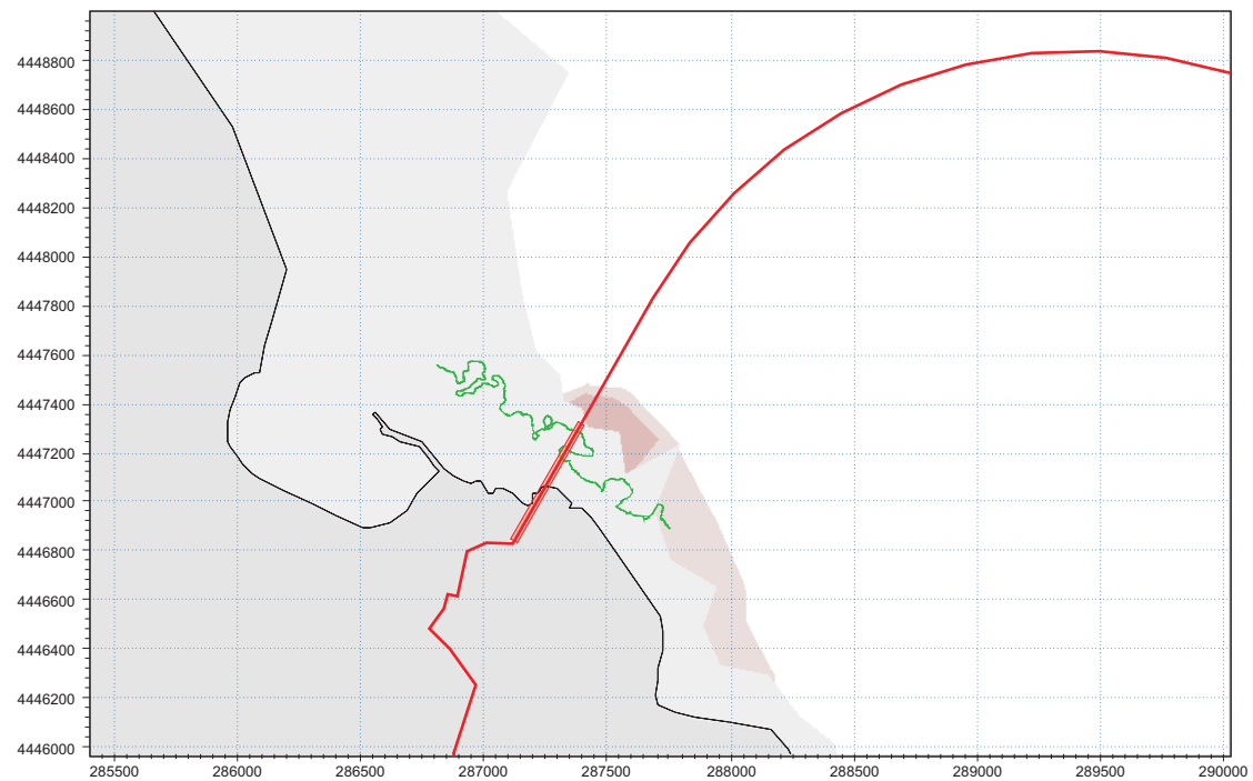
d) Sezione orizzontale z = -30 m
