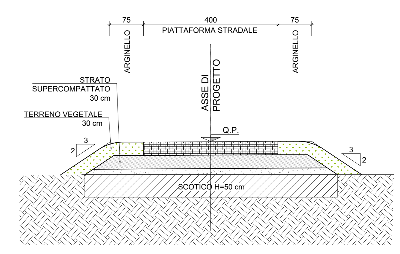
SEZIONE TIPO - STRADA PODERALE 4.00m
