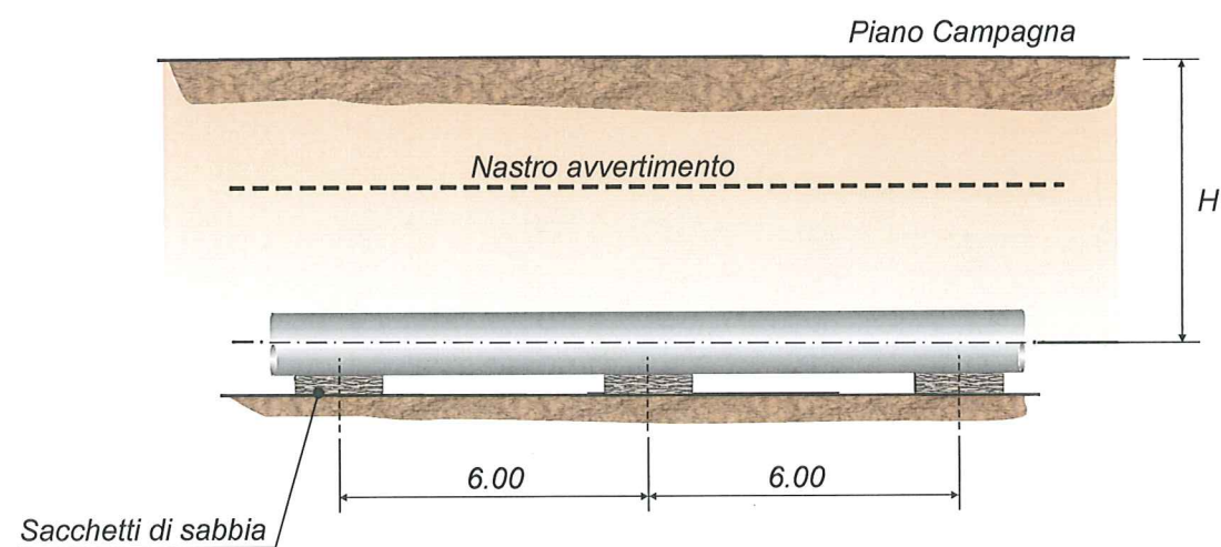
SEZIONE "A-A"
