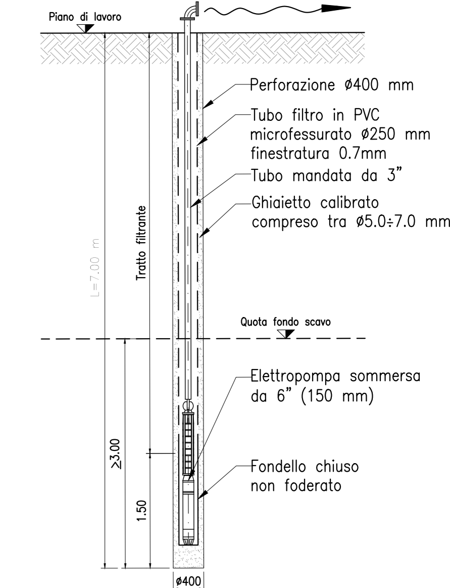
SEZIONE TIPO POZZO PER AGGOTTAMENTO Scala 1:50
