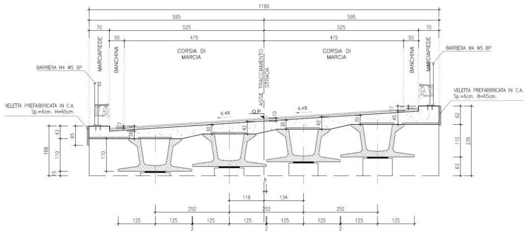
Figura 3 Sezione trasversale d'impalcato
