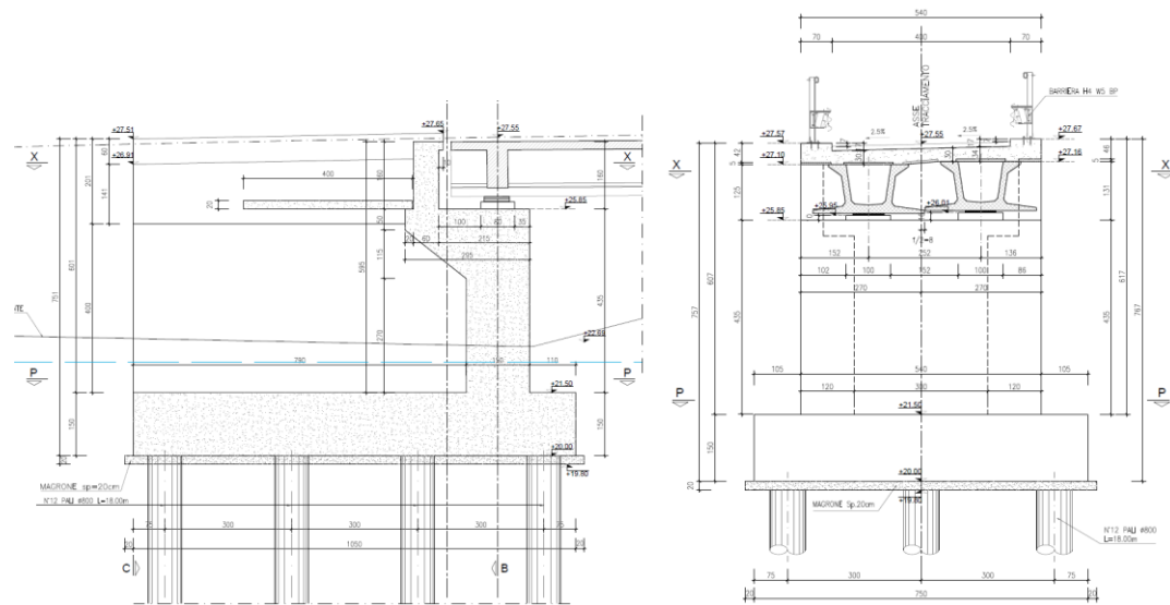
Figura 9: Carpenteria spalle
