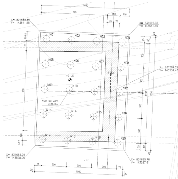
Figura 4: Pianta fondazioni
