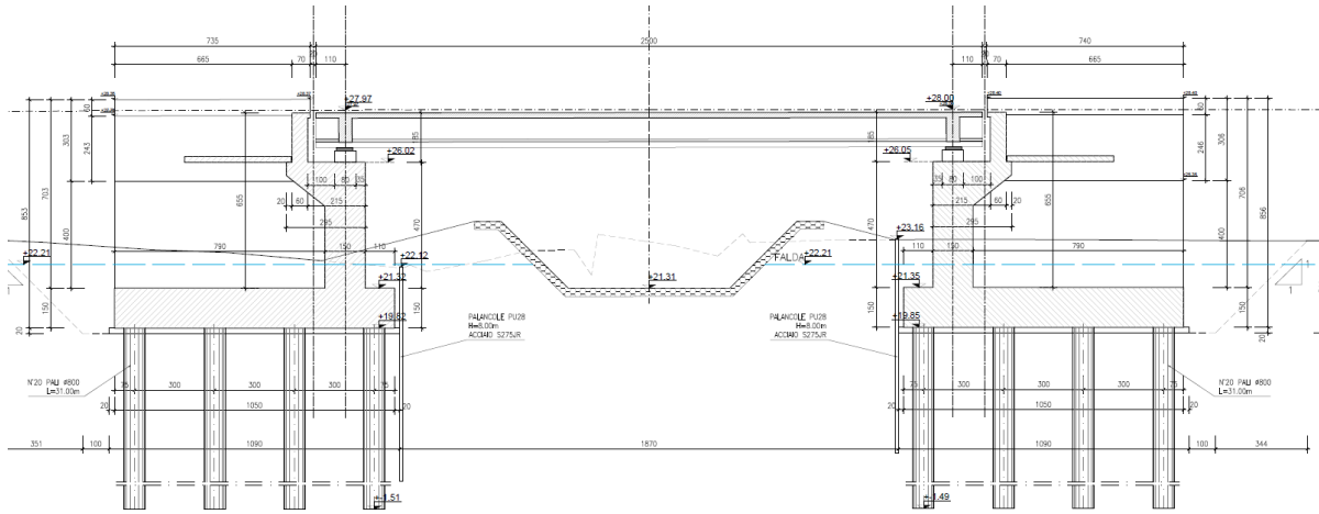
Figura 2 Profilo dell'opera
