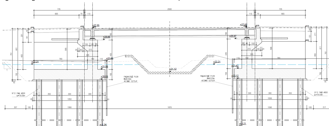
Figura 6 Profilo dell'opera
