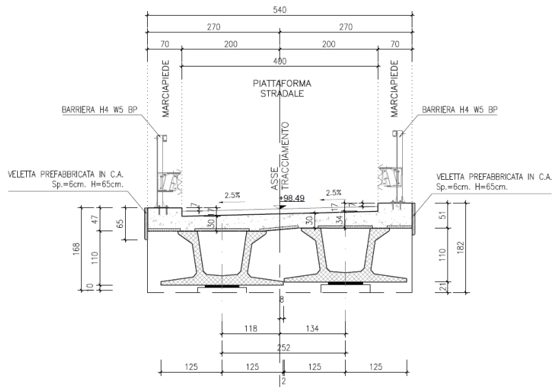
Figura 7 Sezione trasversale d'impalcato
