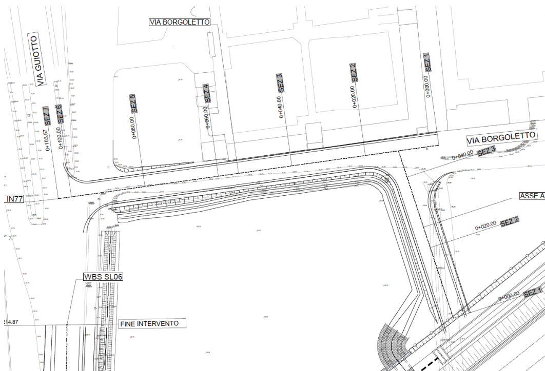
Figura 1: Stato di progetto
