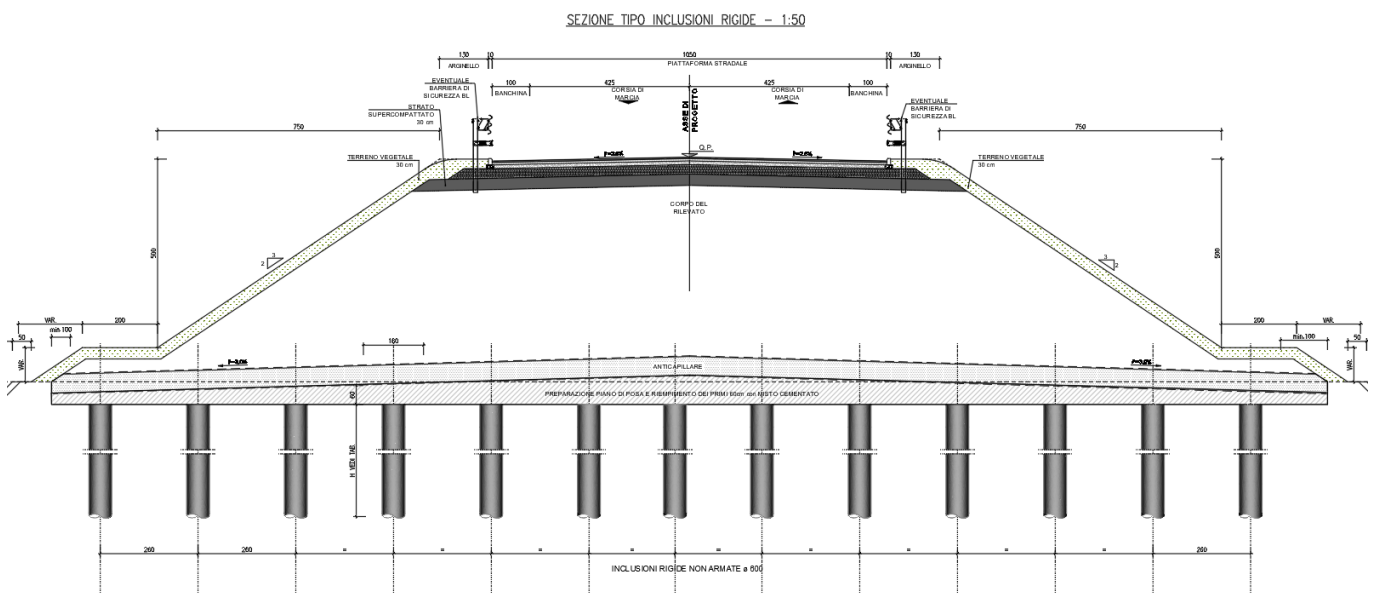
Figura 2: Inclusioni rigide
