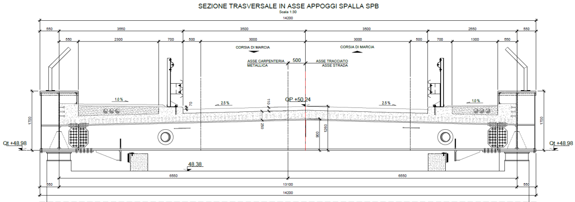
Figura 2: Sezione trasversale
