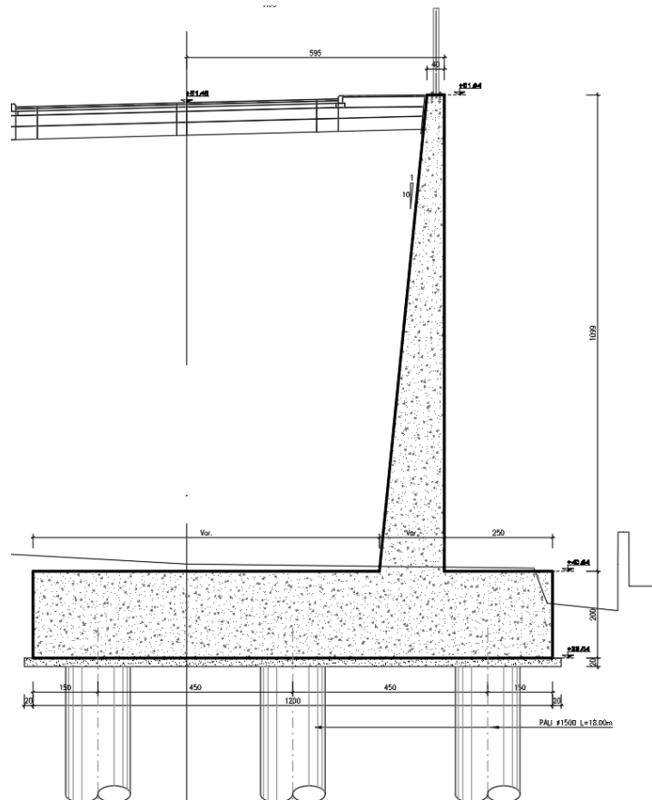
Figura 5: Sezione trasversale muro lato spalla A in dx
