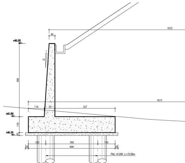
Figura 6: Sezione trasversale muro lato spalla A in sx
