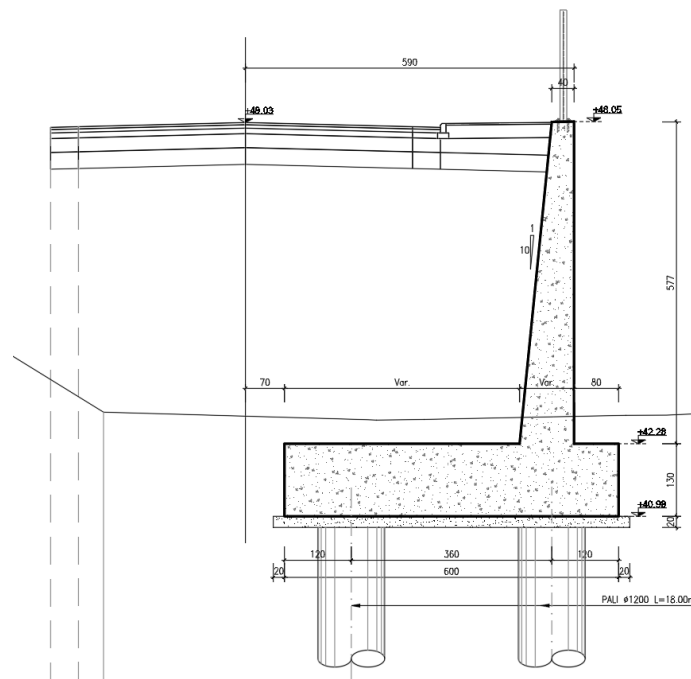
Figura 7: Sezione trasversale muro lato spalla B in dx
