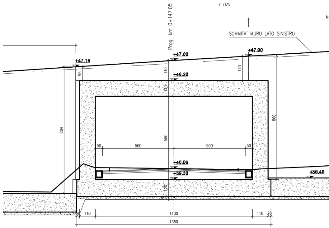
Figura 8: Sezione trasversale scatolare
