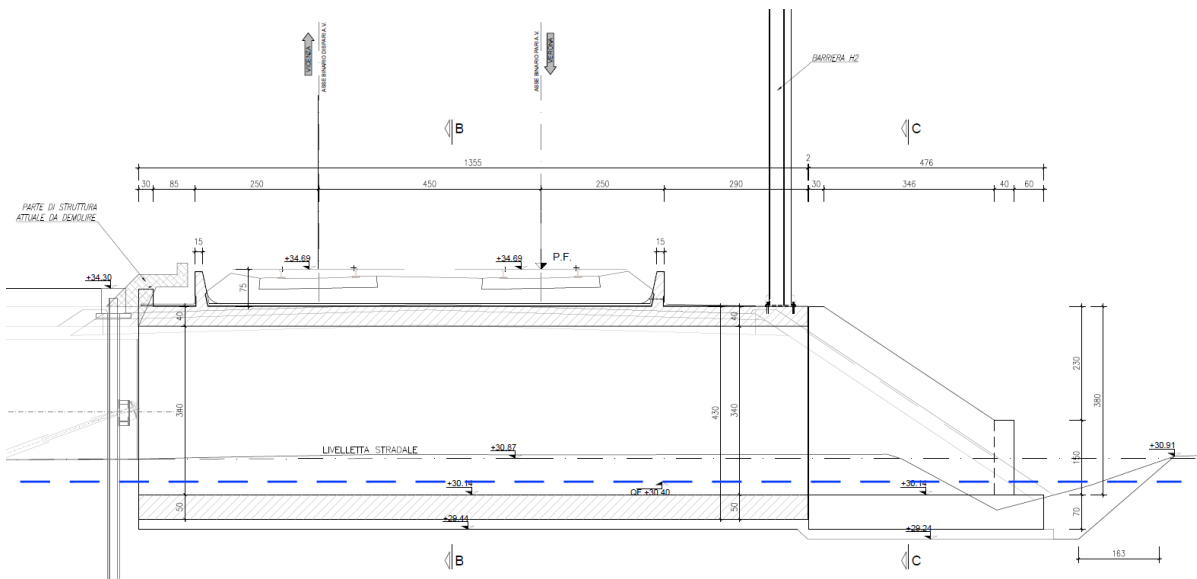
Figura 1.2: Sezione Longitudinale PE
