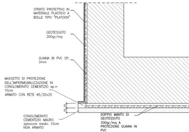
Figura 1.3: Dettaglio impermeabilizzazione
