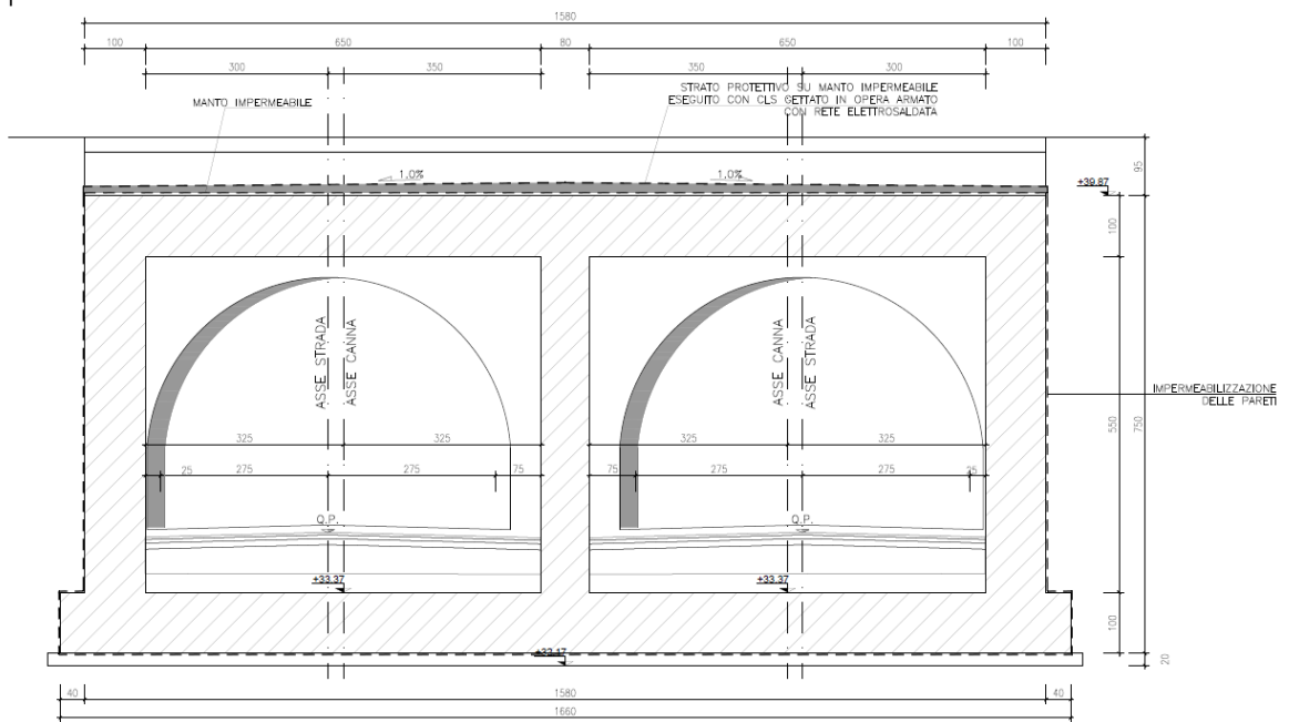
Figura 1.2: Sezione trasversale
