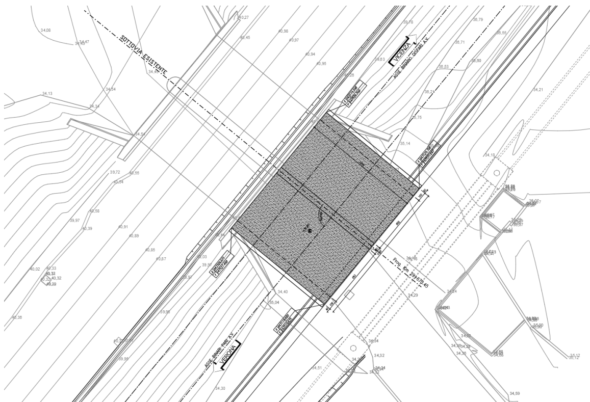
Figura 1.3: Planimetria di progetto
