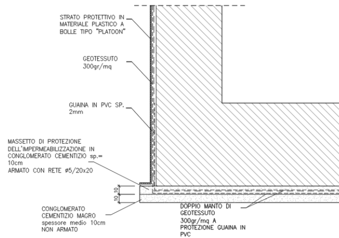
Figura 1.5: Dettaglio impermeabilizzazione
