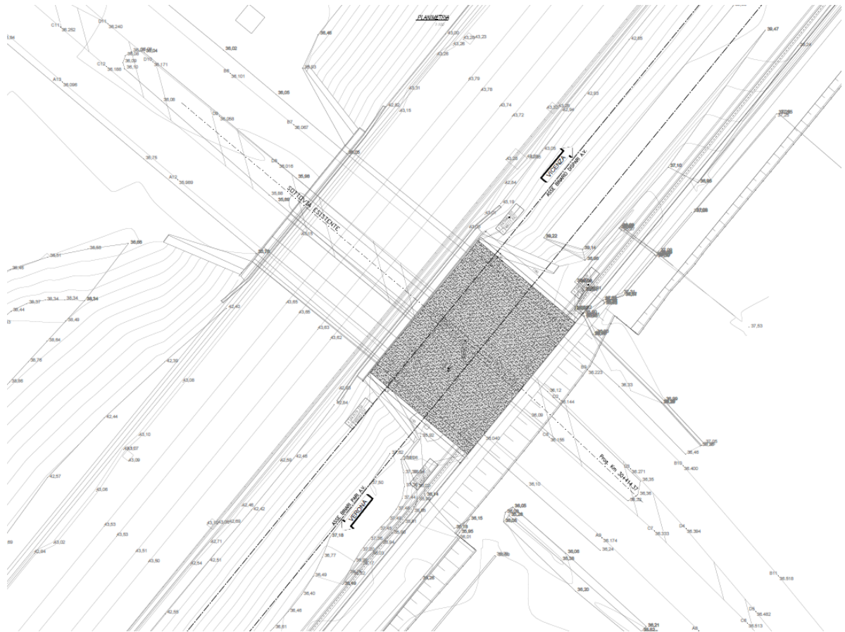
Figura 1.3: Planimetria di progetto
