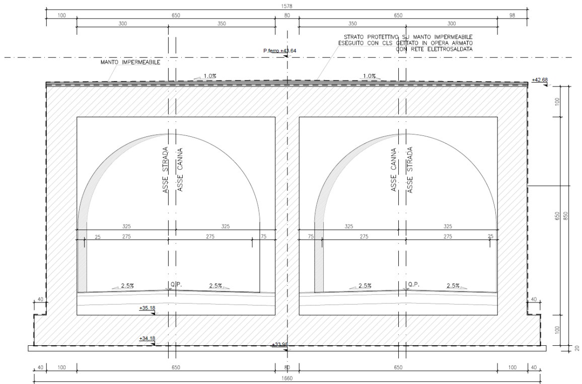
Figura 1.2: Sezione trasversale
