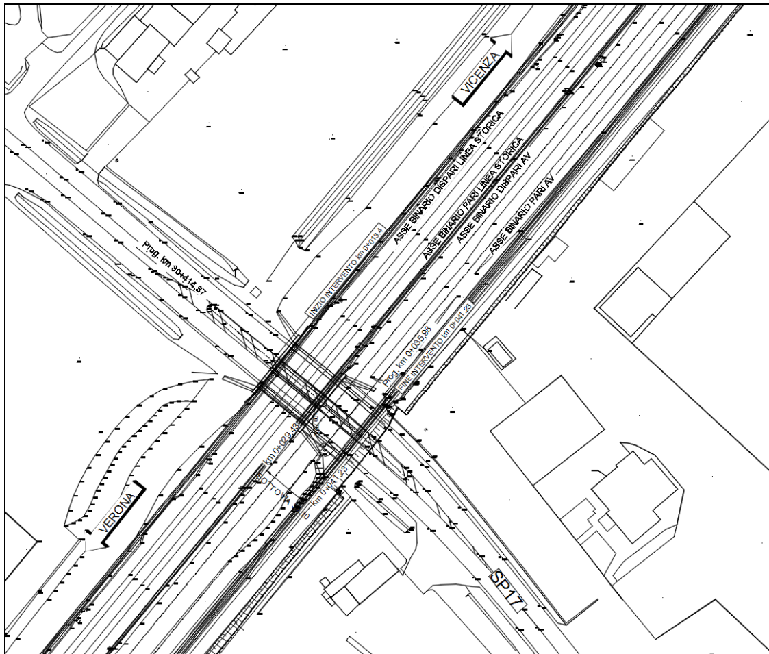
Figura 1: Stato di progetto
