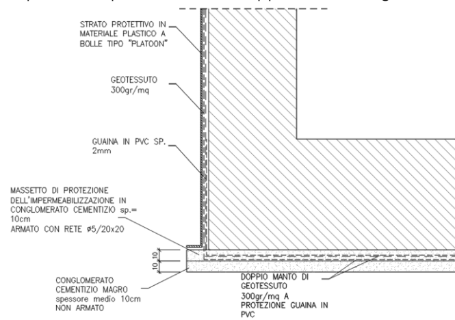
Figura 1.5: Dettaglio impermeabilizzazione
