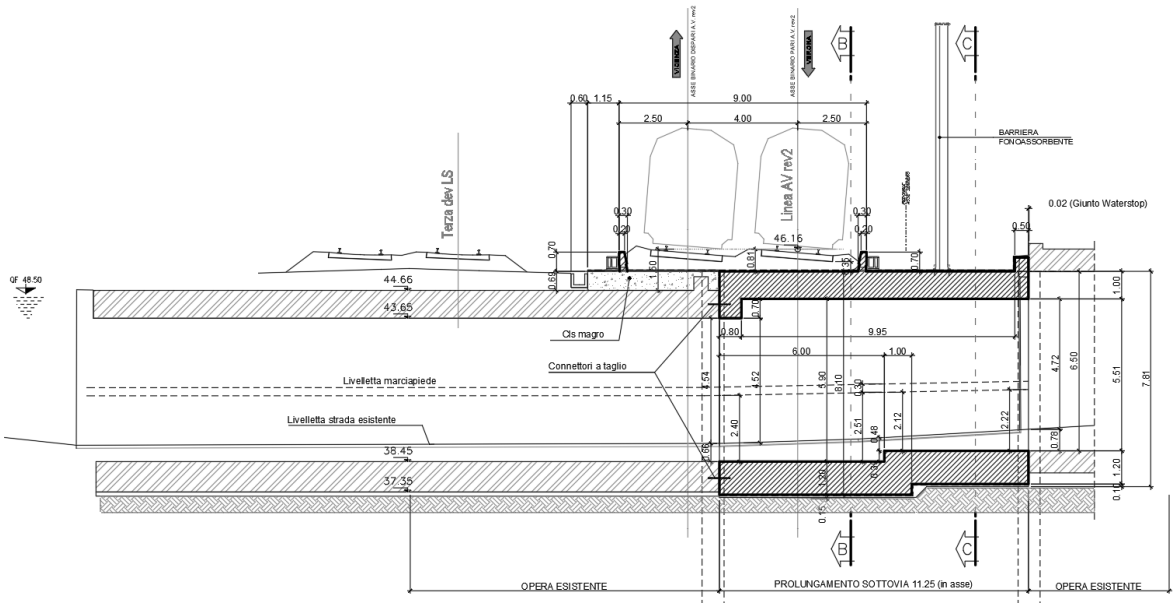
Figura 2: Sezione longitudinale
