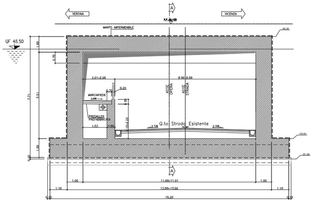
Figura 4: Sezione trasversale lato SP34
