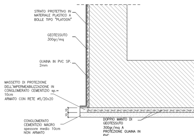
Figura 5: Dettaglio impermeabilizzazione
