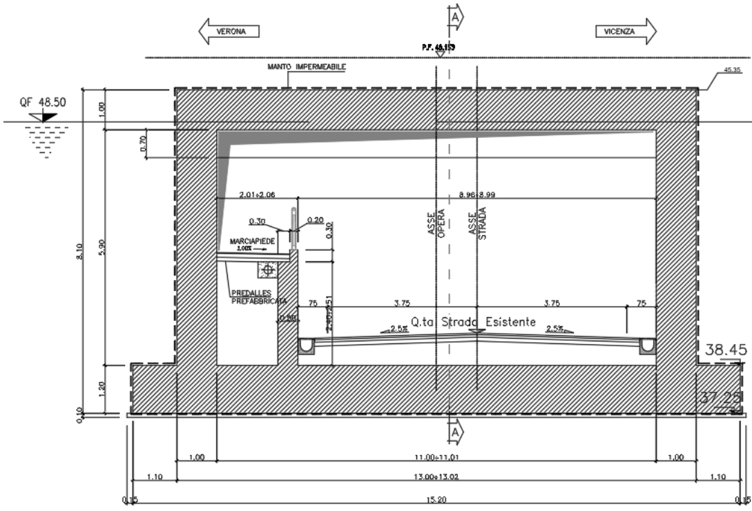
Figura 3: Sezione trasversale lato ferrovia
