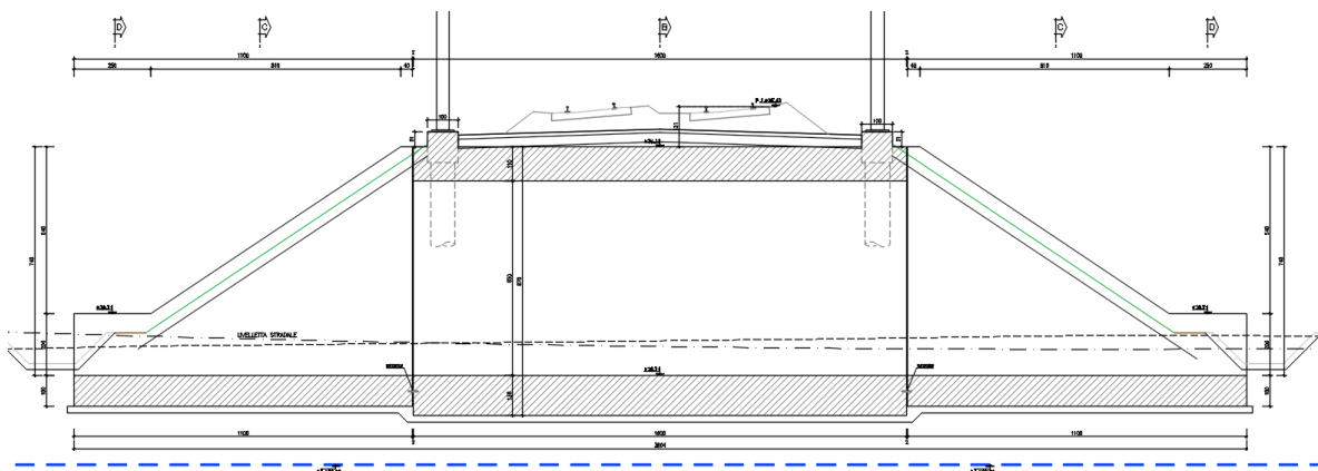
Figura 3: Sezione longitudinale
