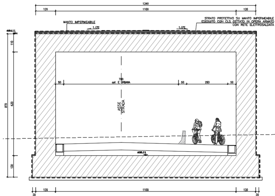
Figura 2: Sezione trasversale in opera
