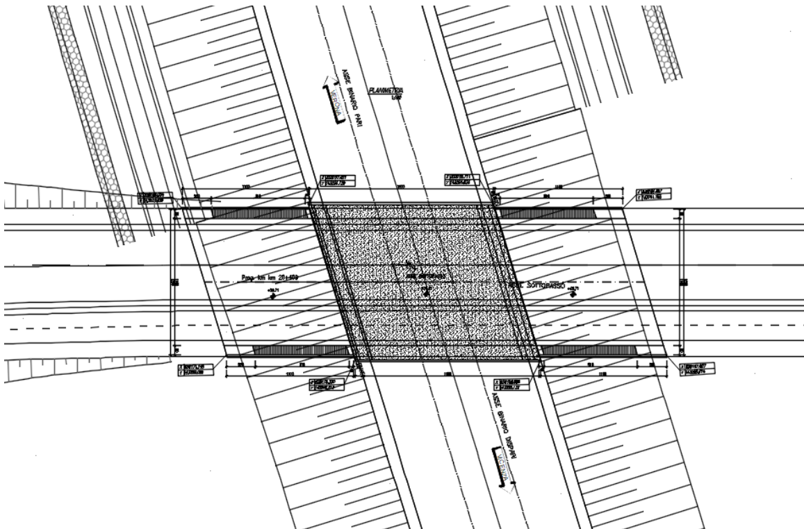
Figura 1: Planimetria di progetto
