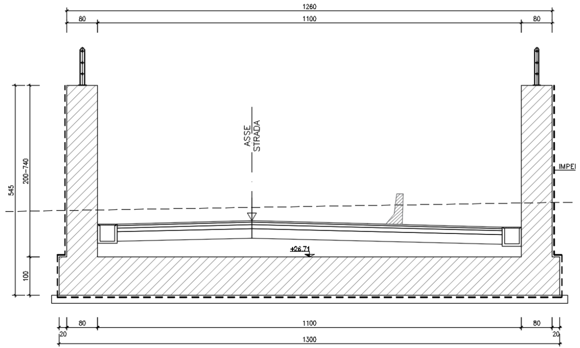
Figura 4: Sezione trasversale muri
